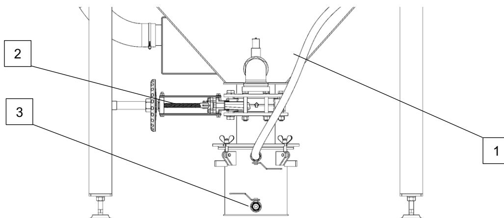
Rysunek 7.3-4 Zbiornik wodny z pojemnikiem na szlam
