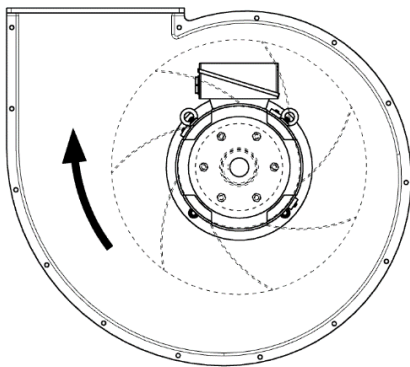
Rysunek 7.3-1 Prawidłowy kierunek obrotu wirnika
