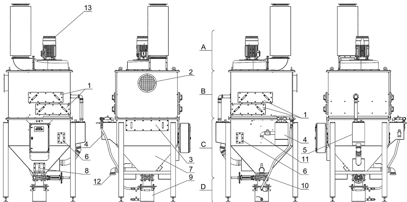
Rysunek 5.3-1 Budowa urządzenia
