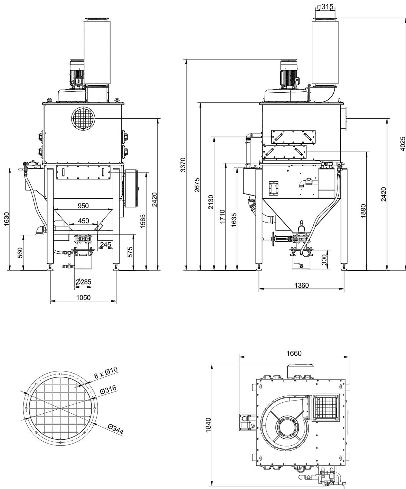
Rysunek 5.4-1 Wymiary urządzenia WET-4000-N
