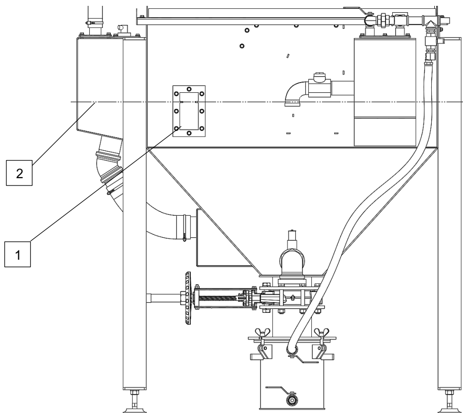
Rysunek 7.3-2 Zbiornik główny z wizjerami
