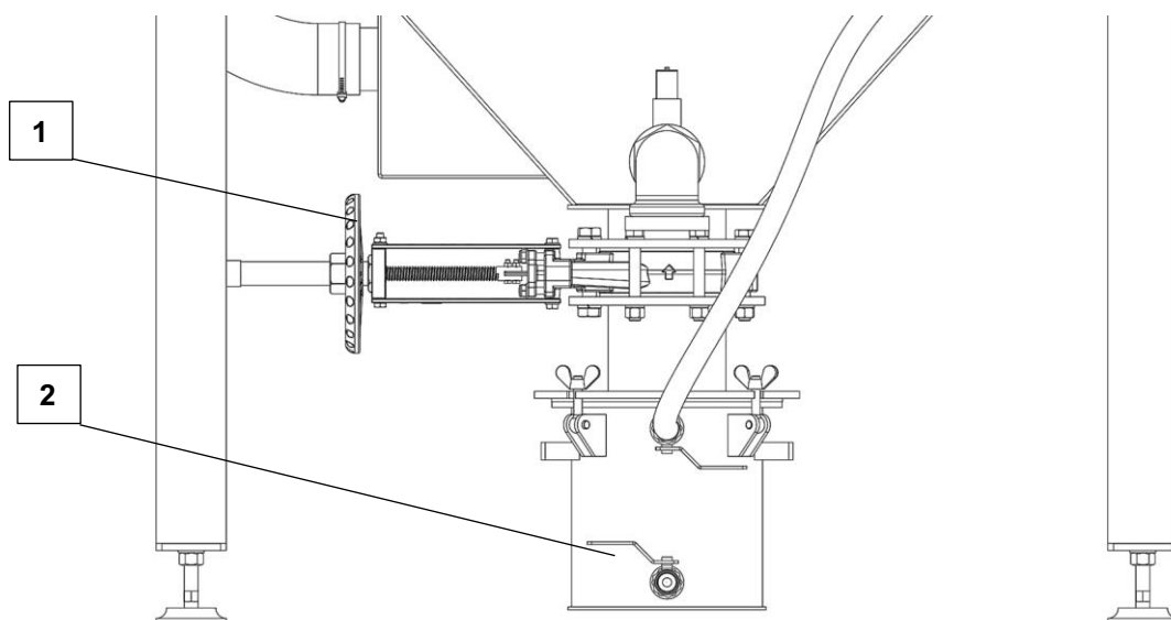
Rysunek 8.2-2 Zbiornik, zasuwa nożowa i pojemnik
