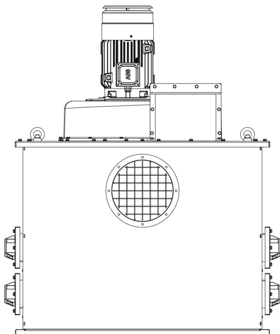
Rysunek 7.1-4 Część górna – Widok 1
