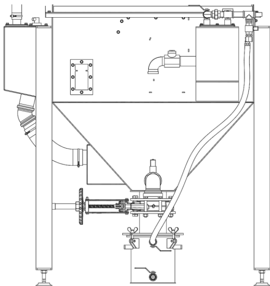
Rysunek 7.1-1 Część dolna – Widok 1
