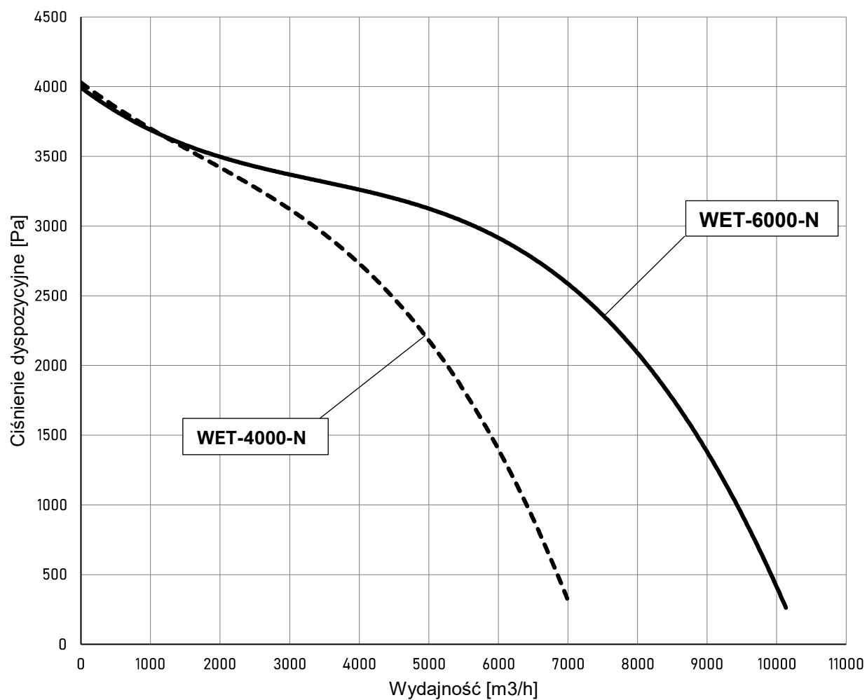
Wykres 1 Charakterystyka przepływowa urządzenia WET-4000-N i WET-6000-N
