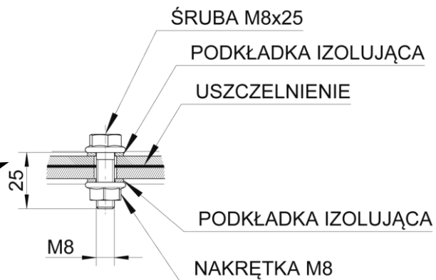
Rysunek 7.1-7 Połączenie śrubowe
