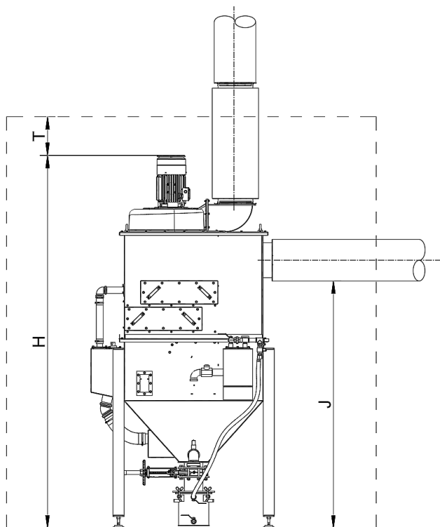
Rysunek 7.2-1 Przestrzeń robocza – Rzut boczny
