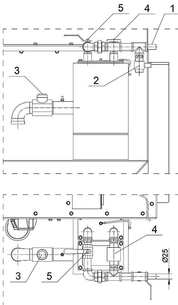
Rysunek 5.3-2 Kolektor zaworów
