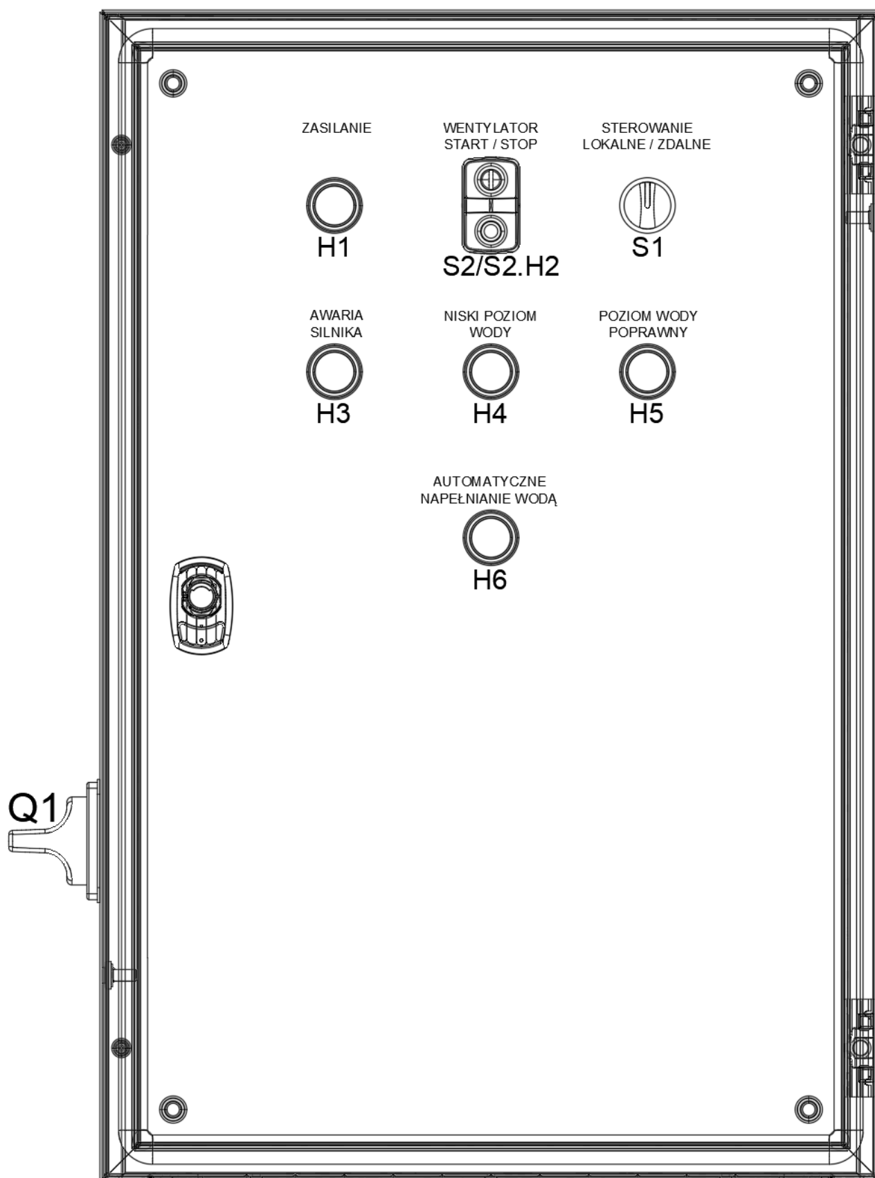
Rysunek 13.2-1 Panel przedni rozdzielnic
