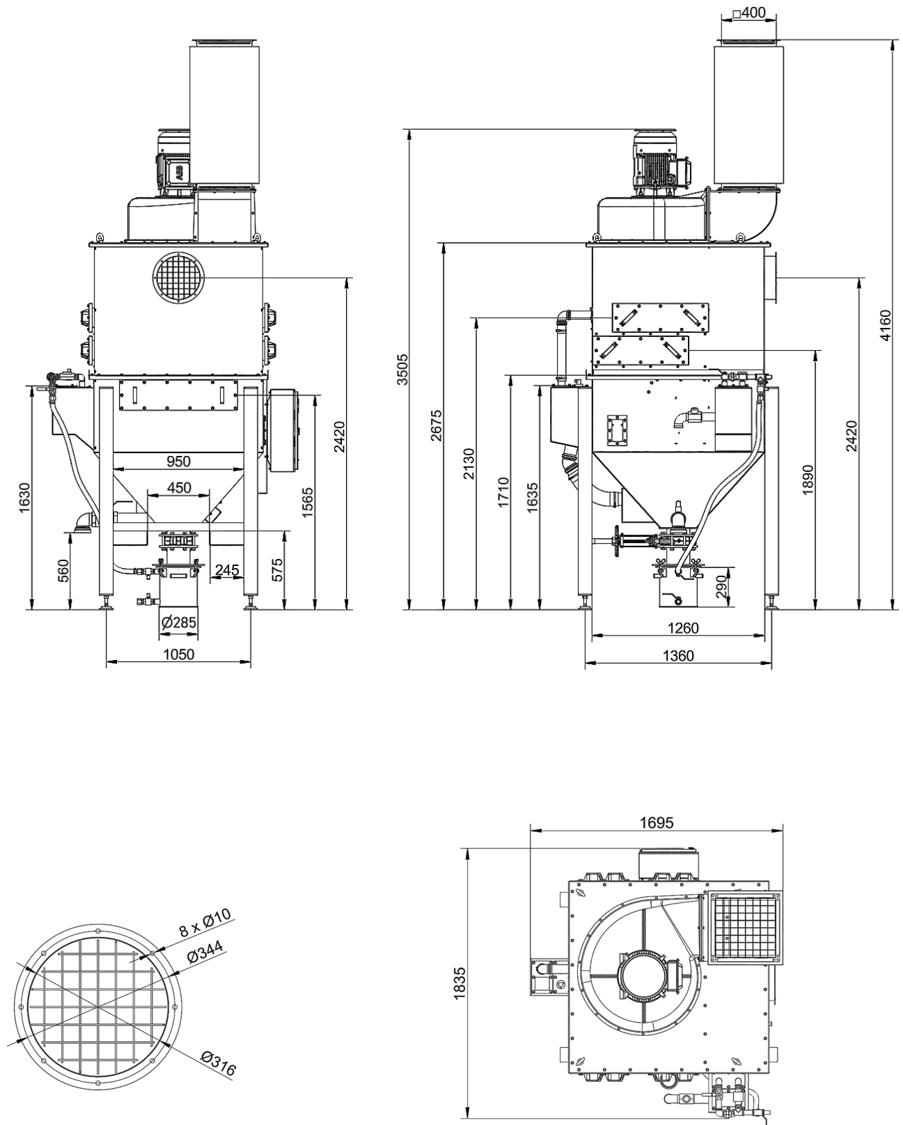
Rysunek 5.4-2 Wymiary urządzenia WET-6000-N
