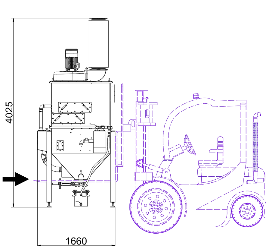
Rysunek 6.1-1 Transport urządzenia na wózku widłowym
