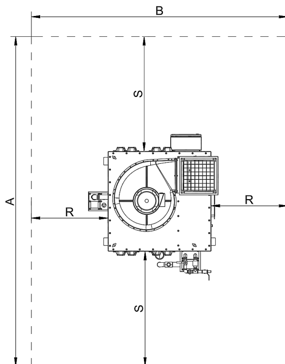
Rysunek 7.2-2 Przestrzeń robocza – Rzut góry
