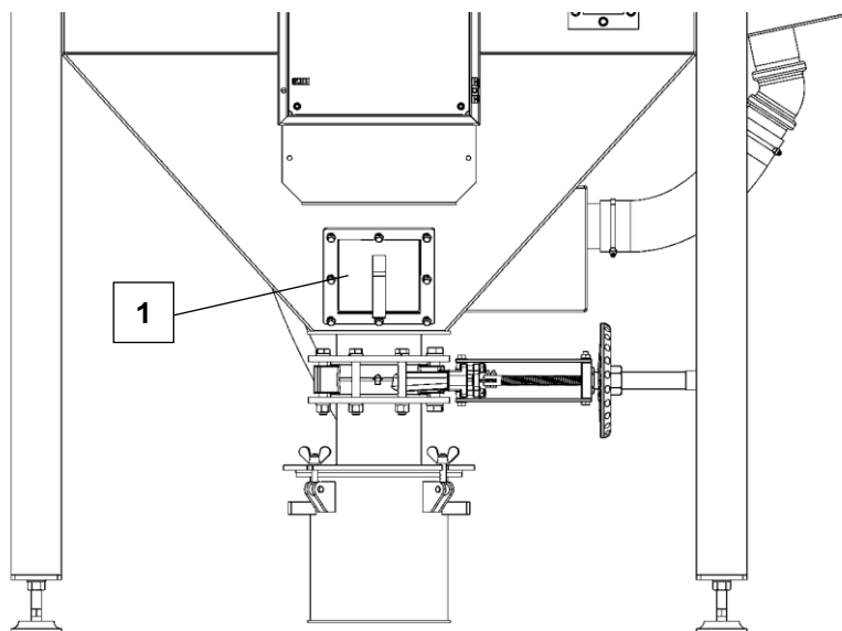
Rysunek 9.2-1 Rewizja zbiornika głównego
