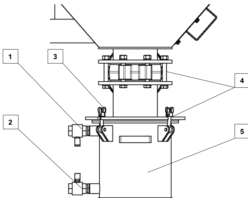
Rysunek 8.2-3 Pojemnik na szlam
