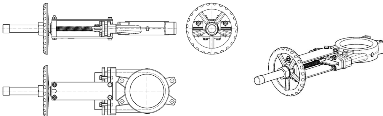
Rysunek 7.3-3 Zasuwa nożowa
