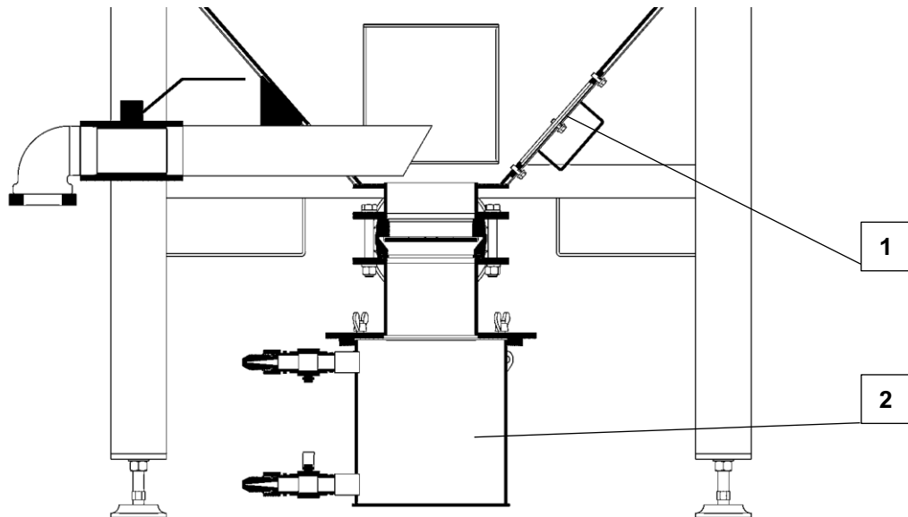
Rysunek 9.2-2 Przekrój zbiornika głównego
