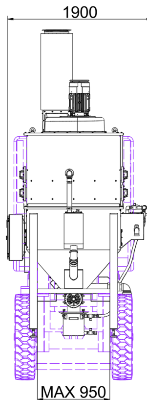
Rysunek 6.1-2 Rozstaw wideł wózka
