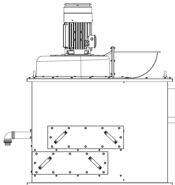
Rysunek 7.1-5 Część górna – Widok 2
