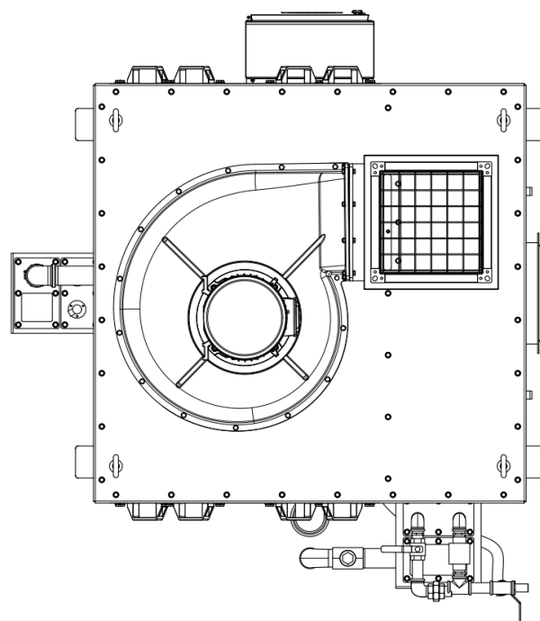
Rysunek 7.1-5 Część górna – Widok 2
