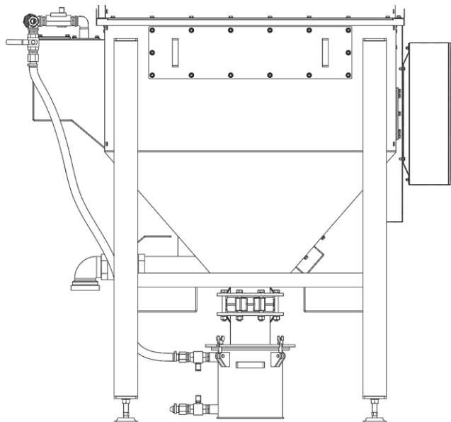
Rysunek 7.1-2 Część dolna – Widok 2
