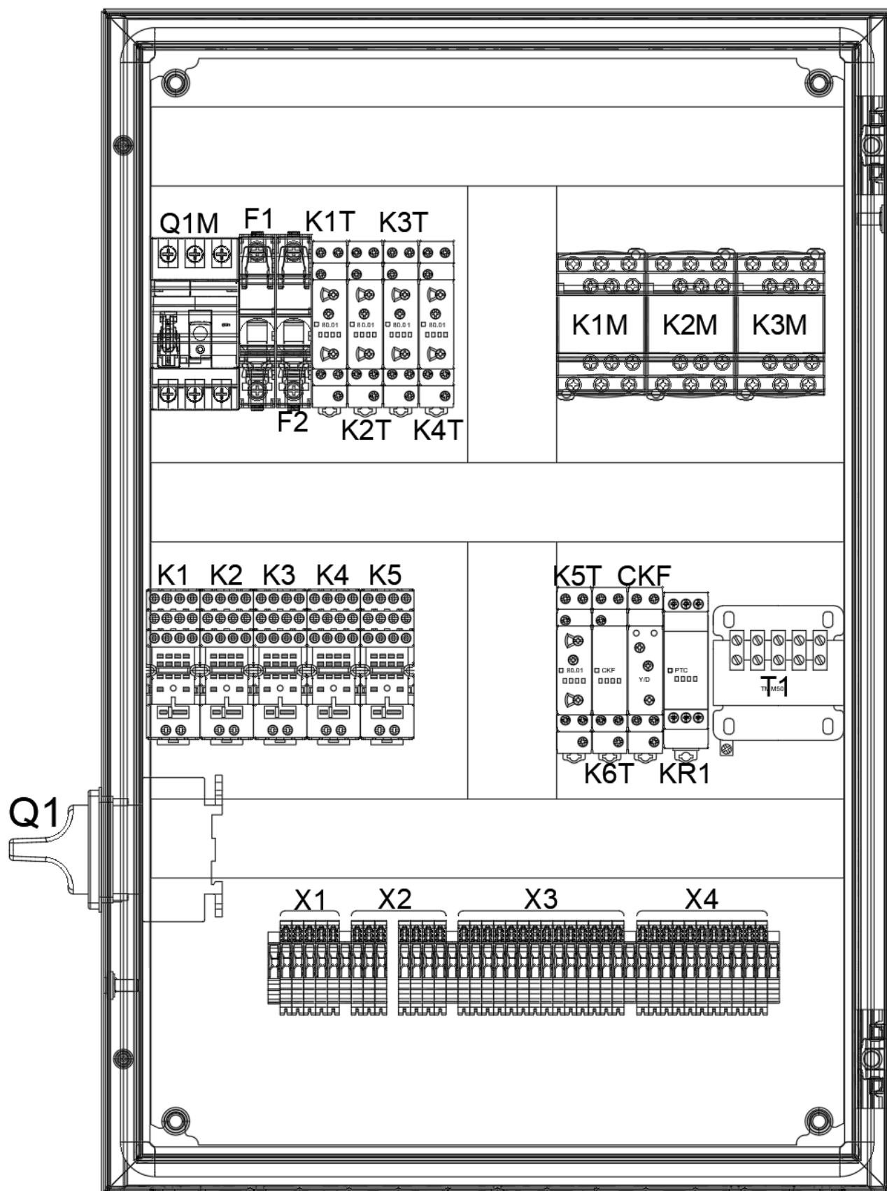
Rysunek 13.2-3 Wnętrze rozdzielnic
