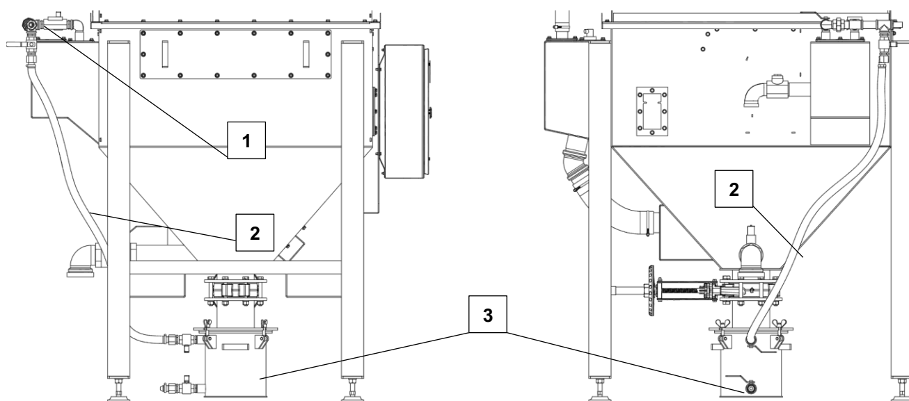
Rysunek 8.2-1 Połączenie sieci wodociągowej z pojemnikiem na szlam
