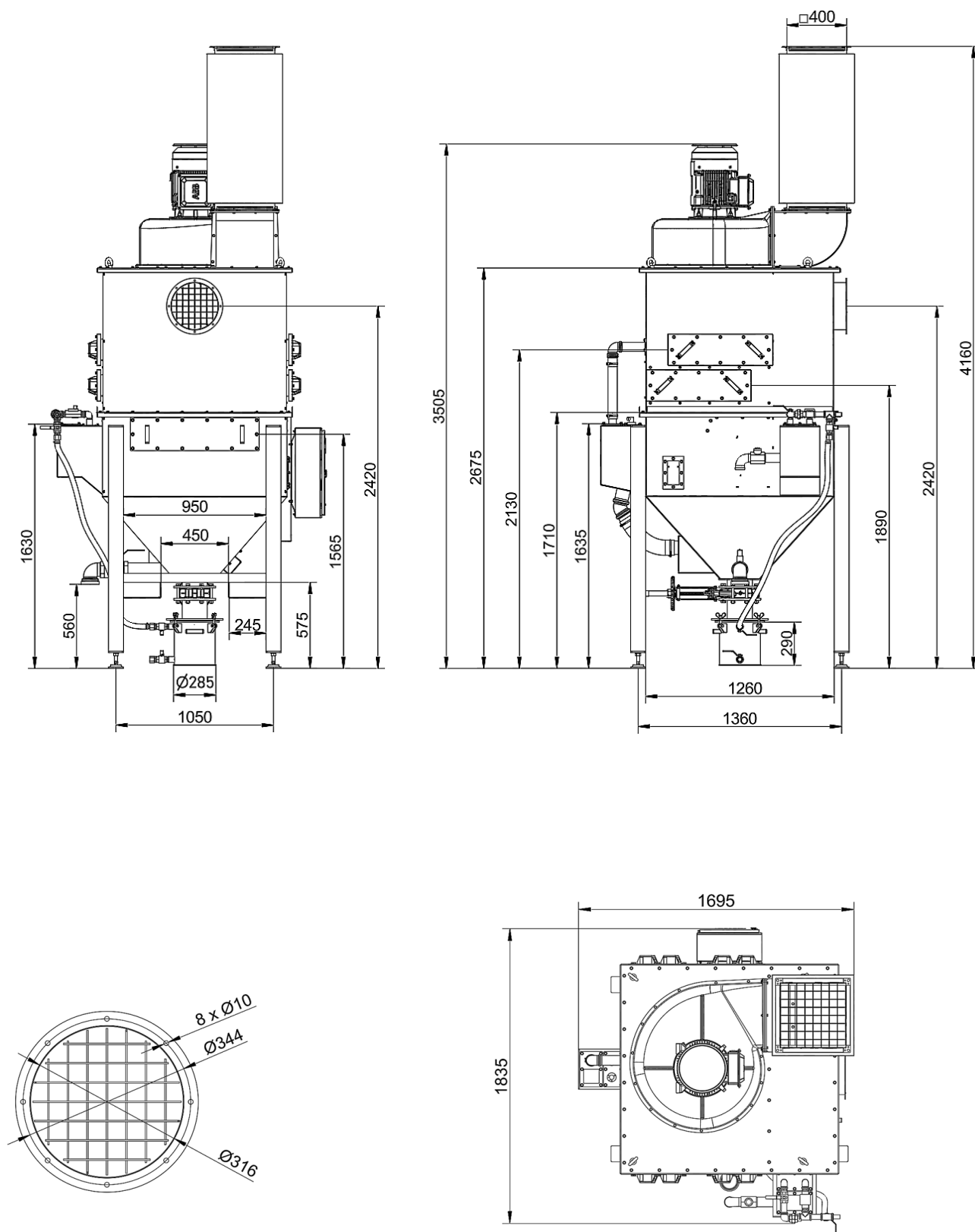
Rysunek 5.4-2 Wymiary urządzenia WET-6000-N
