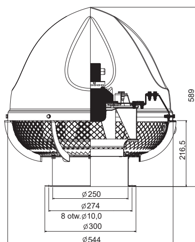
Wentylator dachowy SMART-EC-3000
