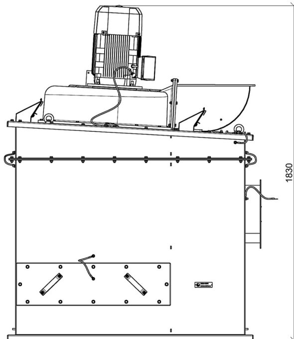
Rysunek 14 Część górna – Widok 2
