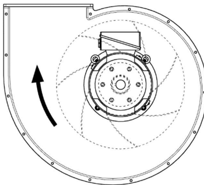
Rysunek 20 Prawidłowy kierunek obrotu wirnika
