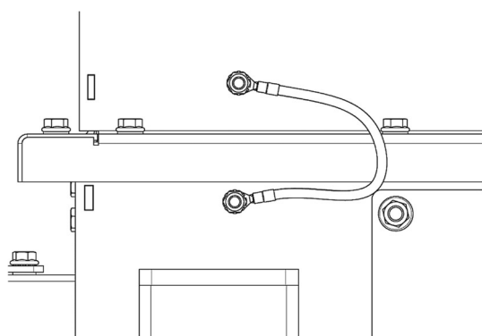
Rysunek 17 Przykład połączenia wyrównawczego
