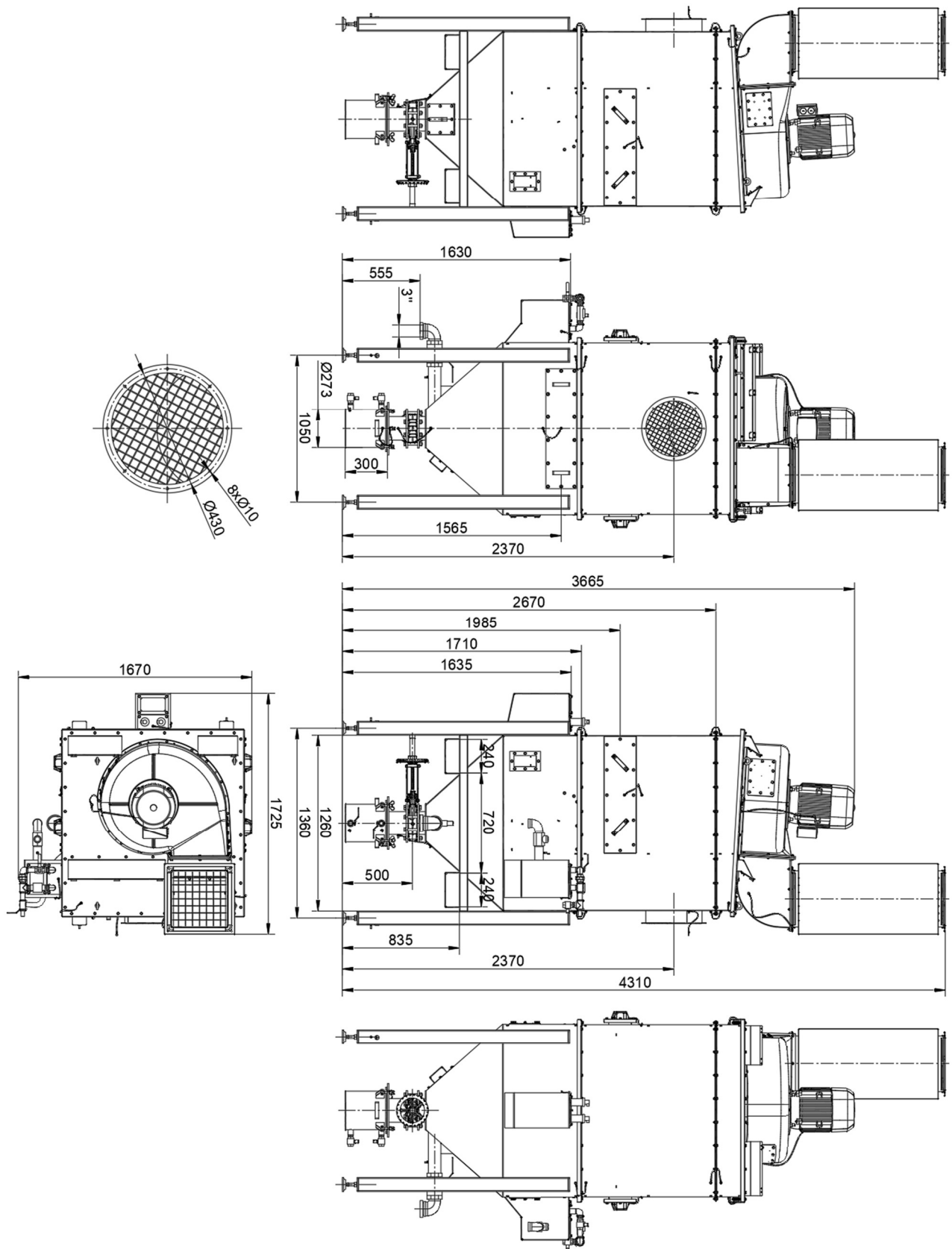
Rysunek 29 WET-6000-ALU/Ex
