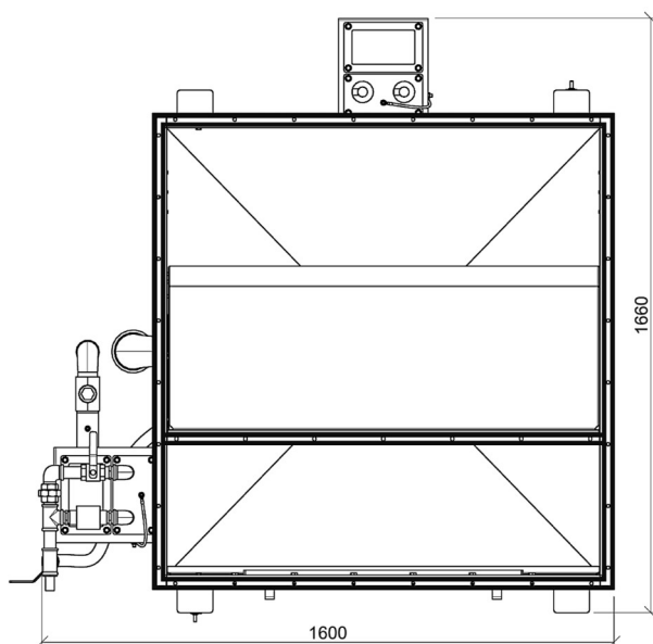
Rysunek 12 Część dolna – Widok 3
