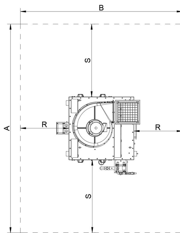
Rysunek 19 Przestrzeń robocza – Rzut góry
