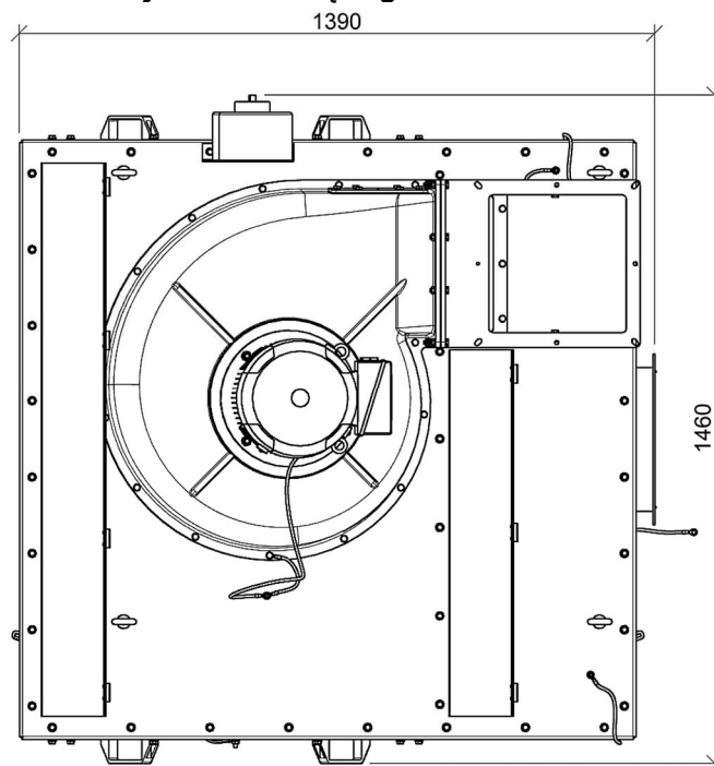
Rysunek 15 Część górna – Widok 3
