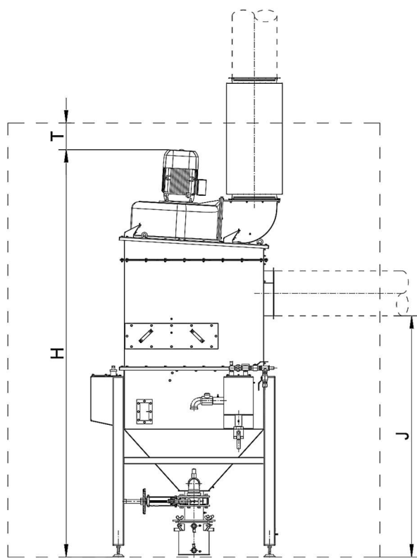
Rysunek 18 Przestrzeń robocza – Rzut boczny
