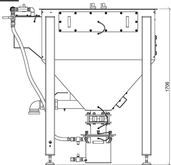
Rysunek 10 Część dolna – Widok 1
