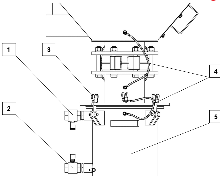
Rysunek 26 Pojemnik na szlam
