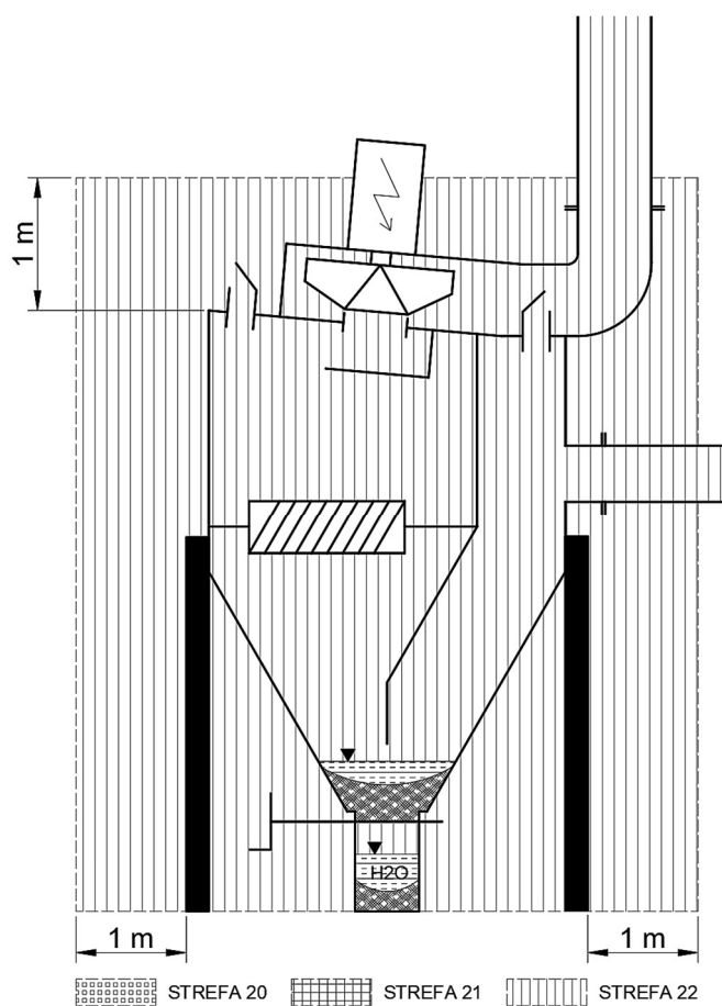
Rysunek 2 Strefy niebezpieczne podczas postoju dla pyłu
