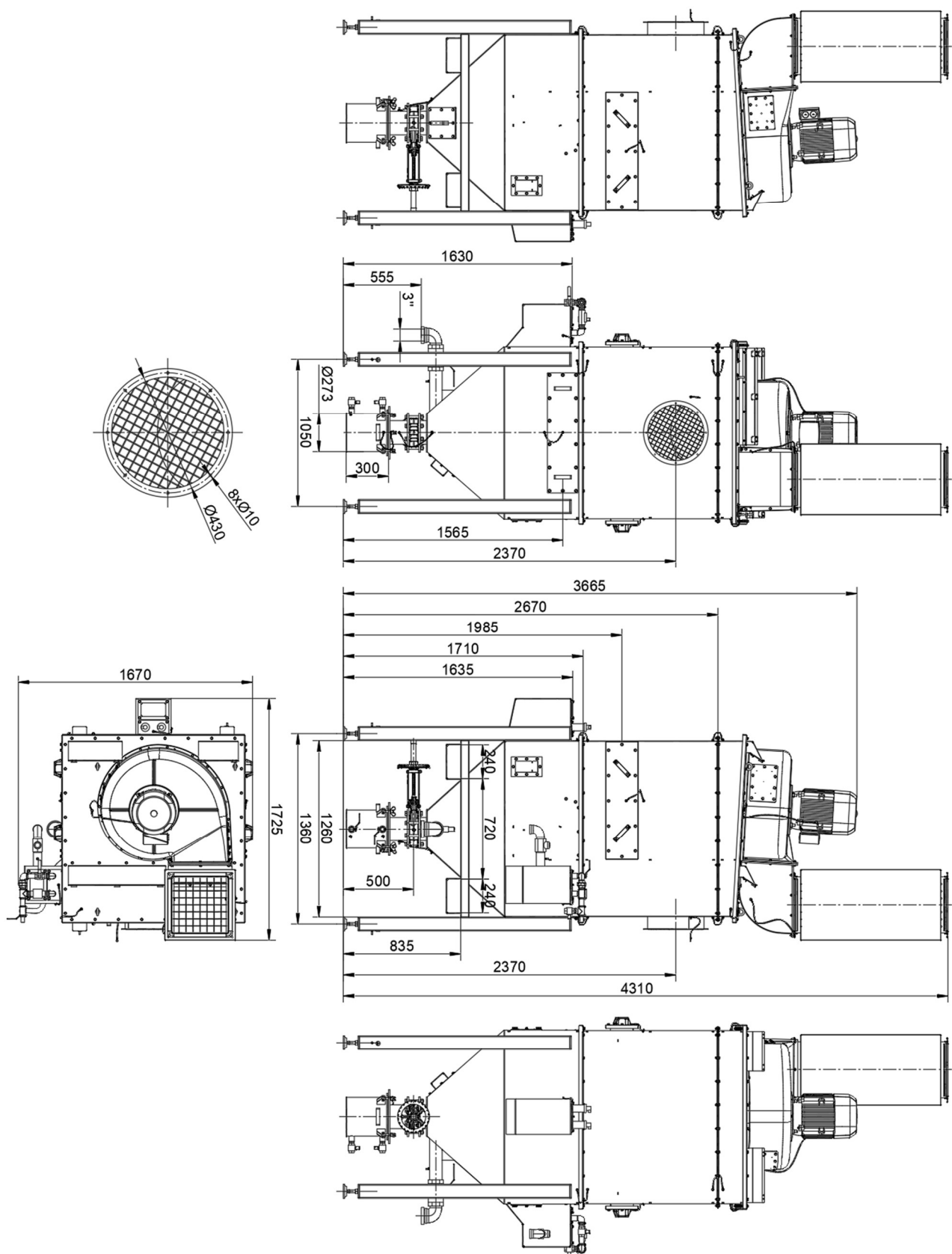
Rysunek 9 Wymiary gabarytowe urządzenia WET-6000-ALU/Ex
