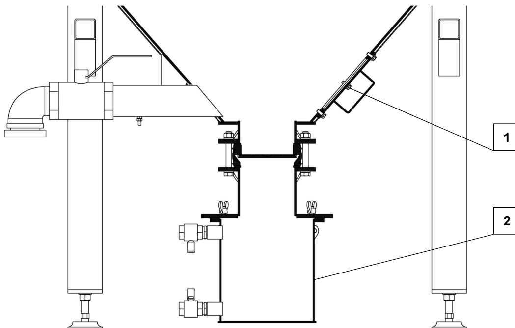
Rysunek 28 Przekrój zbiornika głównego
