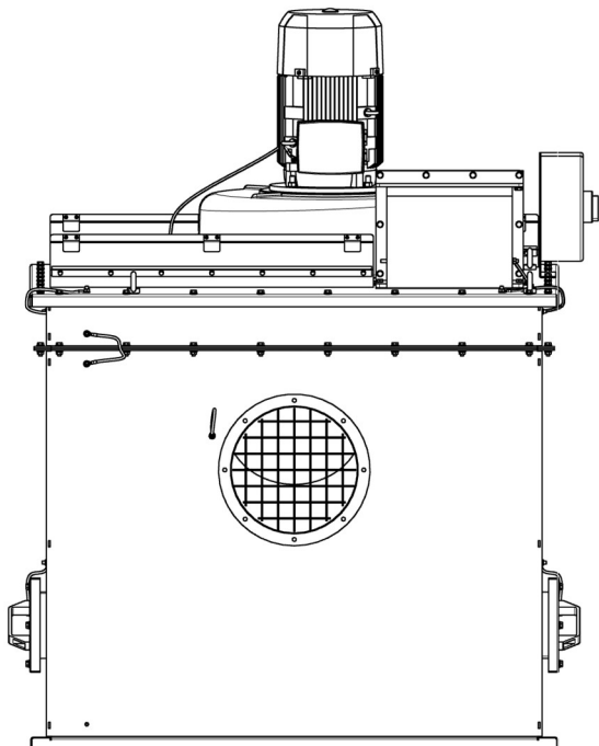
Rysunek 13 Część górna – Widok 1
