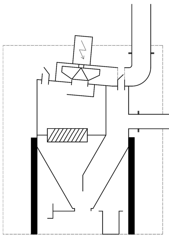
Rysunek 5 Strefy niebezpieczne podczas postoju dla gazów
