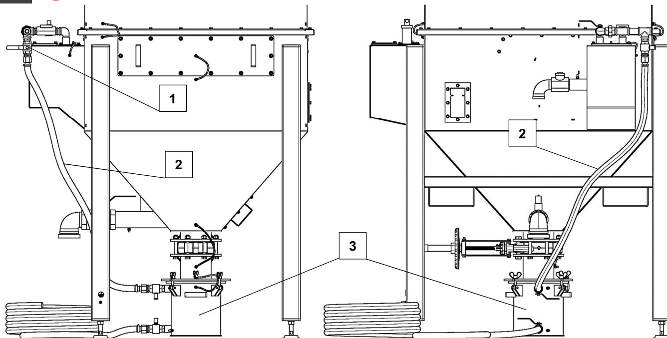
Rysunek 24 Połączenie sieci wodociągowej z pojemnikiem na szlam
