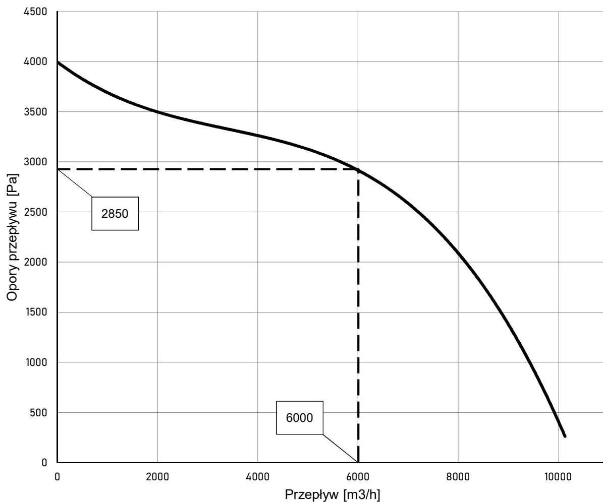
Wykres 1 Charakterystyka przepływowa urządzenia WET-6000-ALU/Ex
