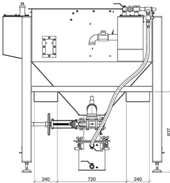
Rysunek 11 Część dolna – Widok 2
