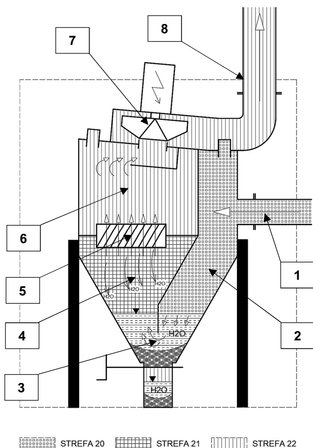
Rysunek 1 Strefy niebezpieczne podczas pracy dla pyłu
