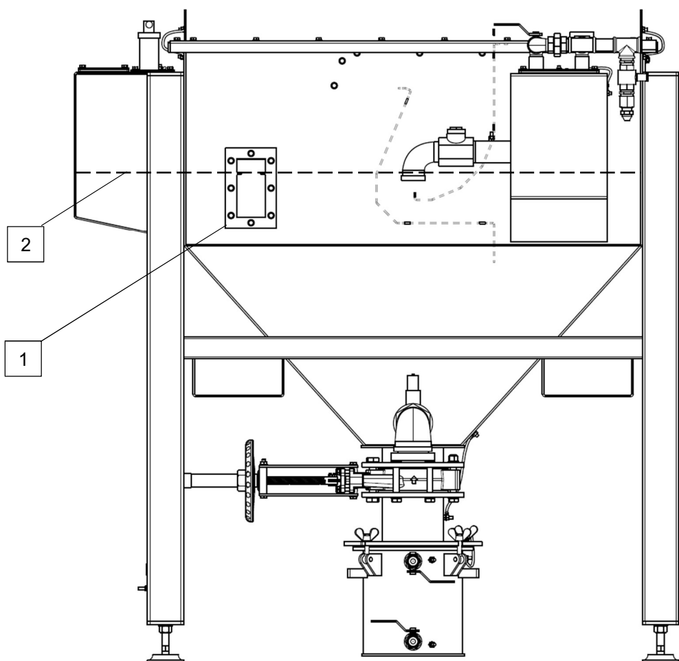
Rysunek 21 Zbiornik główny z wizjerami
