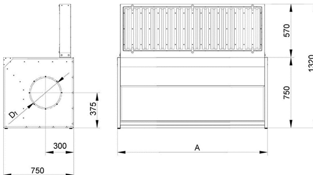
Rysunek 1 Budowa i wymiary stanowisk SLOT
