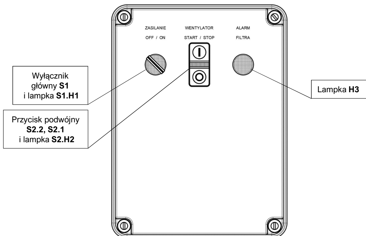
Rysunek 3 Wygląd elewacji zespołu elektrycznego urządzenia MISTOL MIX-5000
