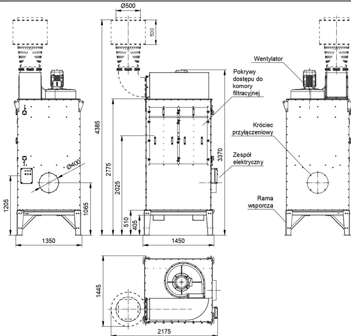
Rysunek 2 Budowa i wymiary urządzenia MISTOL MIX-500
