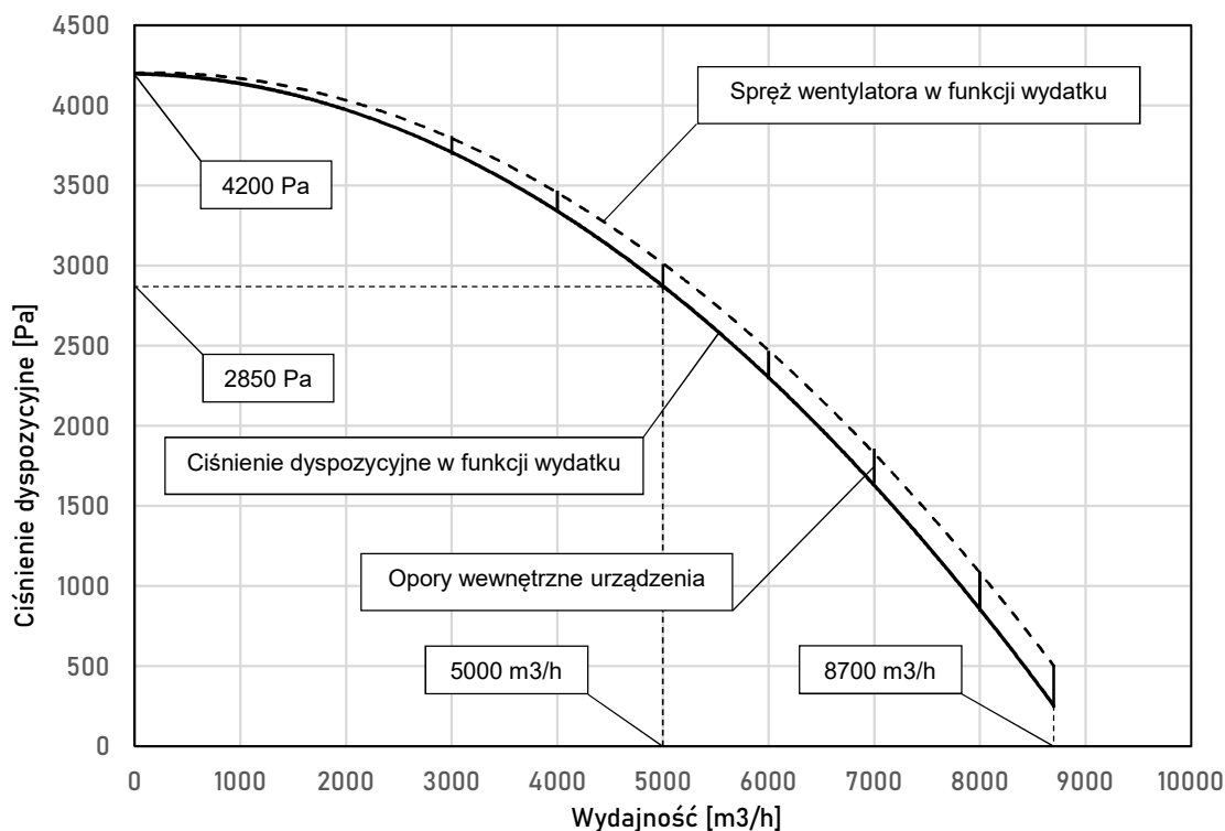
Rysunek 1 Charakterystyka przepływowa urządzenia MISTOL MIX-5000
