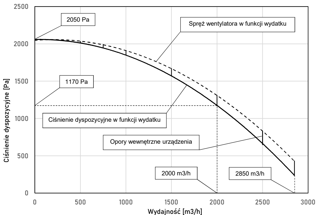
Rysunek 1 Charakterystyka przepływowa urządzenia MISTOL MIX-2000
