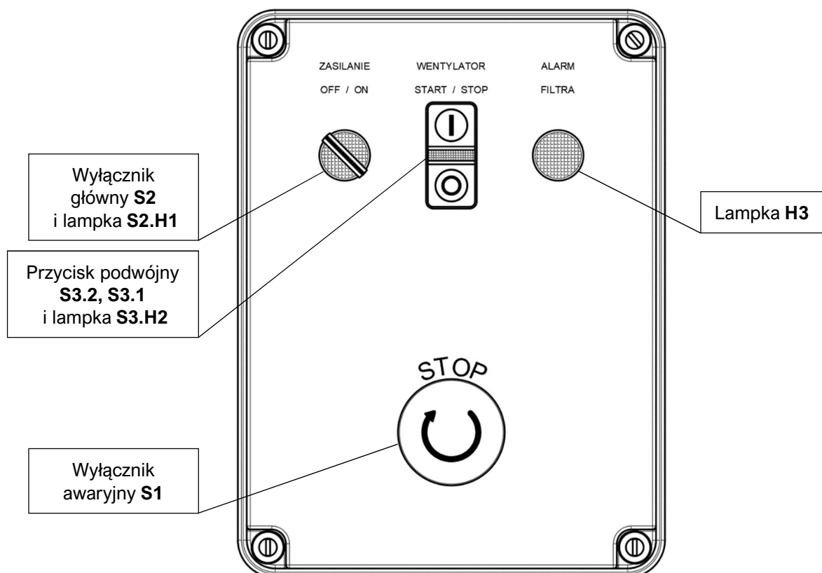
Rysunek 3 Wygląd elewacji zespołu elektrycznego urządzenia MISTOL MIX-2000
