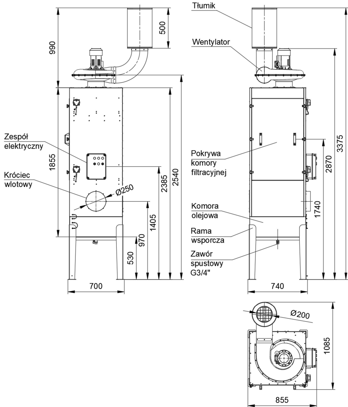
Rysunek 2 Budowa i wymiary urządzenia MISTOL MIX-2000
