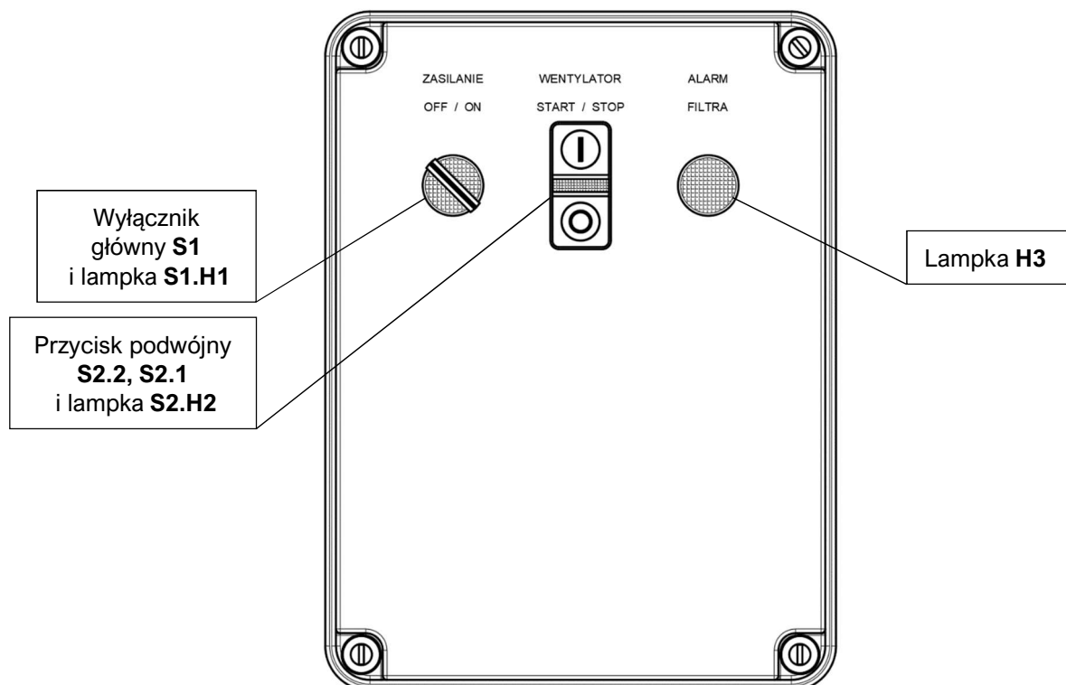
Rysunek 3 Wygląd elewacji zespołu elektrycznego urządzenia MISTOL DUST-5000
