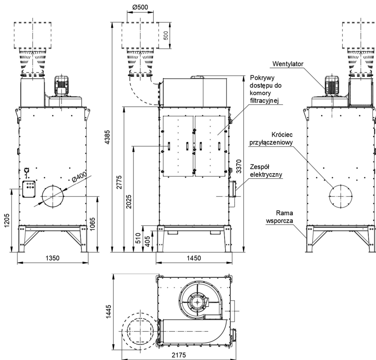
Rysunek 2 Budowa i wymiary urządzenia MISTOL DUST-5000
