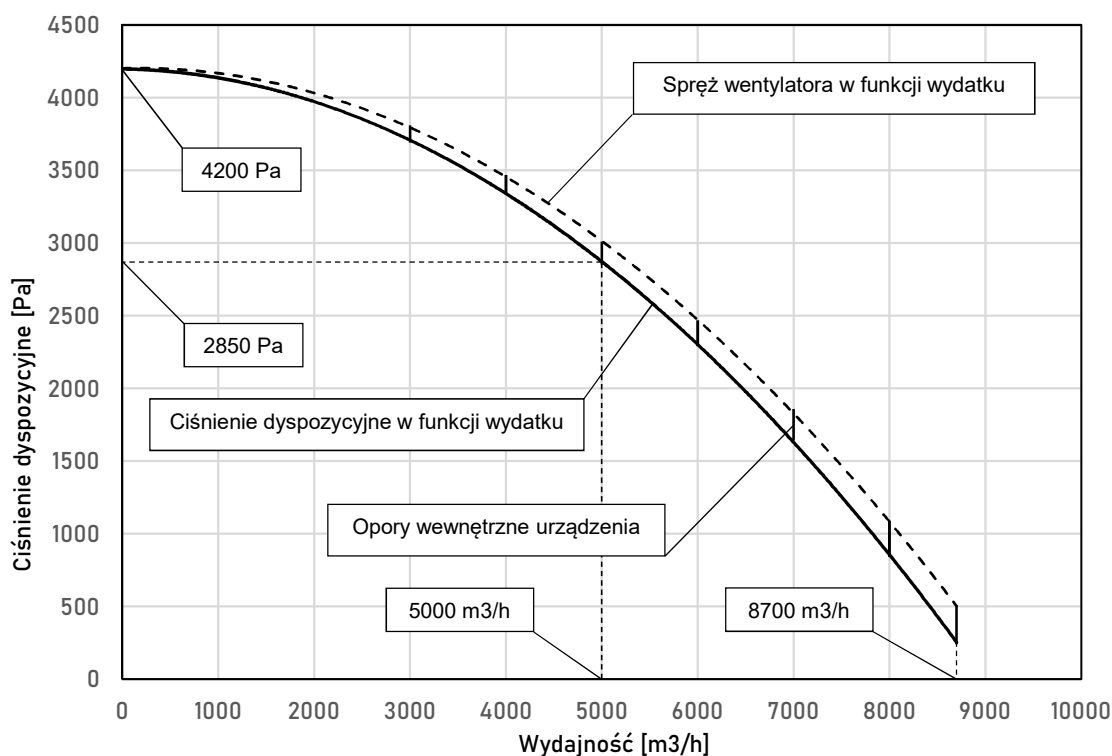
Rysunek 1 Charakterystyka przepływowa urządzenia MISTOL DUST-5000
