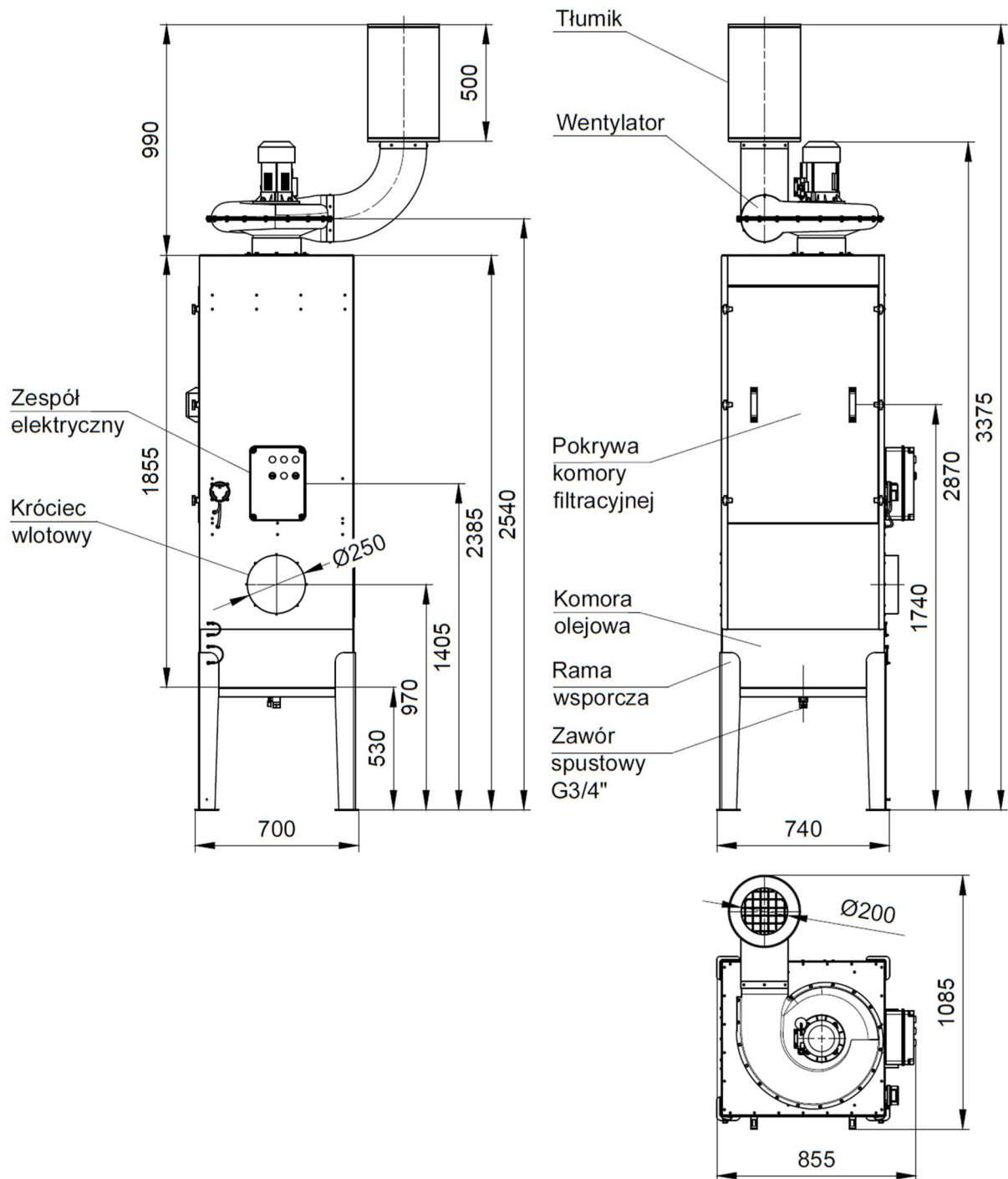
Rysunek 2 Budowa i wymiary urządzenia MISTOL DUST-2000
