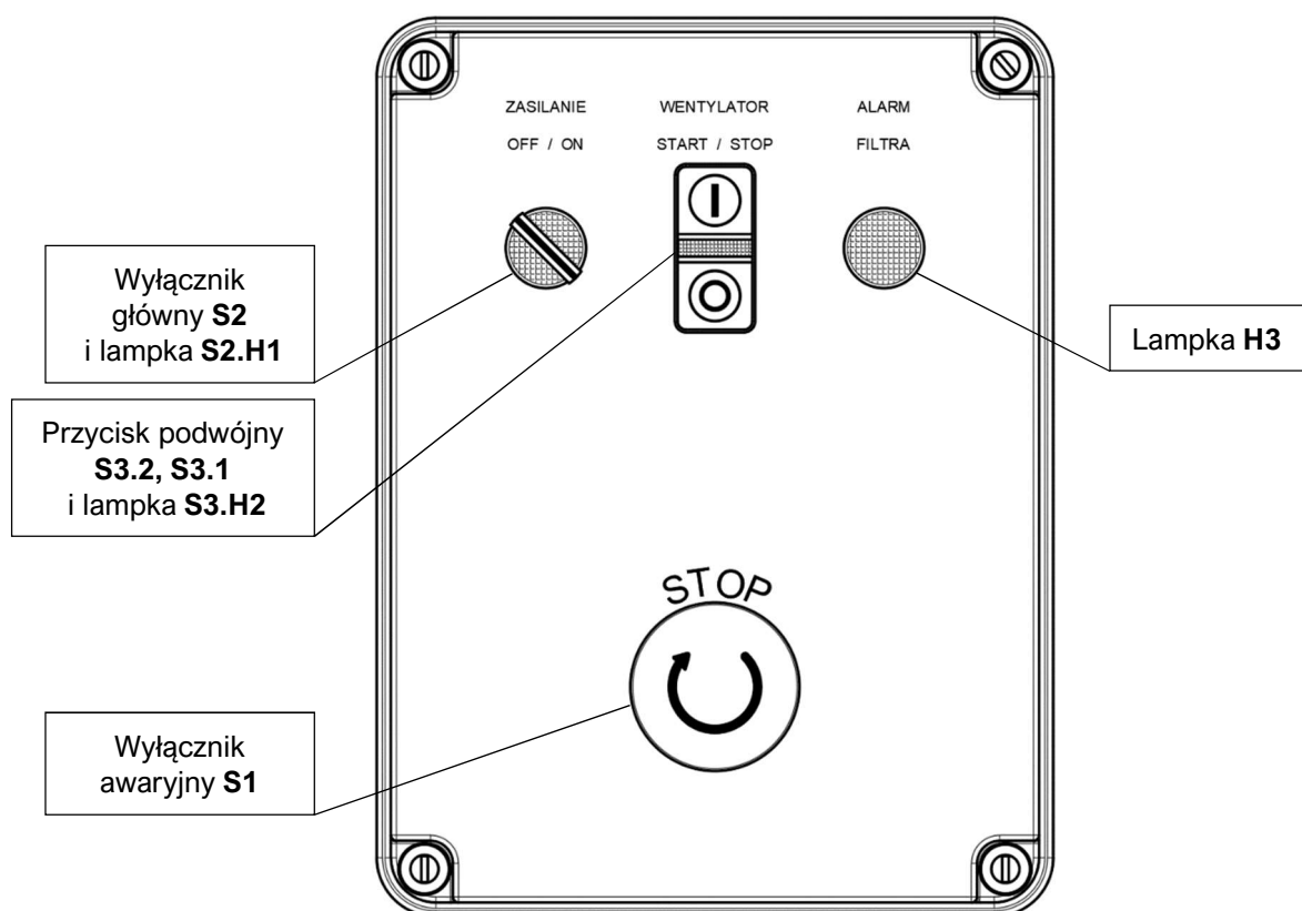
Rysunek 3 Wygląd elewacji zespołu elektrycznego urządzenia MISTOL DUST-2000
