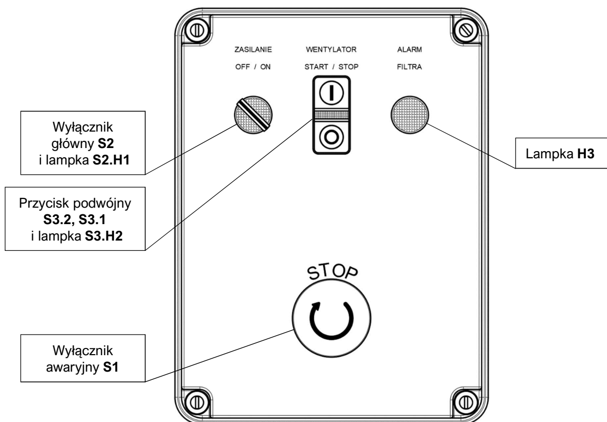
Rysunek 3 Wygląd elewacji zespołu elektrycznego urządzenia MISTOL DUST-1000
