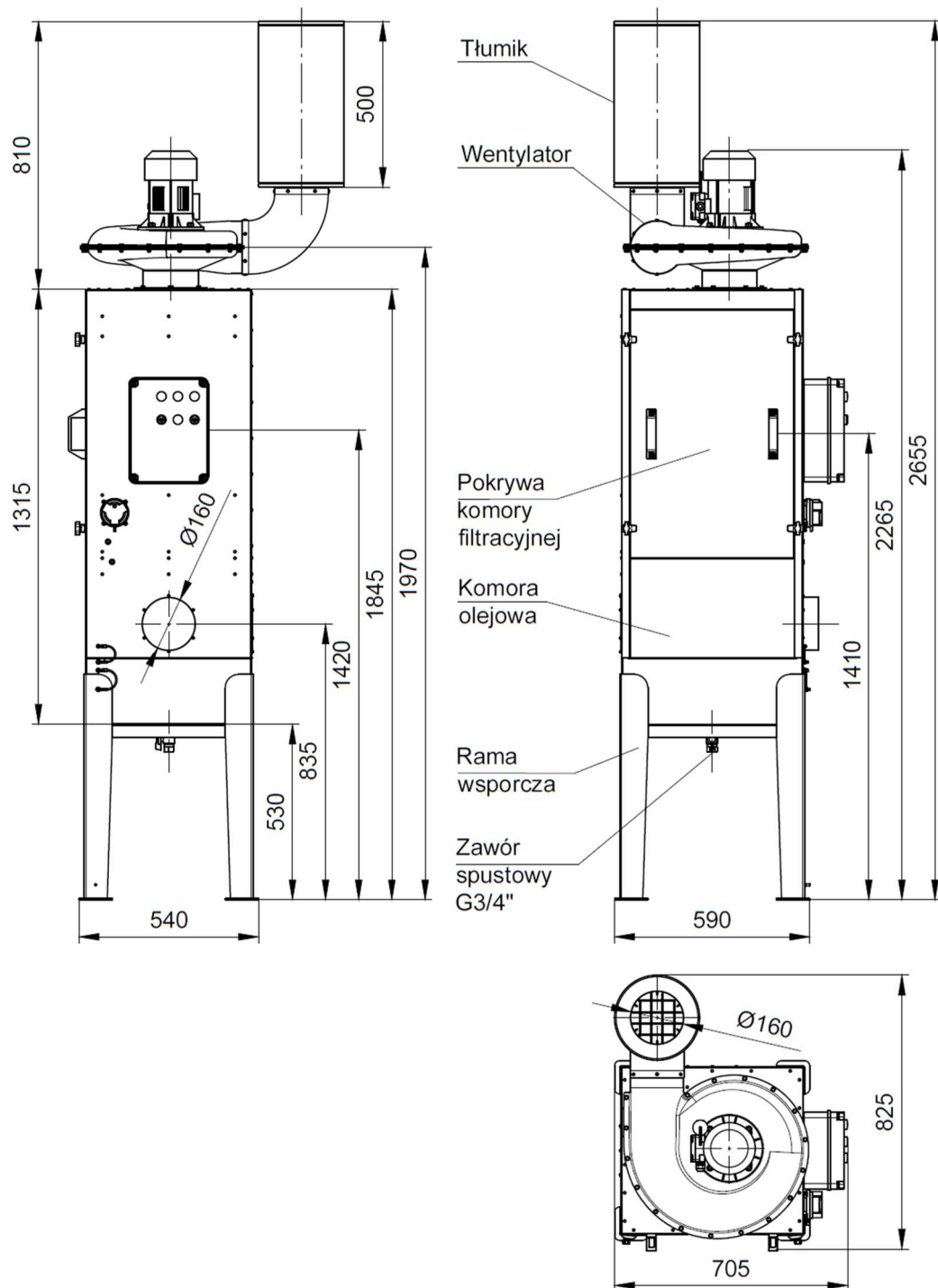
Rysunek 2 Budowa i wymiary urządzenia MISTOL DUST-1000
