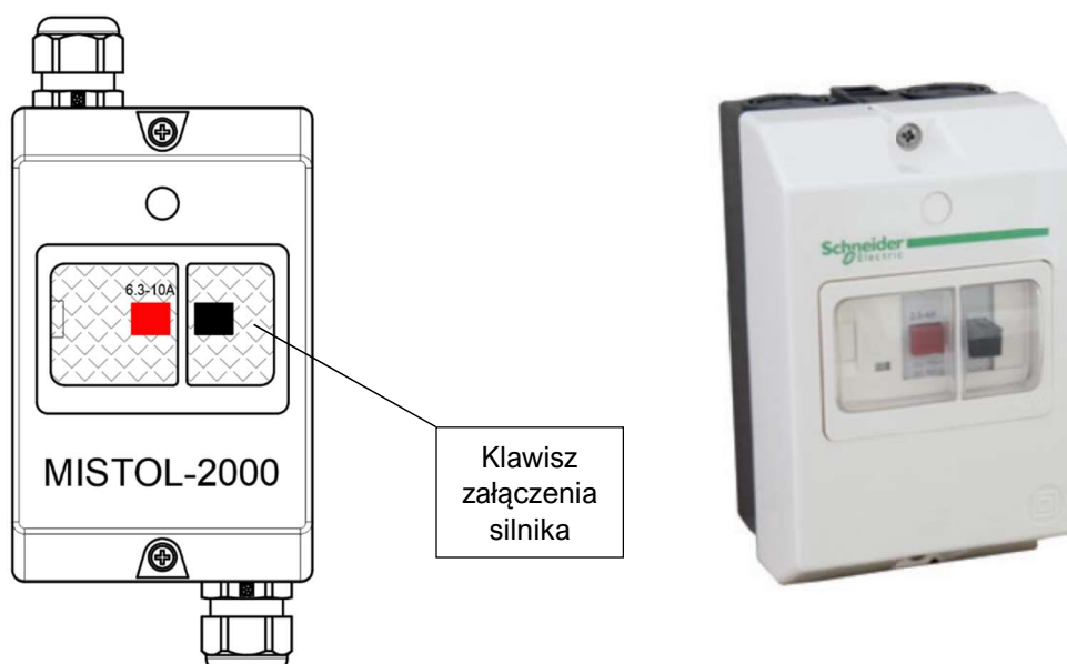
Rysunek 3 Wygląd elewacji wyłącznika silnikowego urządzenia MISTOL-2000
