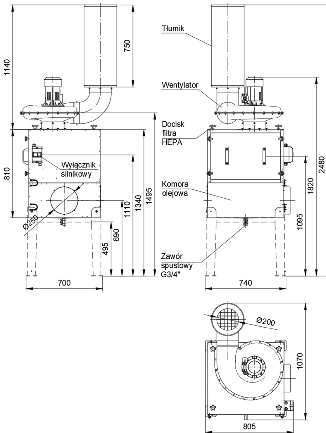
Rysunek 2 Budowa i wymiary urządzenia MISTOL-2000
