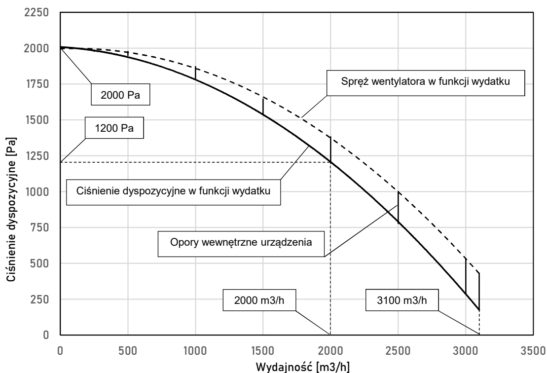
Rysunek 1 Charakterystyka przepływowa urządzenia MISTOL-2000
