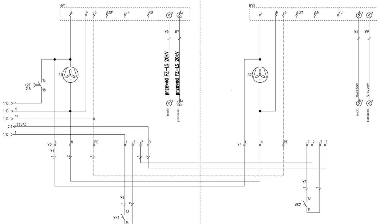
Schemat 3 Obwód wysokiego napięcia
