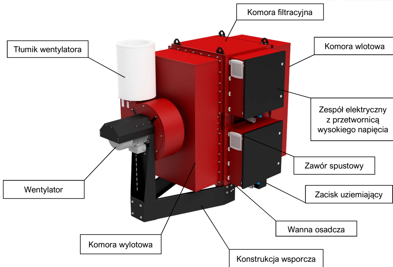
Fotografia 1 Budowa urządzenia PROTON-8000
