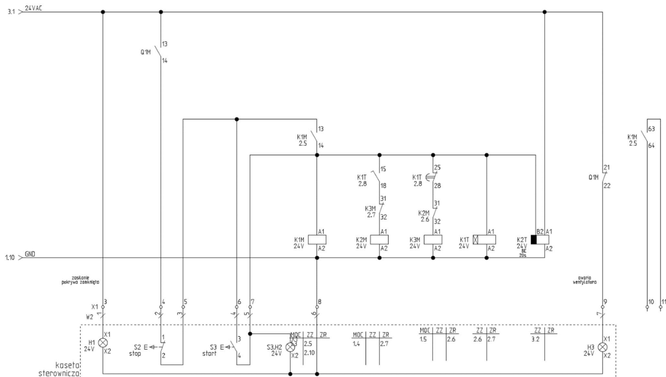
Schemat 2 Układ rozruchowy i sterowania
