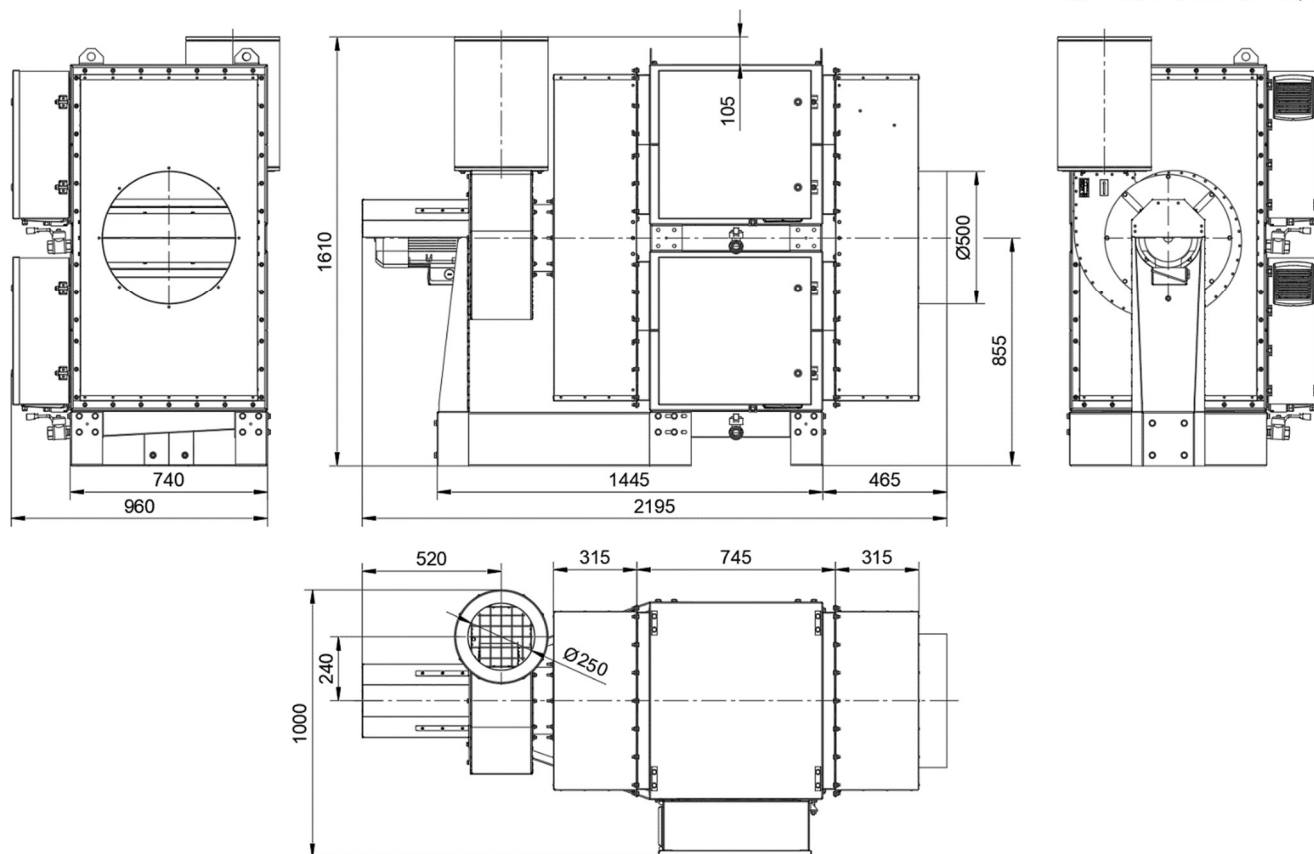
Rysunek 1 Wymiary gabarytowe urządzenia PROTON-8000
