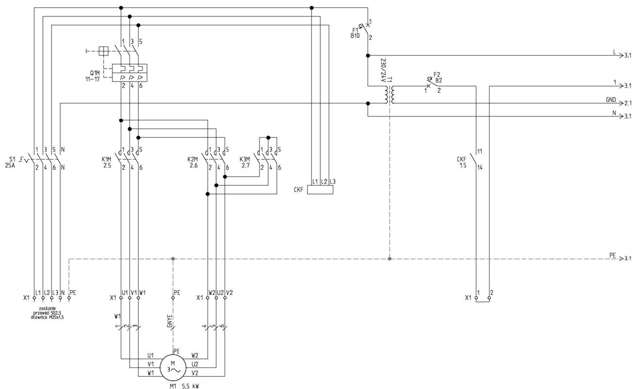
Schemat 1 Obwód prądowy zasilania wentylatora
