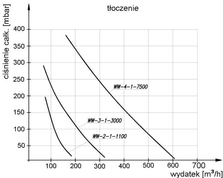
Rys. 2 Charakterystyki przepływowe
