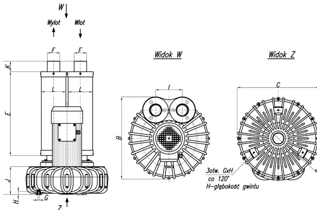
Rys. 1 Wymiary wentylatora WW
