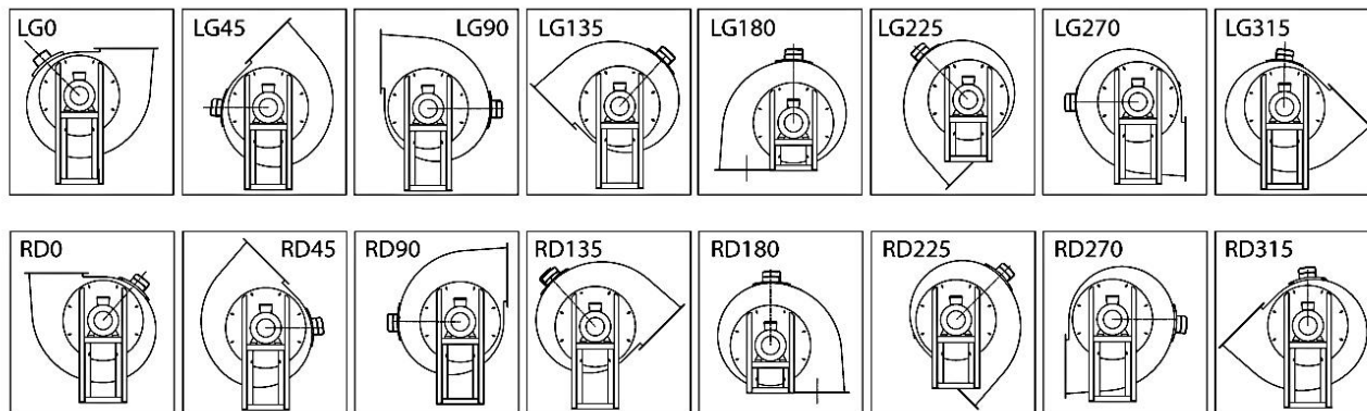
Rys. 3 Pozycje montażu wentylatora WPA-S-N/Ex
