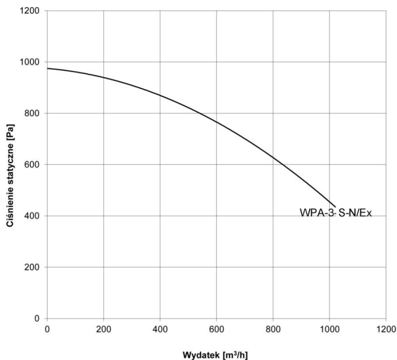
Charakterystyka przepływowa
