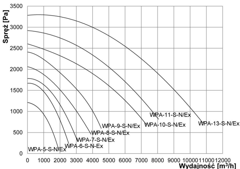
Rys.2 Charakterystyki przepływowe wentylatorów typu WPA-S-N/Ex
