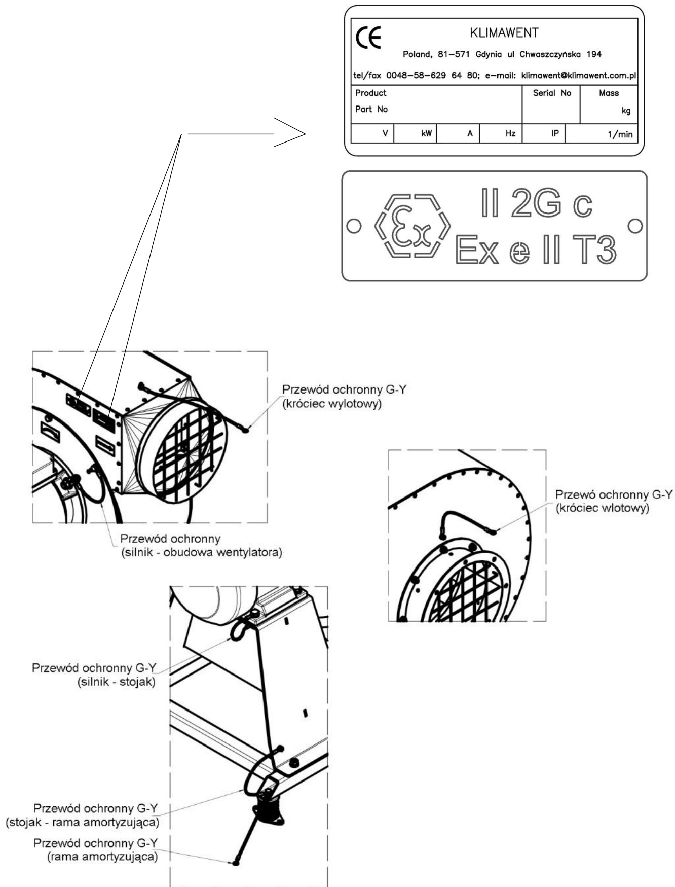
Rys. 5 Rozmieszczenie przewodów ochronnych i tabliczek znamionowych
