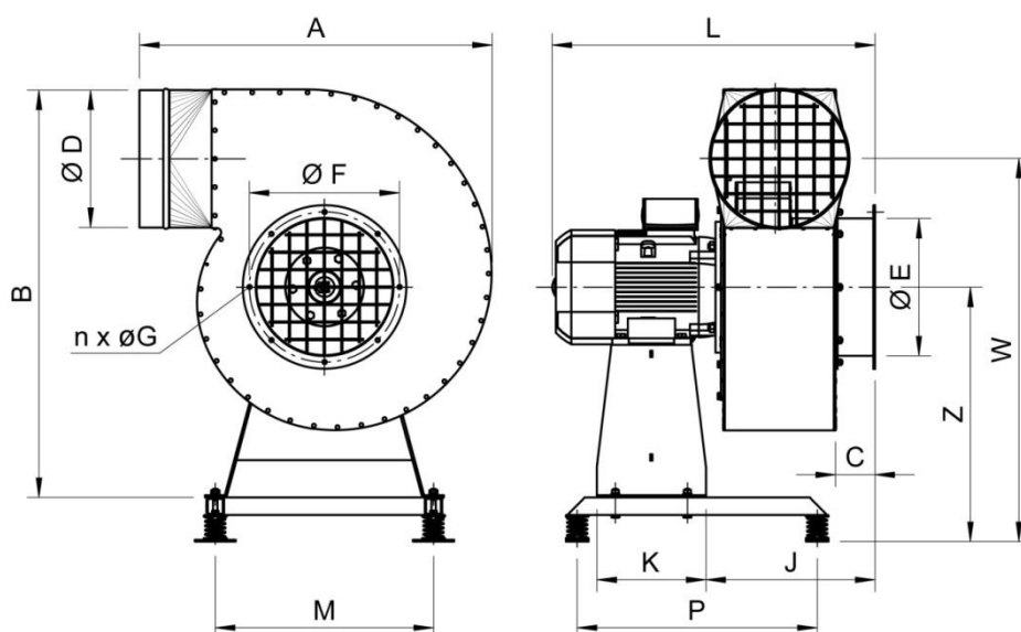
Rys.1 Wentylator z serii WPA-S-N/Ex, budowa, wymiary
