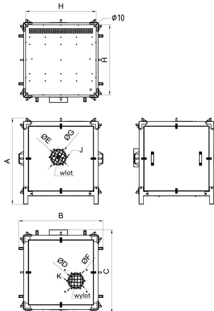
Rys. 1 Wymiary komory wentylatorowej typu WPA-BOX
