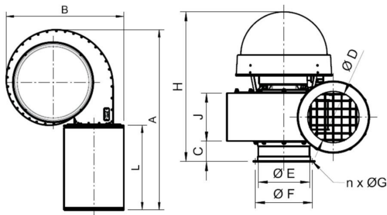
Rys.1 Rysunek gabarytowy
