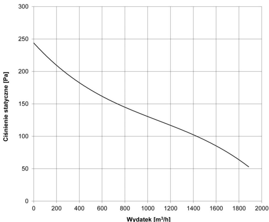
Rys. 1 Charakterystyka przepływowa wentylatora typu WP-11/Ex
