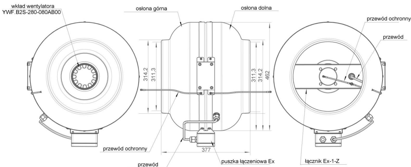
Rys. 2 Wentylator kanałowy WP-11/Ex, budowa i wymiar
