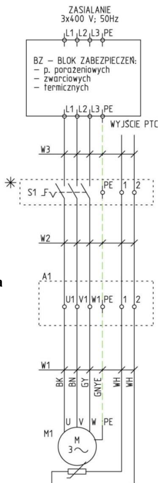
Rys. 3 Przewody ochronne wentylatora
