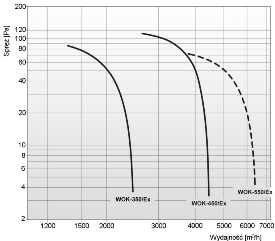
Rys. 1. Charakterystyki przepływowe wentylatorów typu WOK/Ex
