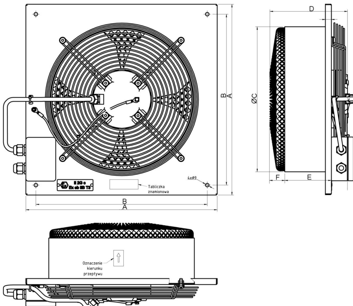
Rys. 2. Budowa i wymiary wentylatorów typu WOK/Ex
