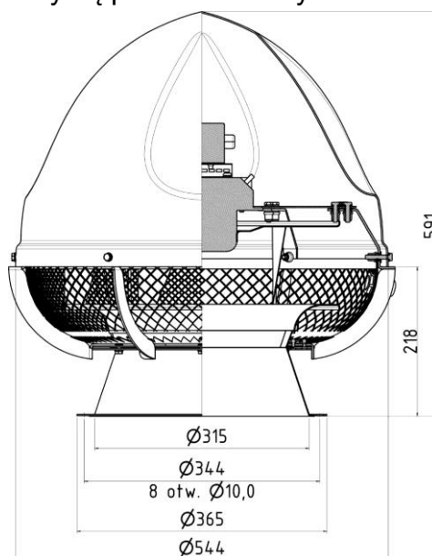
Rys. 1 Budowa i wymiary wentylatora SMART-EC-1300
