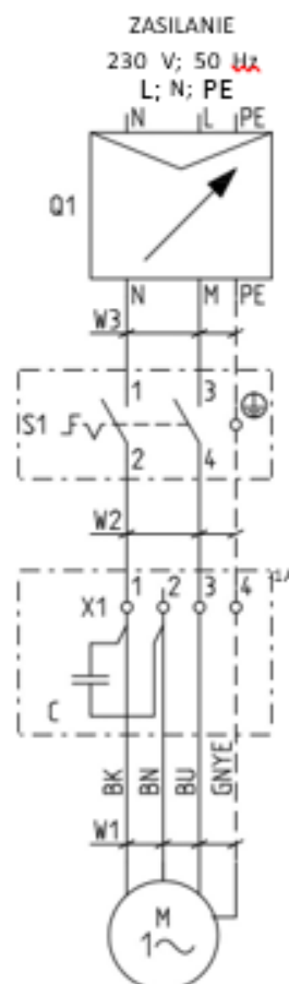
UKŁAD Z REGULACJĄ PRĘDKOŚCI OBROTOWEJ ZA POMOCĄ ELEKTRONICZNEGO REGULATORA PRĘDKOŚCI OBROTOWEJ RP-5-K
