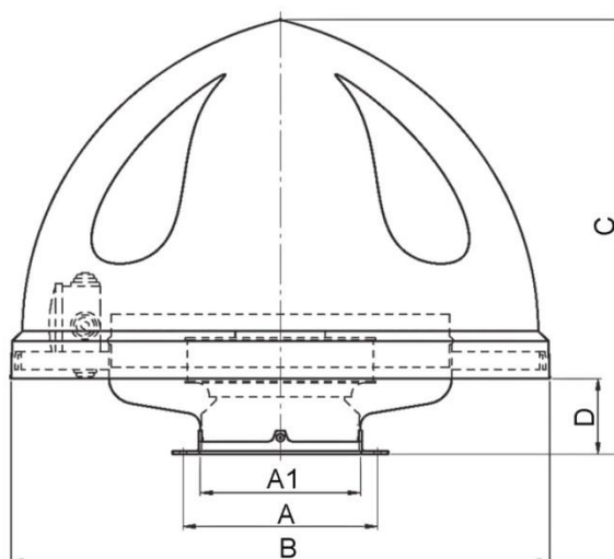
Rys. 1 Wentylatory typu BULLET-N - Budowa i wymiary
