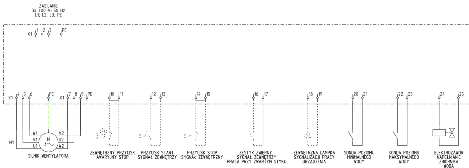
Rys. 4 Schemat blokowy połączeń elektrycznych.
