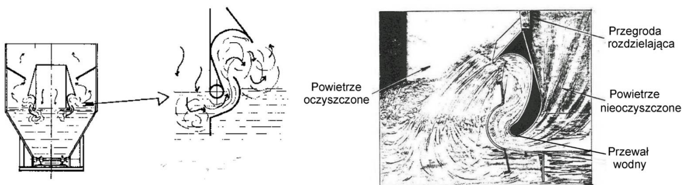
Rys.2. Zasada działania urządzenia filtrowentylacyjnego WET-5000.
