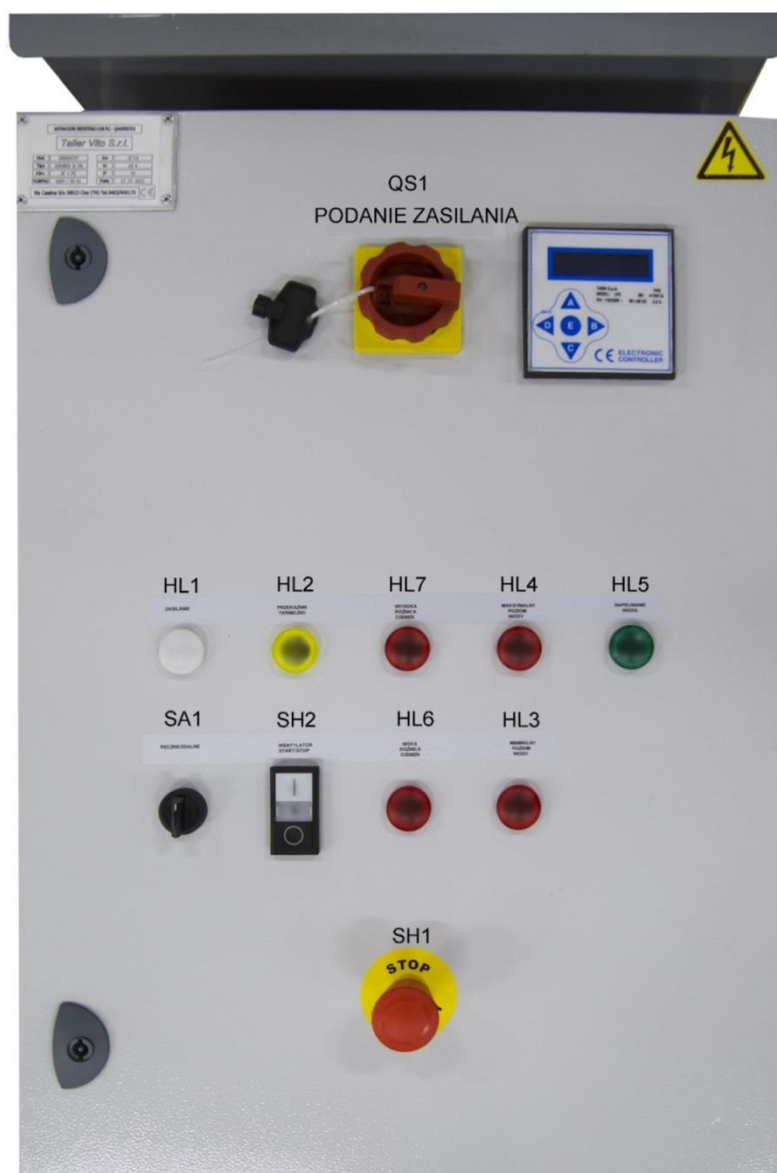
Rys.5. Rozdzielnica elektryczna
