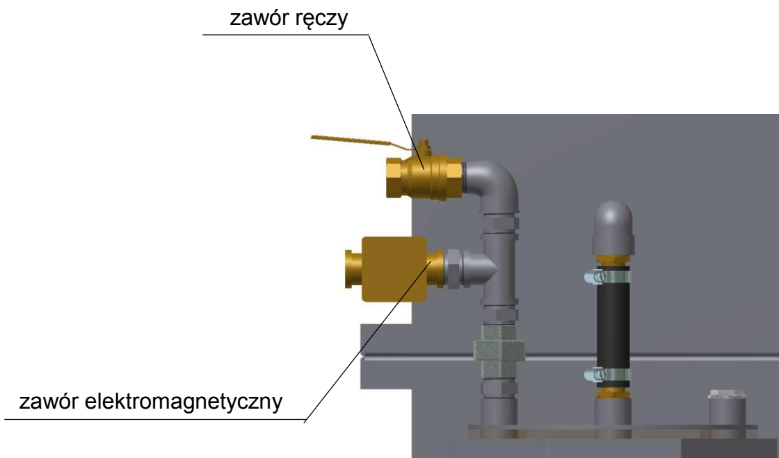
Rys.3. Podłączenie wody zasilającej.
