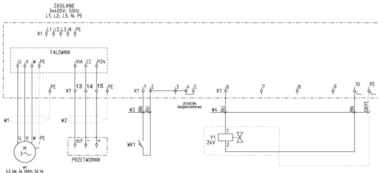
Rys. 4 UFO-A-5000/R, schemat połączeń elektrycznych
