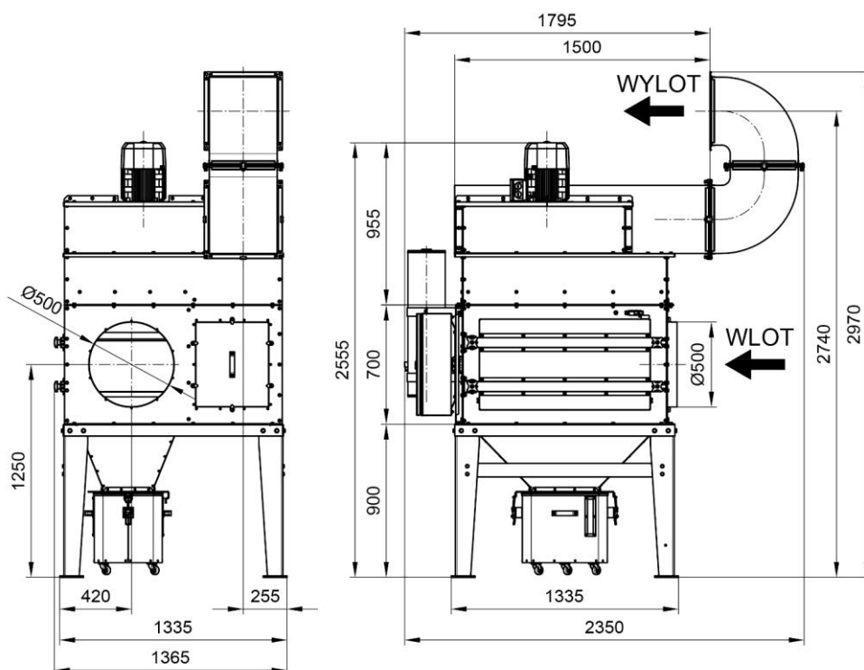
Rys. 2a UFO-A-5000/R RH (z wlotem powietrza z prawej strony) – wymiary
