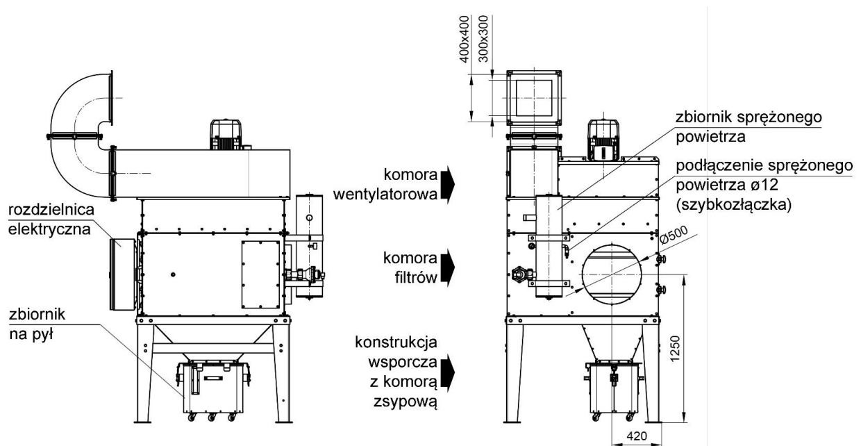
Rys.3 UFO-A-5000 RH i LH, budowa i wymiary
