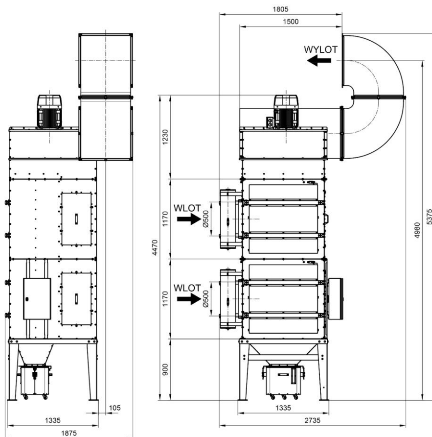
Rys. 2b UFO-A-20000/R LH (z wlotem powietrza z lewej strony) - wymiary
