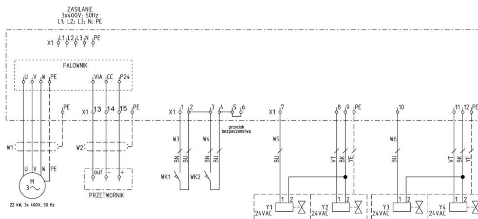
Rys. 4 UFO-A-20000/R, schemat połączeń elektrycznych
