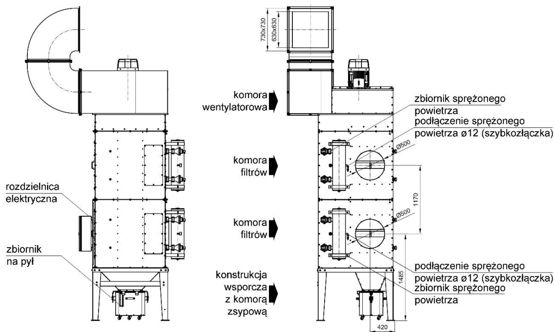
Rys. 3 UFO-A-20000/R, budowa
