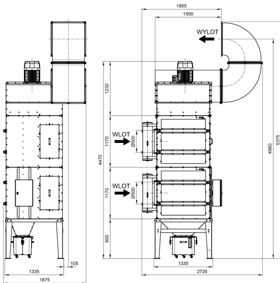
Rys. 2a UFO-A-20000/R RH (z wlotem powietrza z prawej strony) - wymiary
