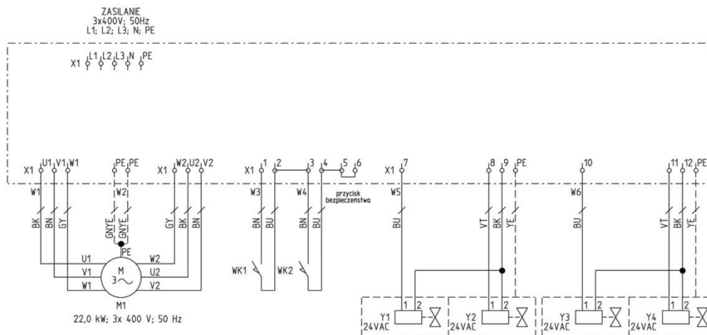
Rys. 4 UFO-A-20000, schemat połączeń elektrycznych
