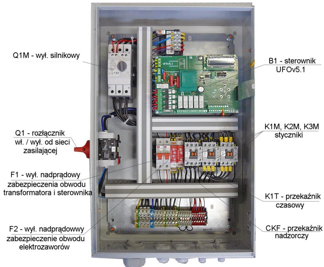
Rys. 7 Rozdzielnica elektryczna ZE-UFO-A – zespoły
