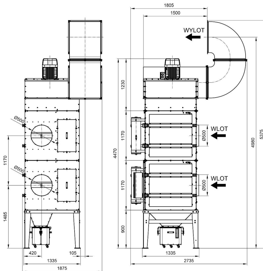
Rys. 2a UFO-A-20000 RH (z wlotem powietrza z prawej strony) - wymiary
