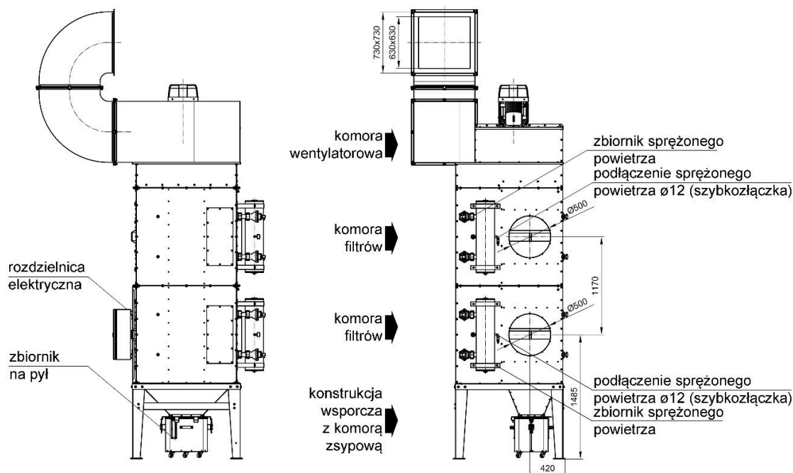
Rys. 3 UFO-A-2000, budowa
