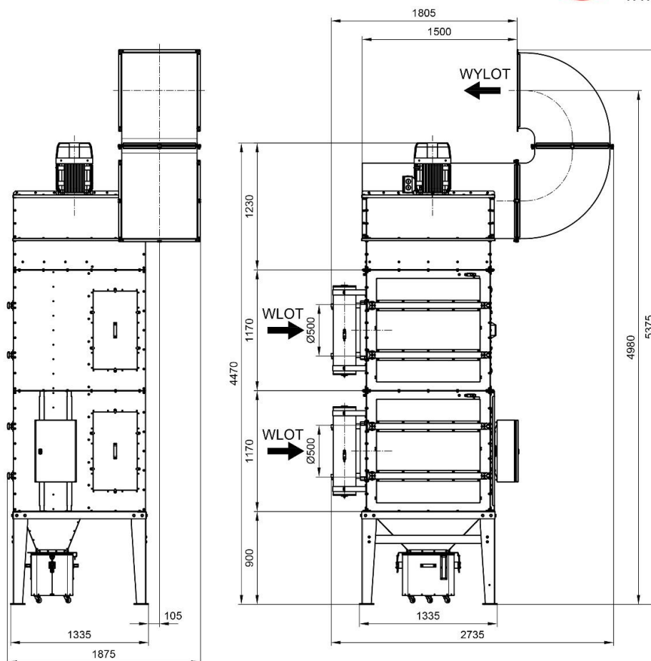
Rys. 2b UFO-A-2000 LH (z wlotem powietrza z lewej strony) - wymiary
