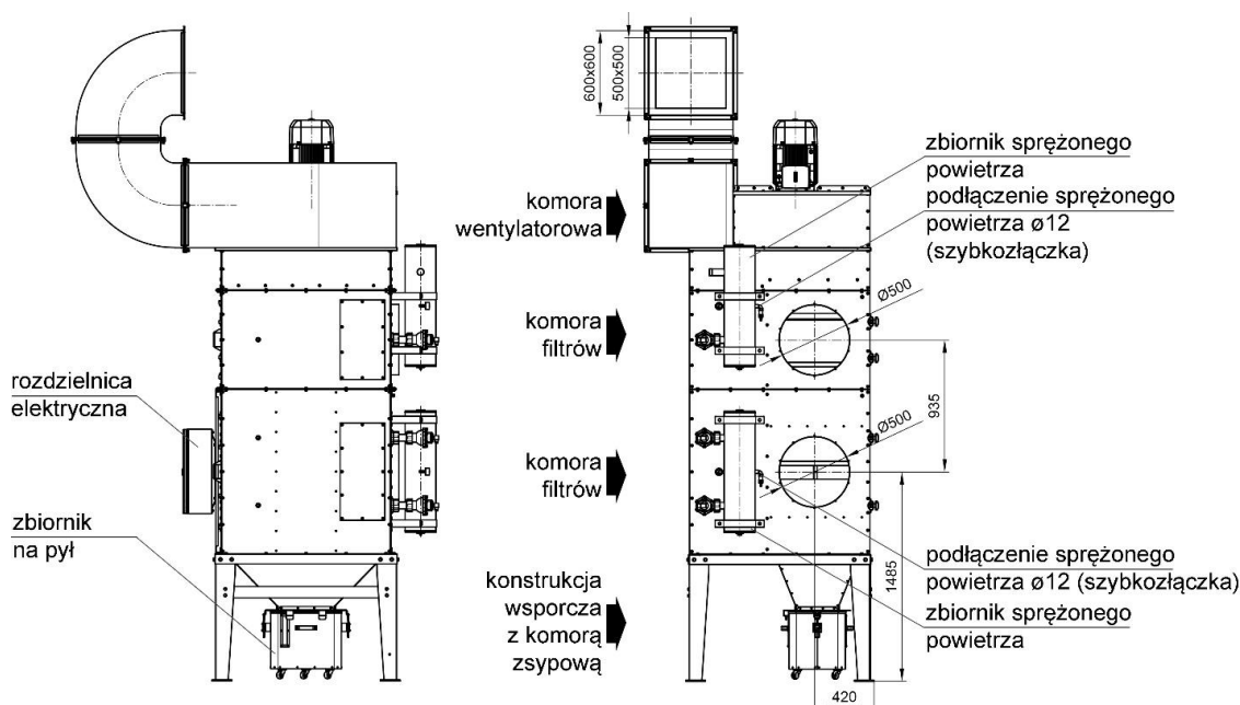
Rys. 3 UFO-A-15000/R, budowa
