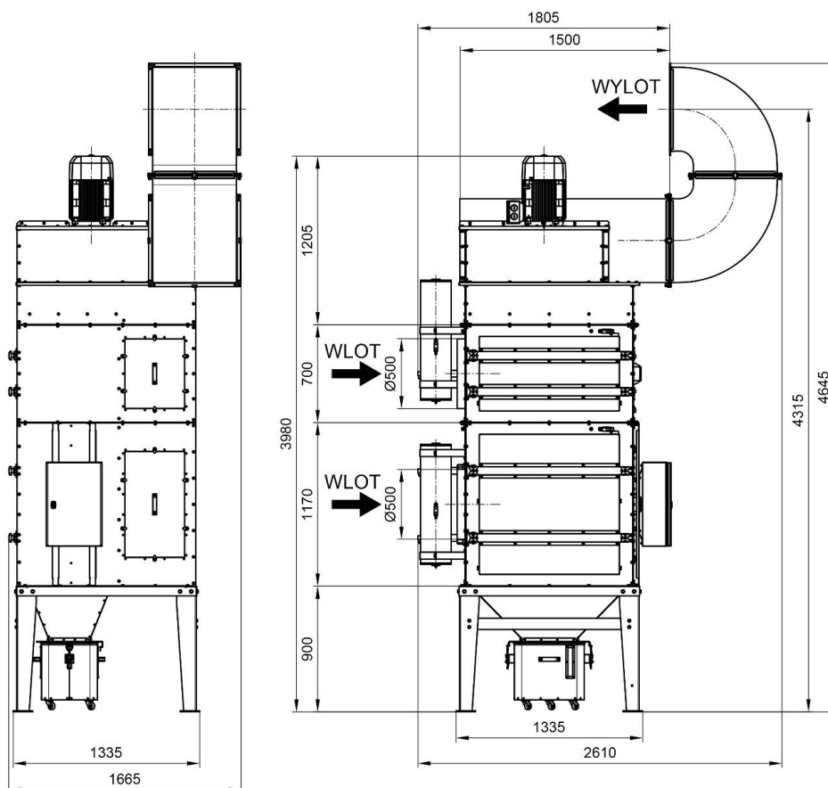
Rys. 2b UFO-A-15000/R LH (z wlotem powietrza z lewej strony) – wymiary
