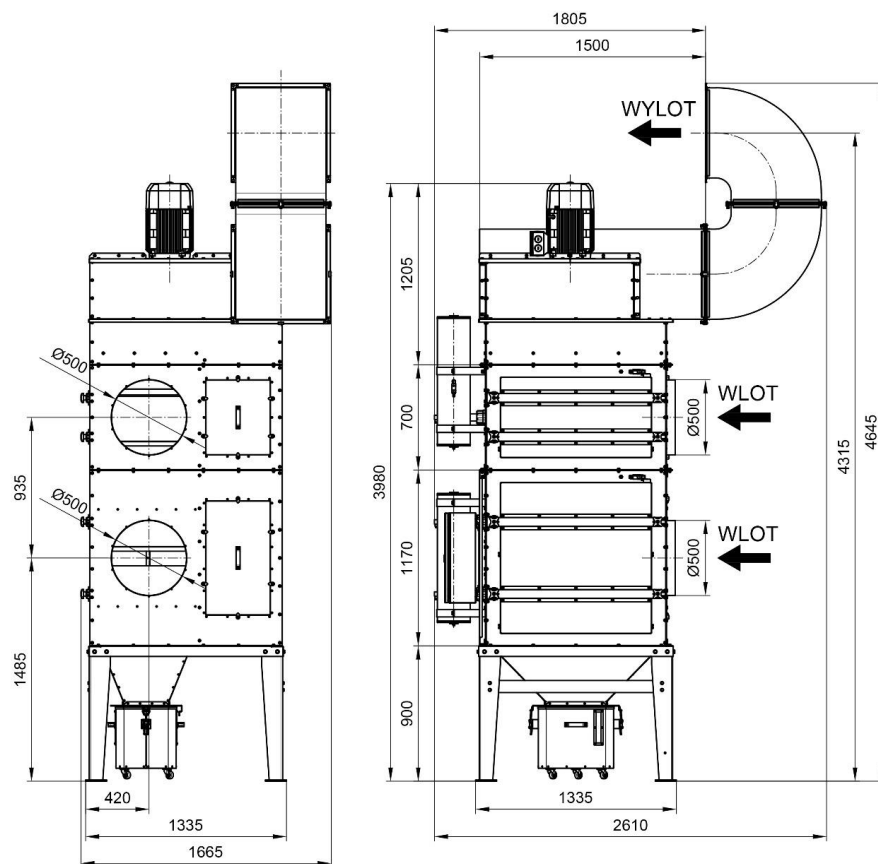
Rys. 2a UFO-A-15000/R RH (z wlotem powietrza z prawej strony) - wymiary
