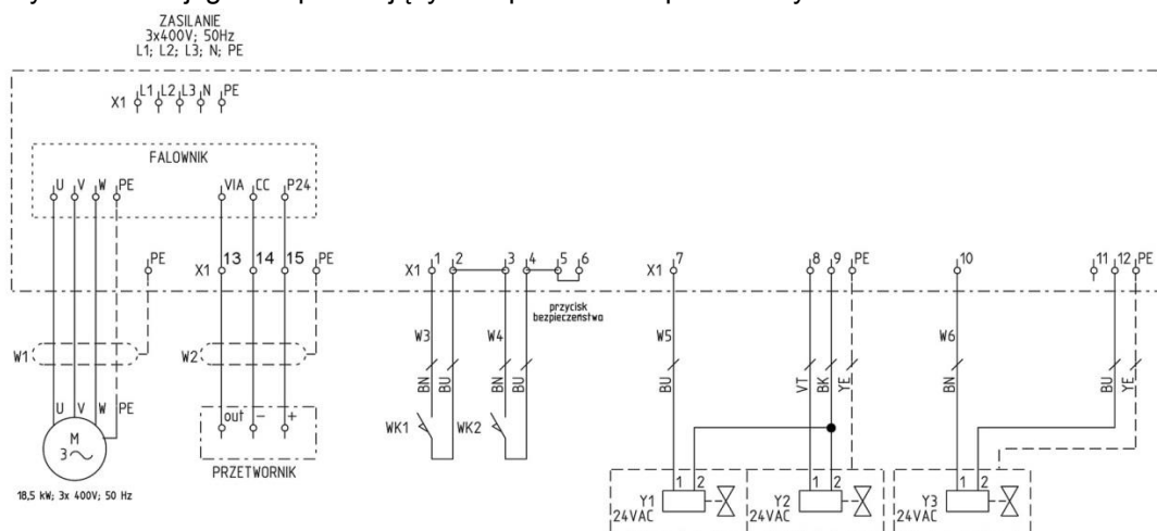
Rys. 4 UFO-A-15000/R, schemat połączeń elektrycznych
