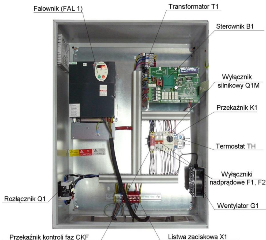
Rys. 7 Rozdzielnica elektryczna ZE-UFO-A – zespoły
