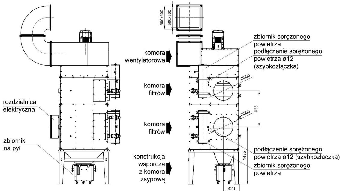
Rys. 3 UFO-A-10000, budowa
