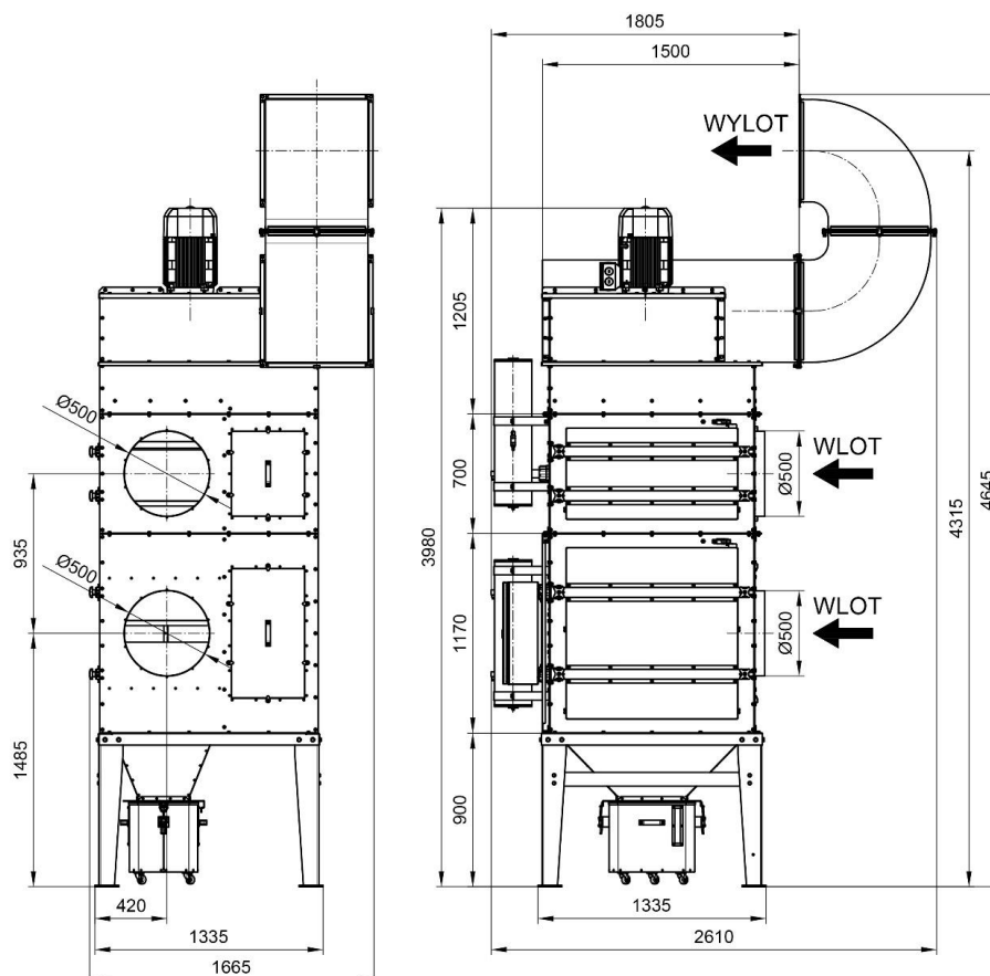
Rys. 2a UFO-A-15000 RH (z wlotem powietrza z prawej strony) - wymiary
