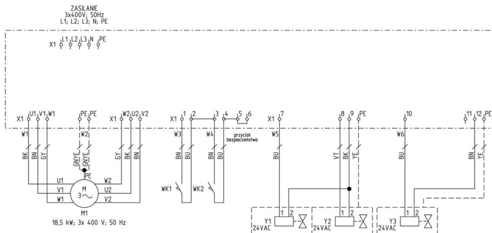
Rys. 4 UFO-A-15000, schemat połączeń elektrycznych
