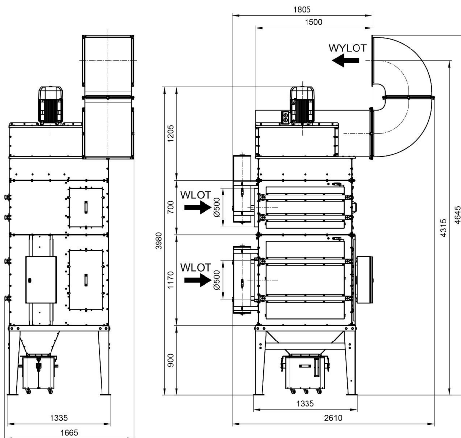
Rys. 2b UFO-A-10000 LH (z wlotem powietrza z lewej strony) - wymiary
