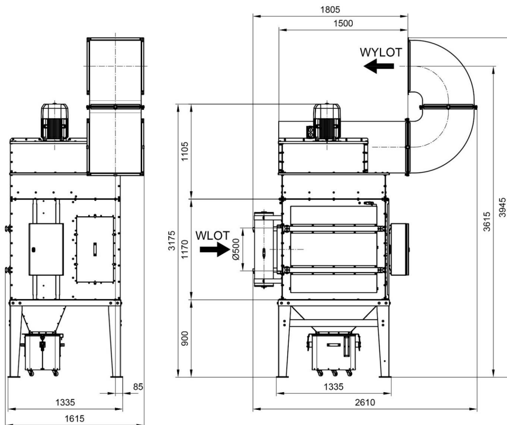
Rys. 2b UFO-A-10000 LH (z wlotem powietrza z lewej strony) - wymiary
