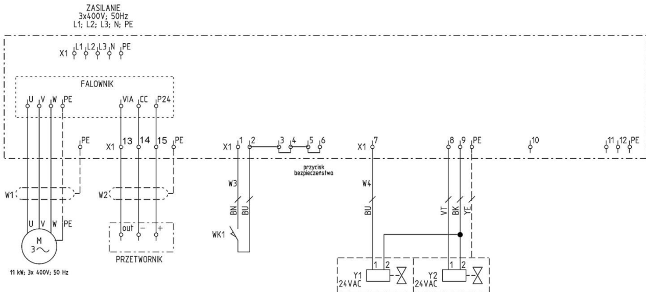
Rys. 4 UFO-A-10000/R, schemat połączeń elektrycznych
