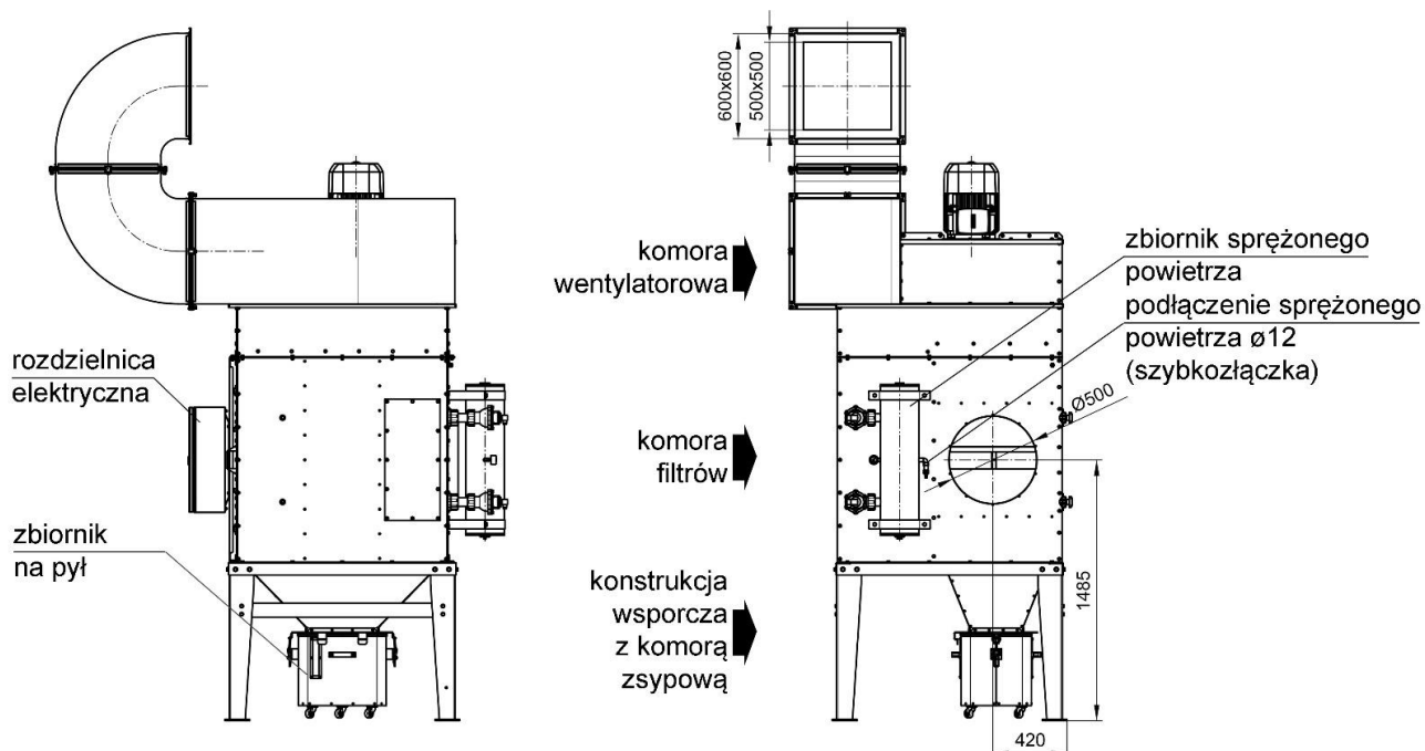
Rys. 3 UFO-A-10000/R, budowa
