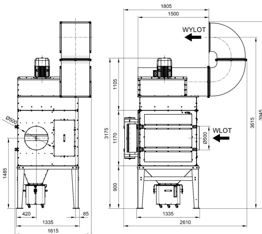
Rys. 2a UFO-A-10000/R RH (z wlotem powietrza z prawej strony) - wymiary
