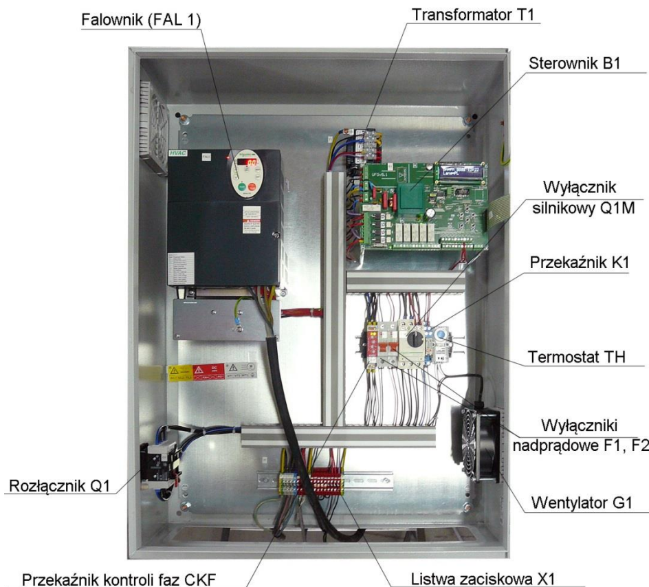
Rys. 7 Rozdzielnica elektryczna - wnętrze
