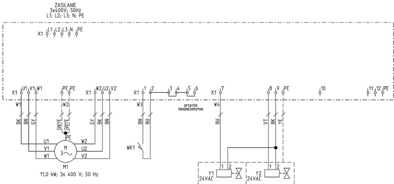
Rys. 4 UFO-A-10000, schemat połączeń elektrycznych
