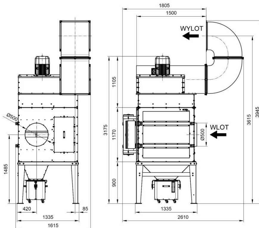
Rys. 2a UFO-A-10000 RH (z wlotem powietrza z prawej strony) - wymiary
