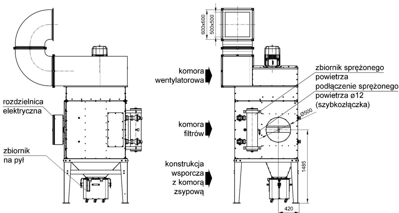
Rys. 3 UFO-A-10000, budowa
