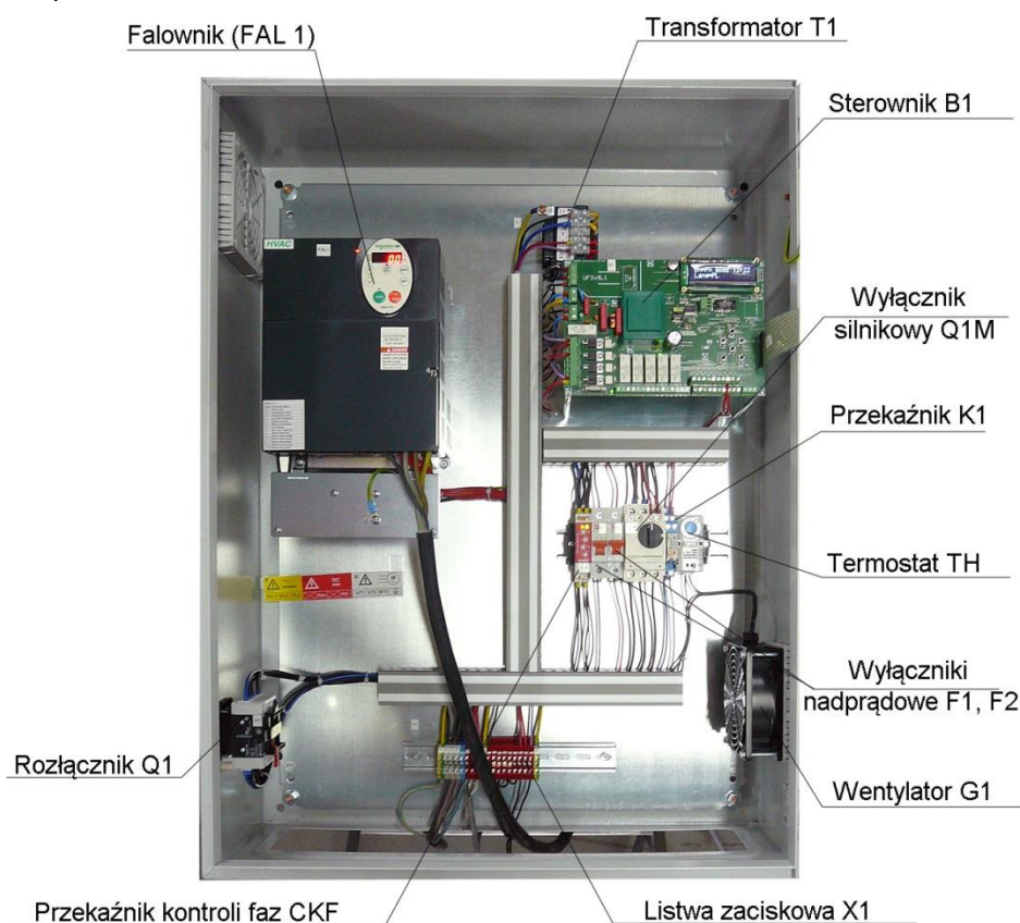
Rys. 8 Zespół elektryczny ZE-UFO-4-M/N-3/R, wnętrze
