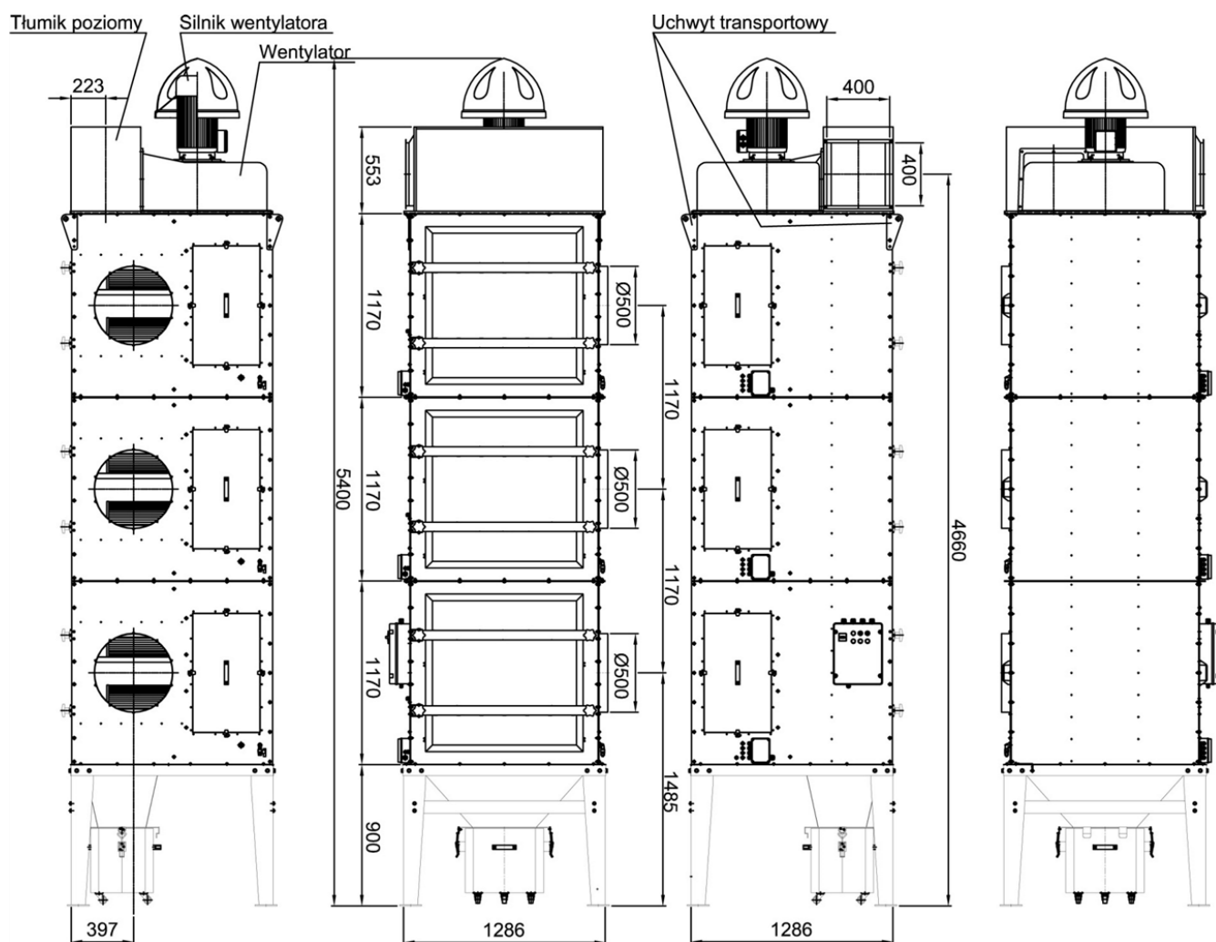
Rys. 1. UFO-4-M/N-3/R, budowa i wymiary
