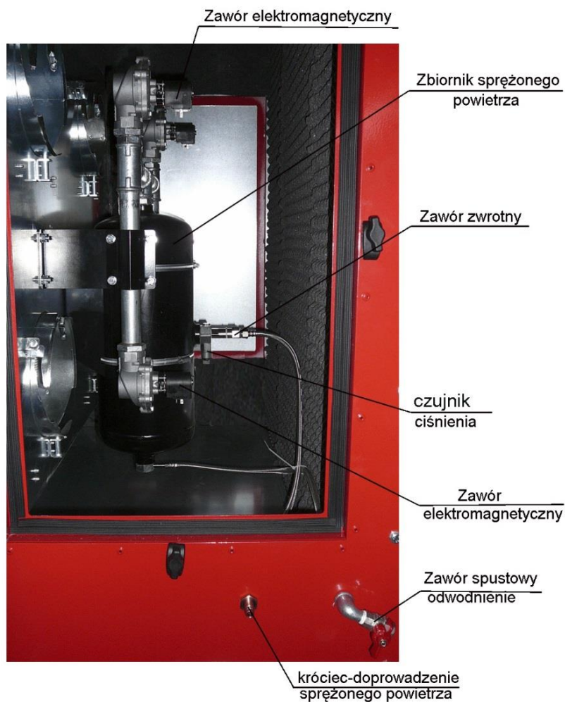
Rys. 3 Instalacja pneumatyczna
