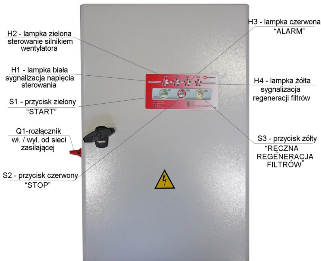
Rys. 6 Zespół elektryczny ZE-UFO-4-MN-3/R, elewacja
