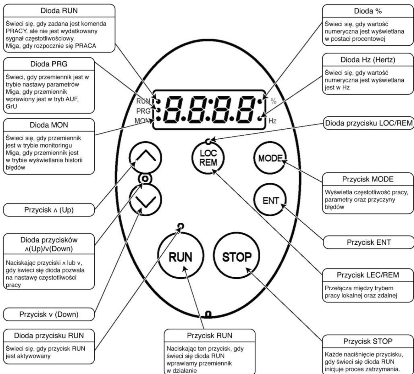
Rys. 10 Opis panelu sterującego przemiennika częstotliwości
