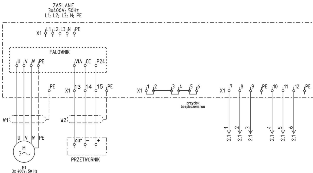
Rys. 4 UFO-4-M/N-3/R, schemat połączeń elektrycznych
