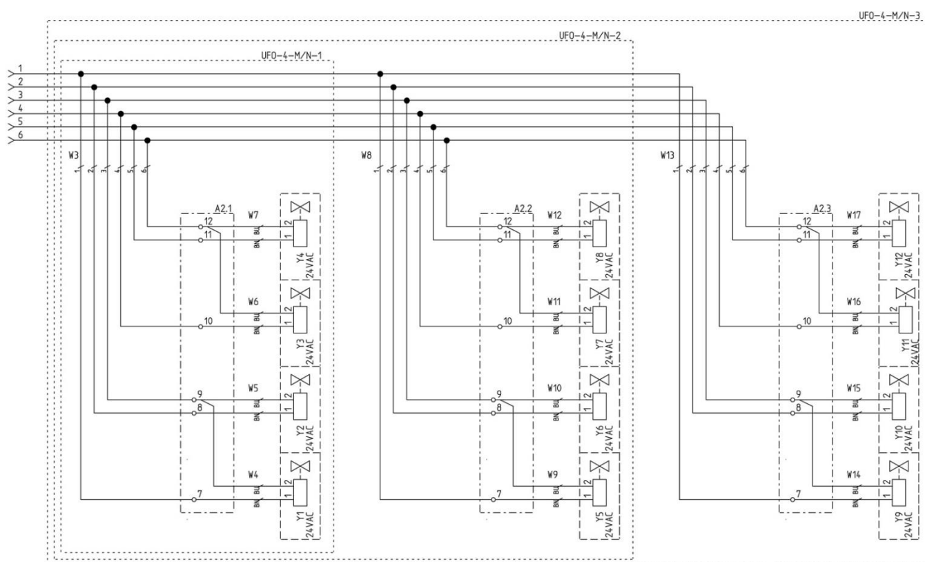
Rys. 5 UFO-4-M/N-3, Podłączenie elektrozaworów
