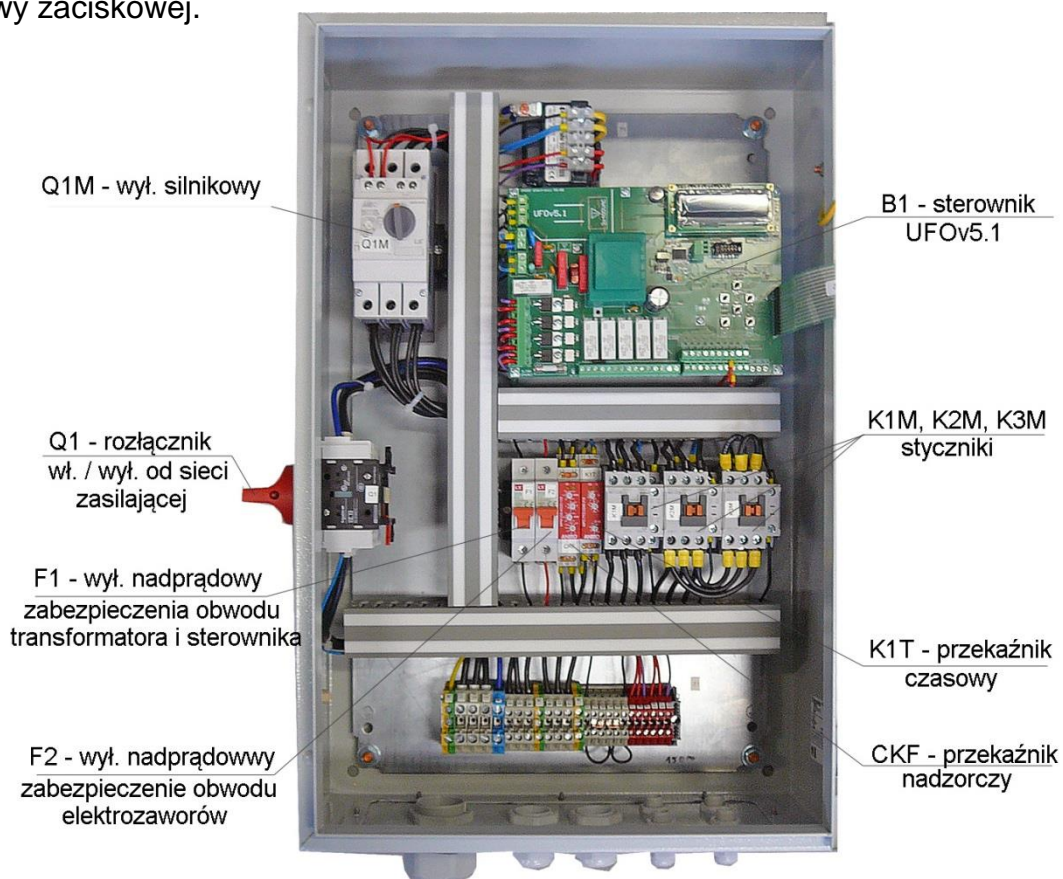
Rys. 8 Zespół elektryczny ZE-UFO-4-M/N-3, wnętrze
