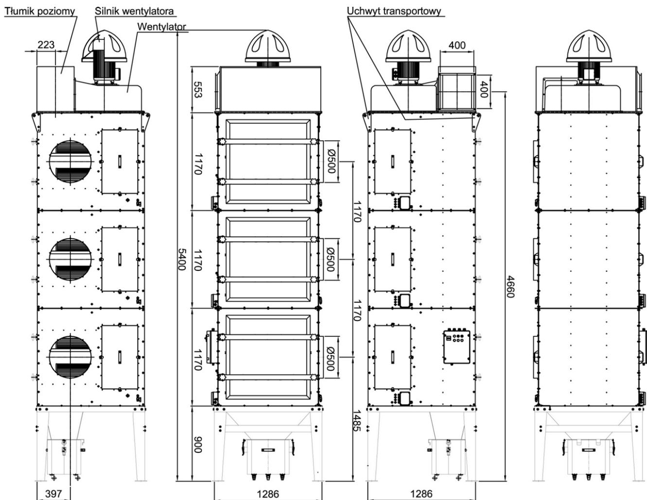
Rys. 1. UFO-4-M/N-3, budowa i wymiary
