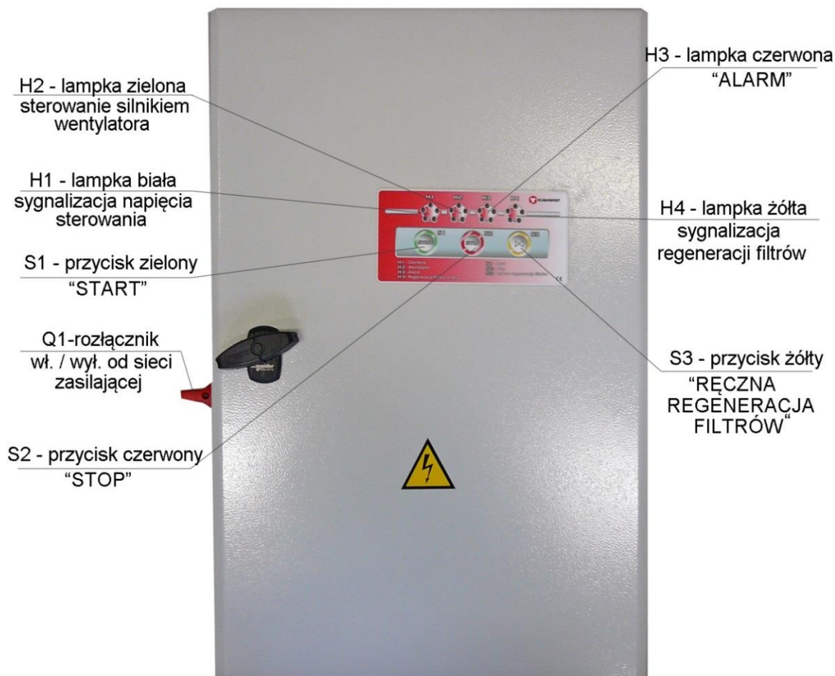
Rys. 6 Zespół elektryczny ZE-UFO-4-MN-3, elewacja
