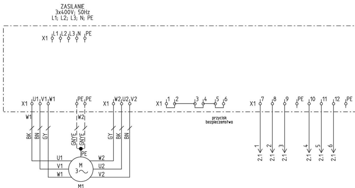
Rys. 4 UFO-4-M/N-3, schemat połączeń elektrycznych
