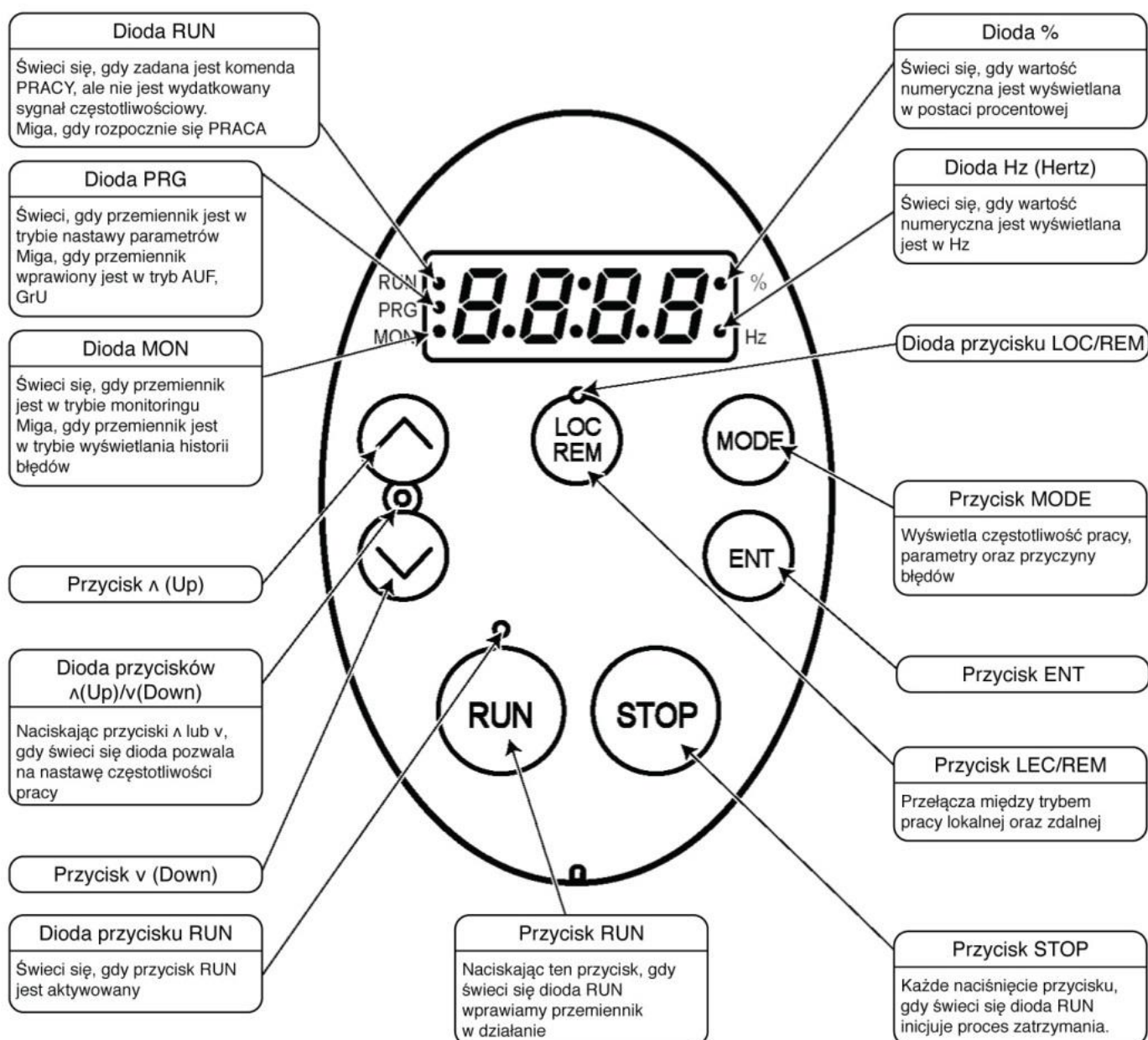
Rys. 10 Opis panelu sterującego przemiennika częstotliwości
