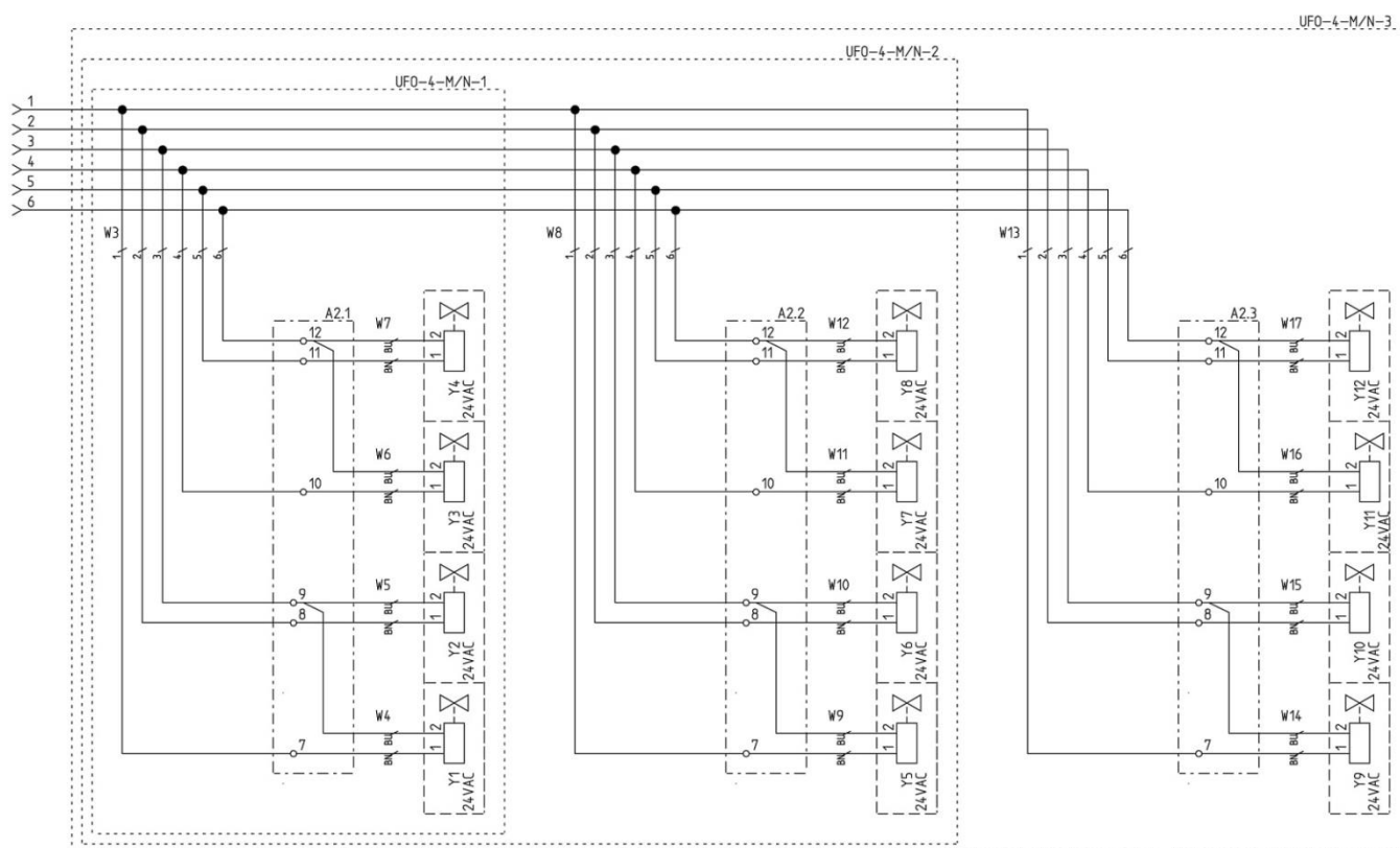
Rys. 5 UFO-4-M/N-2/R, Podłączenie elektrozaworów
