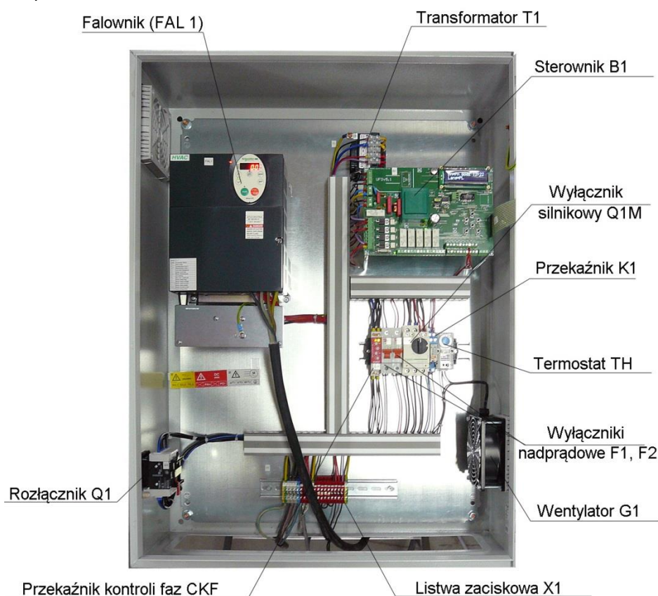
Rys. 8 Zespół elektryczny ZE-UFO-4-M/N-2/R, wnętrze
