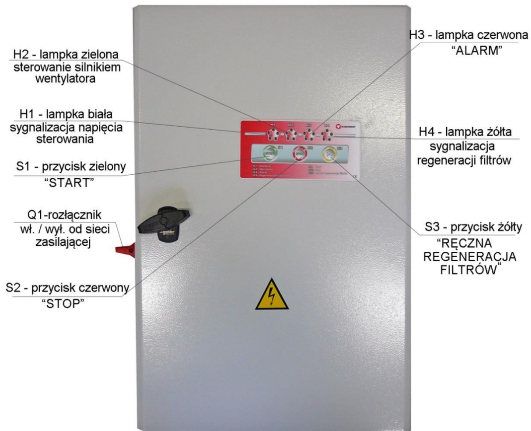
Rys. 6 Zespół elektryczny ZE-UFO-4-MN-1/R, elewacja
