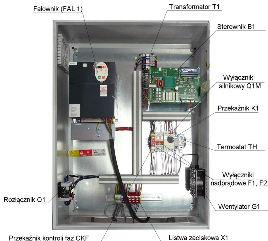
Rys. 8 Zespół elektryczny ZE-UFO-4-M/N-1/R, wnętrze
