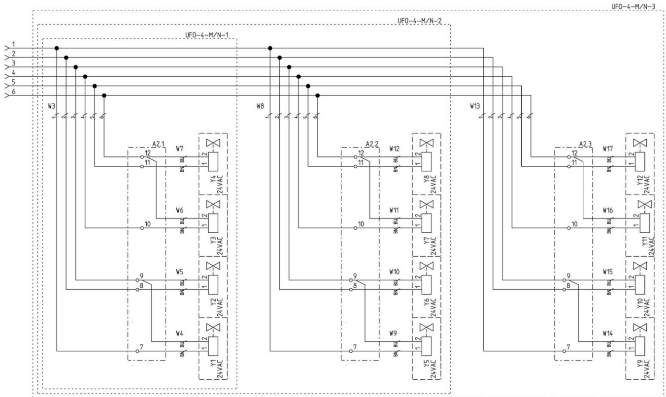
Rys. 5 UFO-4-M/N-1/R, Podłączenie elektrozaworów
