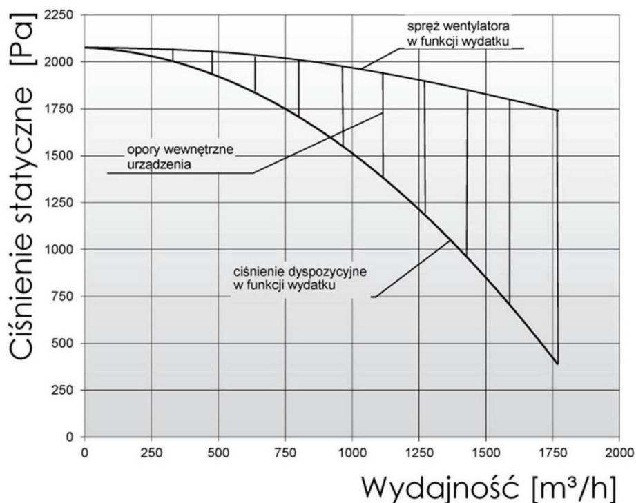
Rys. 1 Charakterystyka przepływowa
