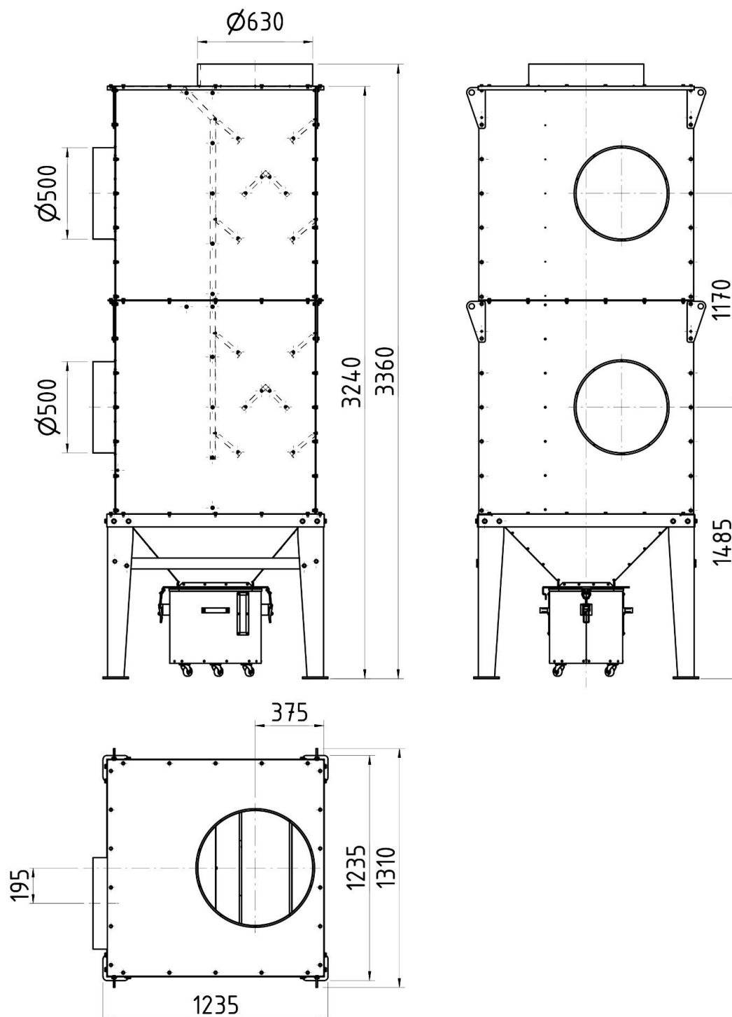
Rys. 2 Budowa i wymiary separatora SEP-UFO-A-20000 – wykonanie prawostronne
