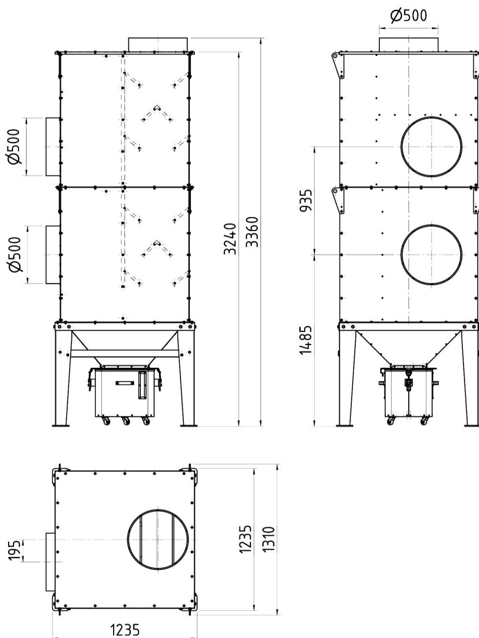
Rys. 1 Budowa i wymiary separatora SEP-UFO-A-20000 – wykonanie lewostronne
