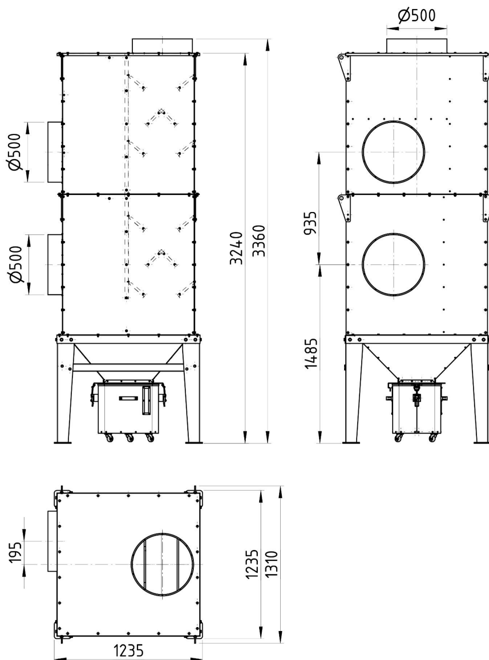
Rys. 1 Budowa i wymiary separatora SEP-UFO-A-15000 – wykonanie lewostronne
