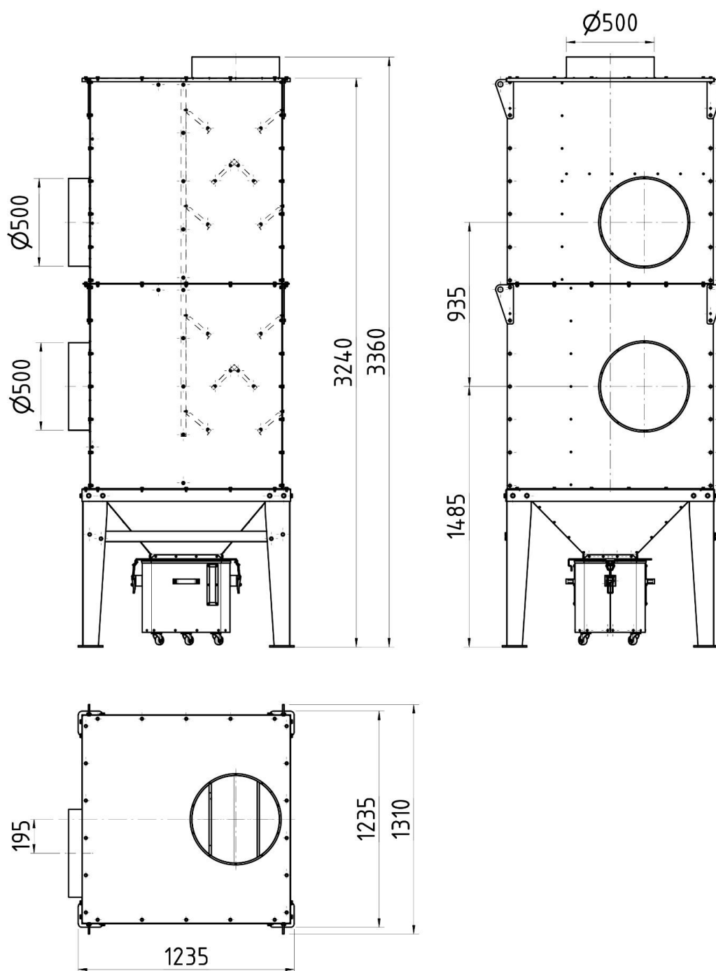
Rys. 2 Budowa i wymiary separatora SEP-UFO-A-15000 – wykonanie prawostronne
