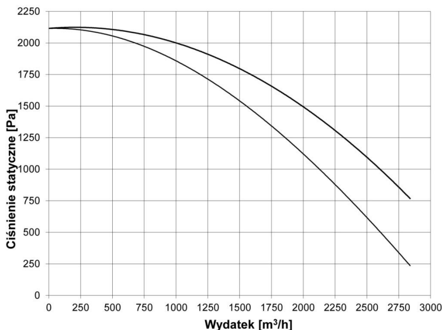
Rys. 1 Charakterystyka przepływowa urządzenia typu MISTOL MIX-2000
