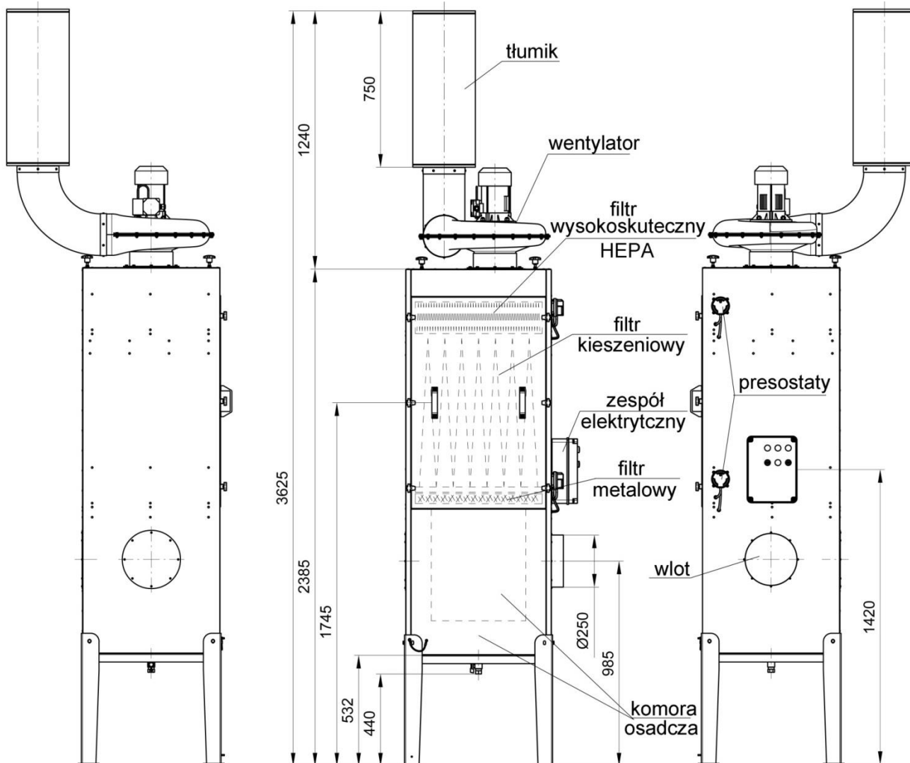
Rys. 2 Budowa i wymiary urządzenia typu MISTOL-2000
