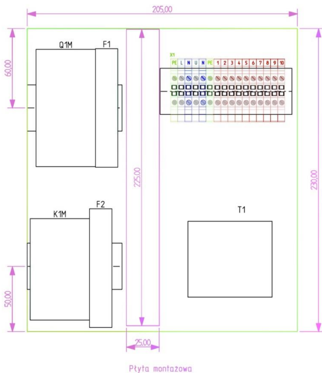
Rys. 4 Zespół elektryczny urządzenia typu MISTOL MIX-2000
