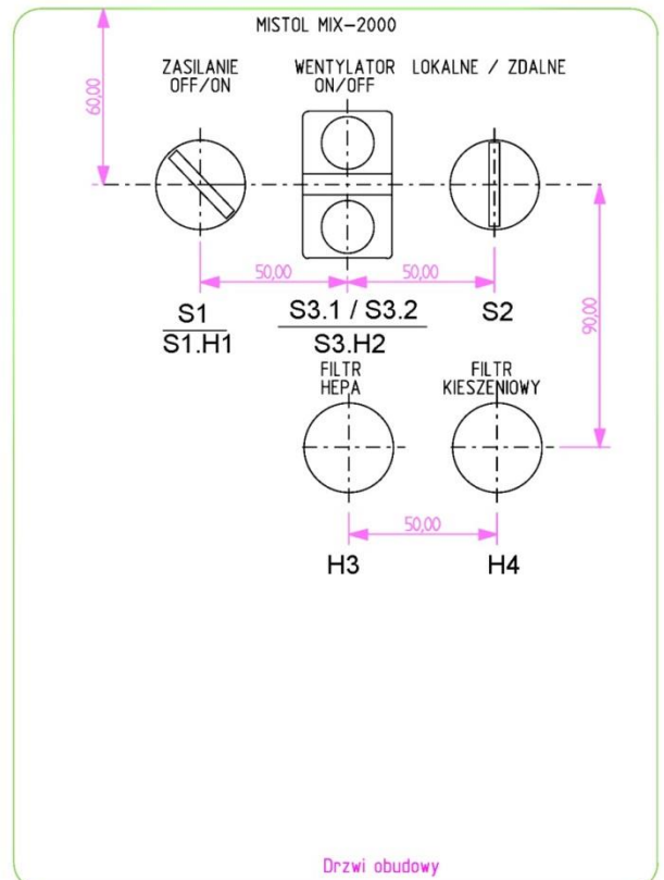
Rys. 4 Zespół elektryczny urządzenia typu MISTOL MIX-2000
