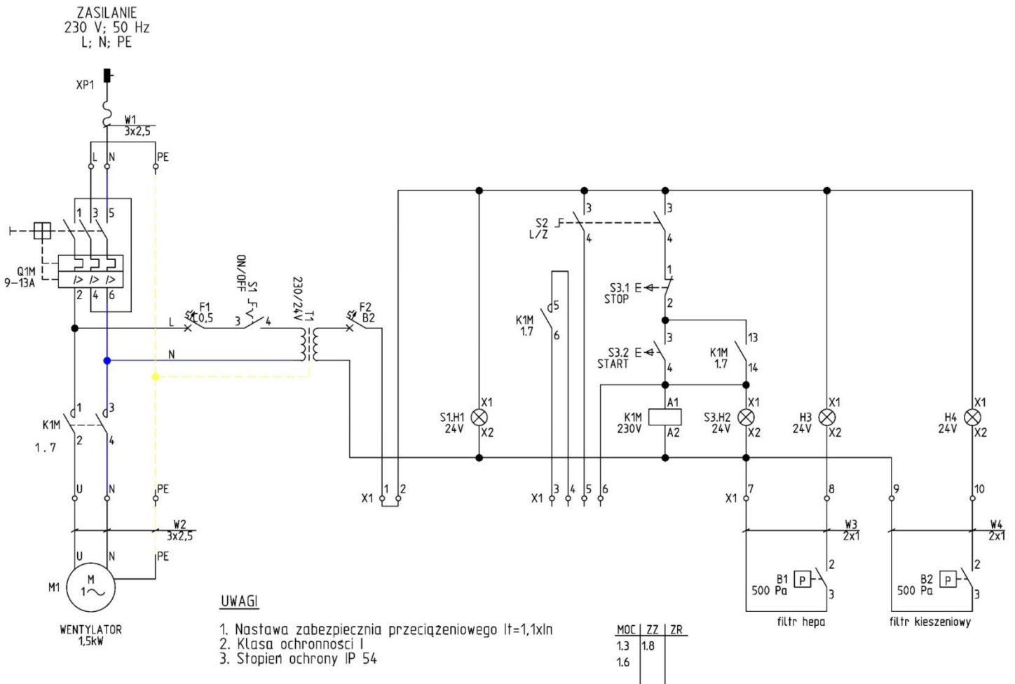
Rys. 3 Schemat elektryczny urządzenia typu MISTOL MIX-2000
