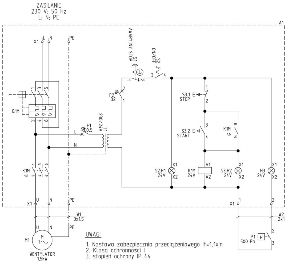
Rys. 3 Schemat elektryczny urządzenia typu MISTOL DUST-2000
