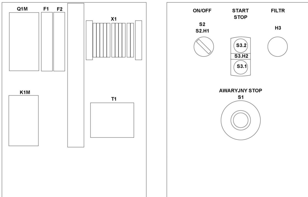
Rys. 4 Zespół elektryczny urządzenia typu MISTOL DUST-2000
