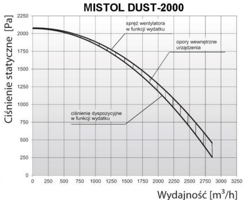
Rys. 1 Charakterystyka przepływowa urządzenia typu MISTOL DUST-2000
