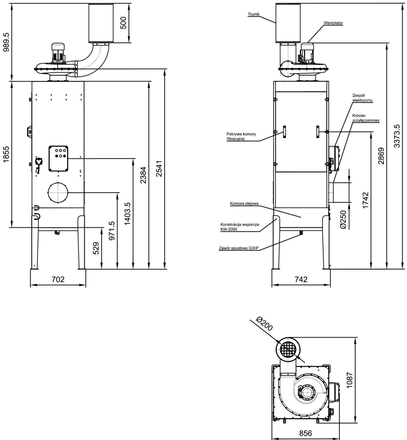
Rys. 2 Budowa i wymiary urządzenia typu MISTOL DUST-2000
