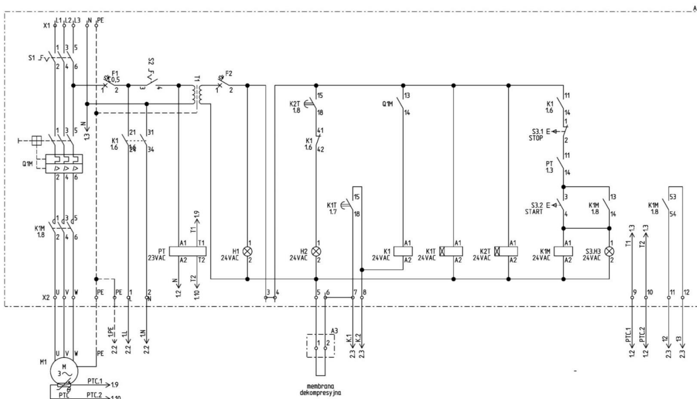
Rys. 7 Schemat ideowy Rozdzielnicy A1
