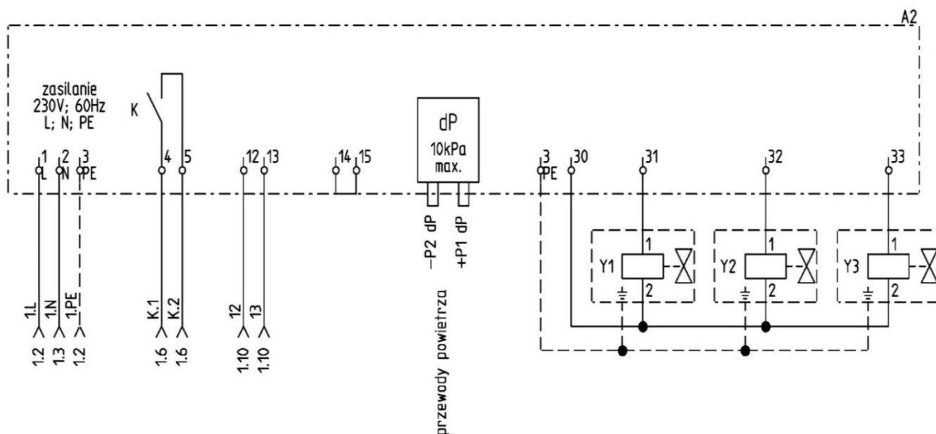
Rys. 8. Schemat ideowy Mikrokontrolera A2
