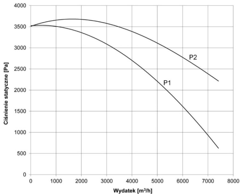
Rys. 1. Charakterystyka przepływowa urządzenia BIG-5000/Ex
