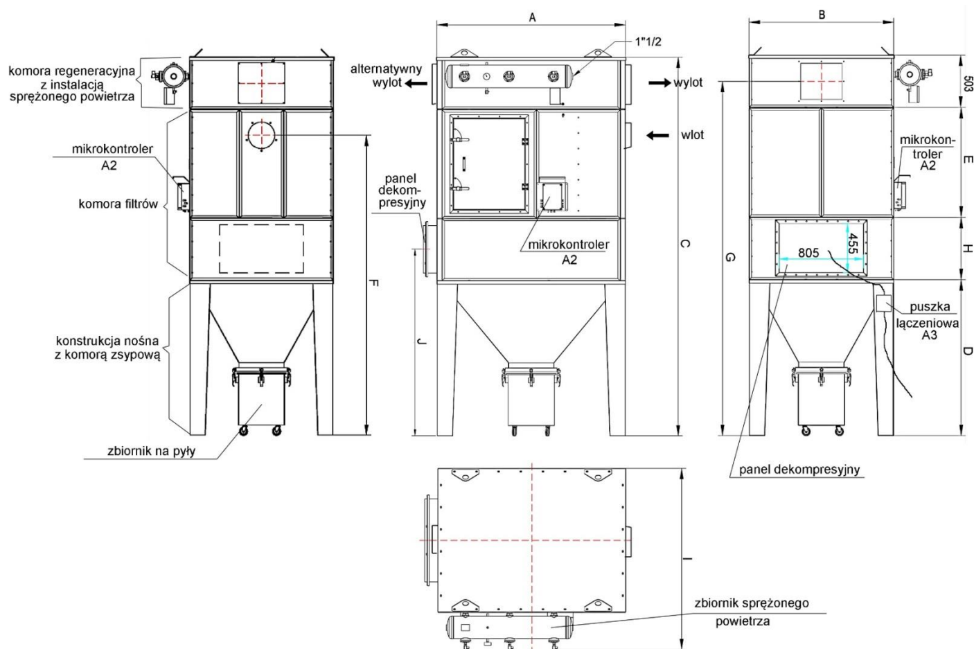
Rys. 4. Budowa i wymiary urządzenia typu BIG-5000/Ex
