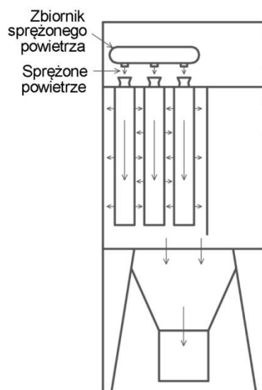
Rys. 4 Schemat regeneracji filtrów
