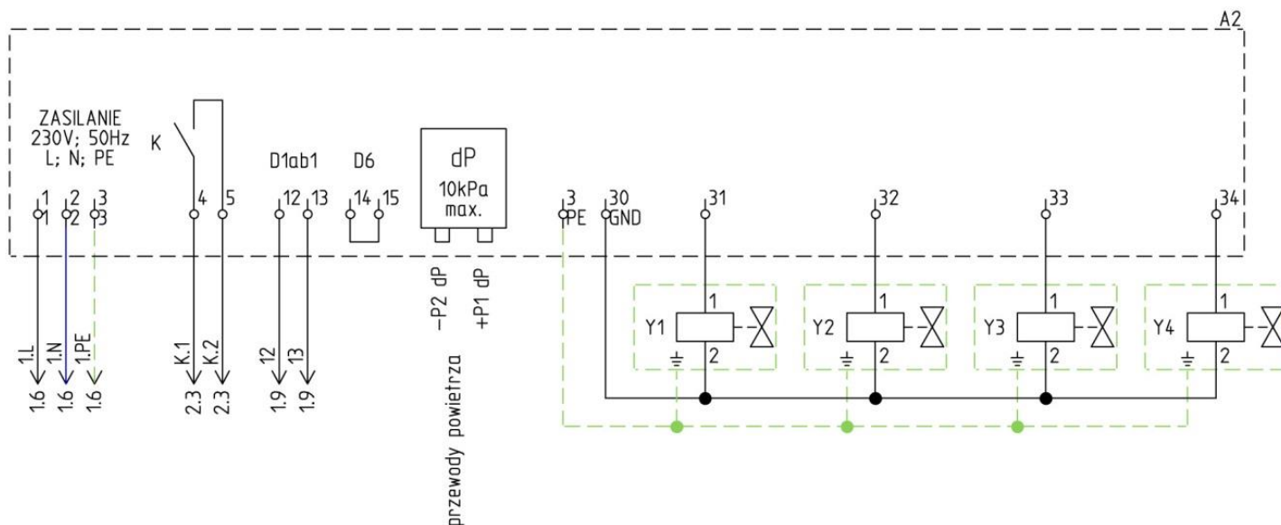
Rys. 8 Schemat elektryczny nr 3/3
