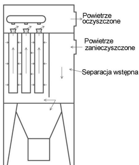
Rys. 3 Schemat filtrowania
