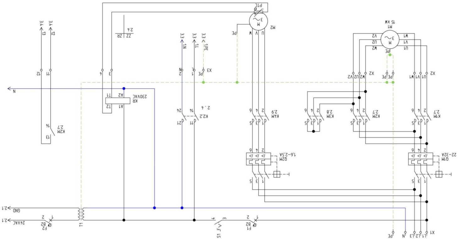
Rys. 6 Schemat elektryczny nr 1/3
