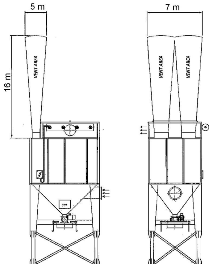
Rys. 5 Panel dekompresyjny – strefa zagrożenia
