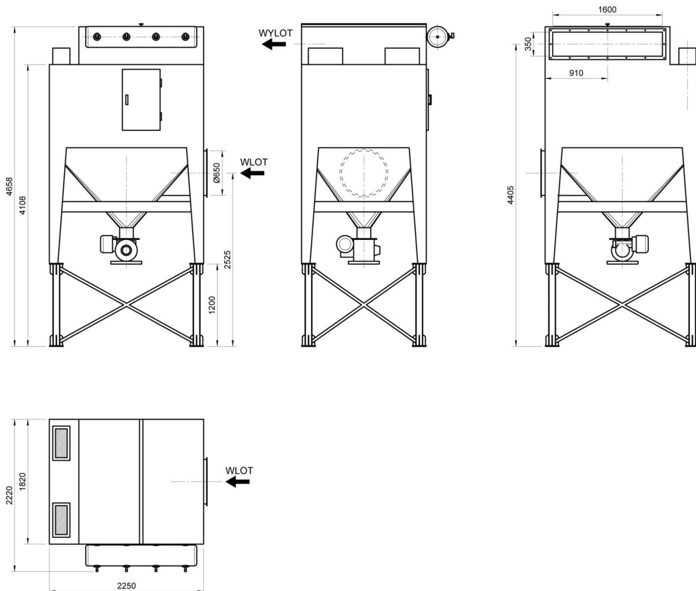
Rys. 2 Budowa i wymiary urządzenia typu BIG-12000/Ex
