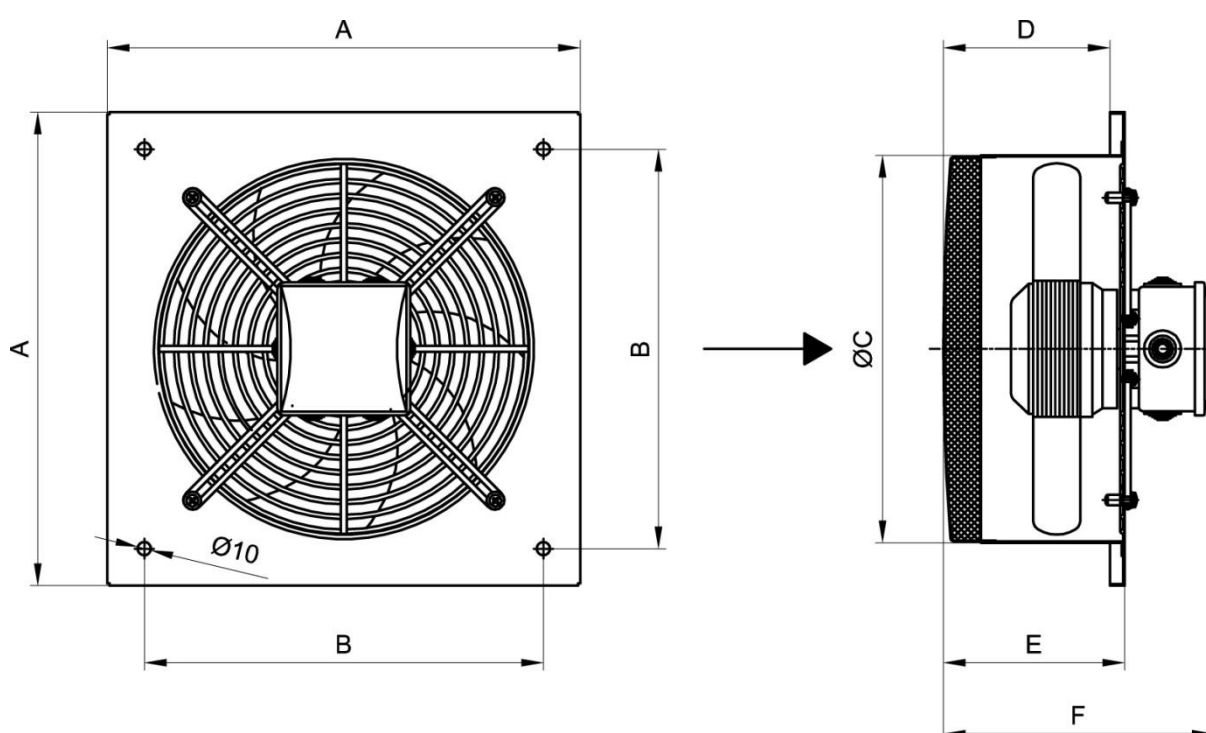
Rys. 1 Budowa i wymiary wentylatorów typu WOK-N
