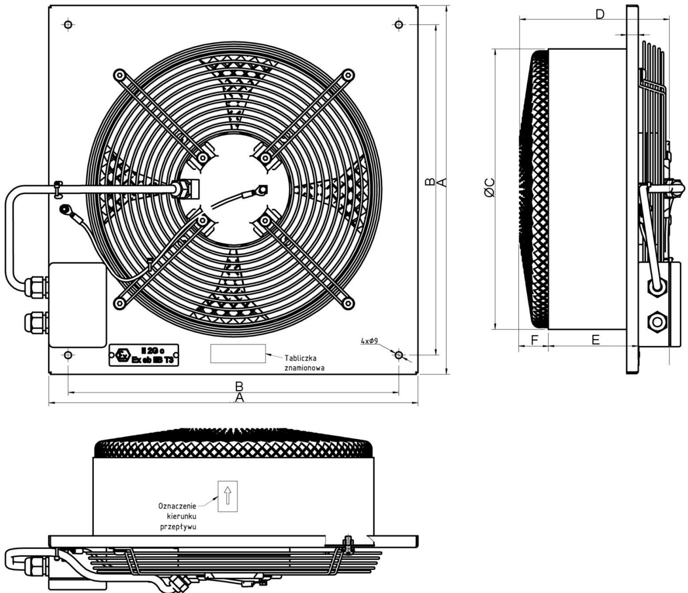
Rys. 2. Budowa i wymiary wentylatorów typu WOK/Ex
