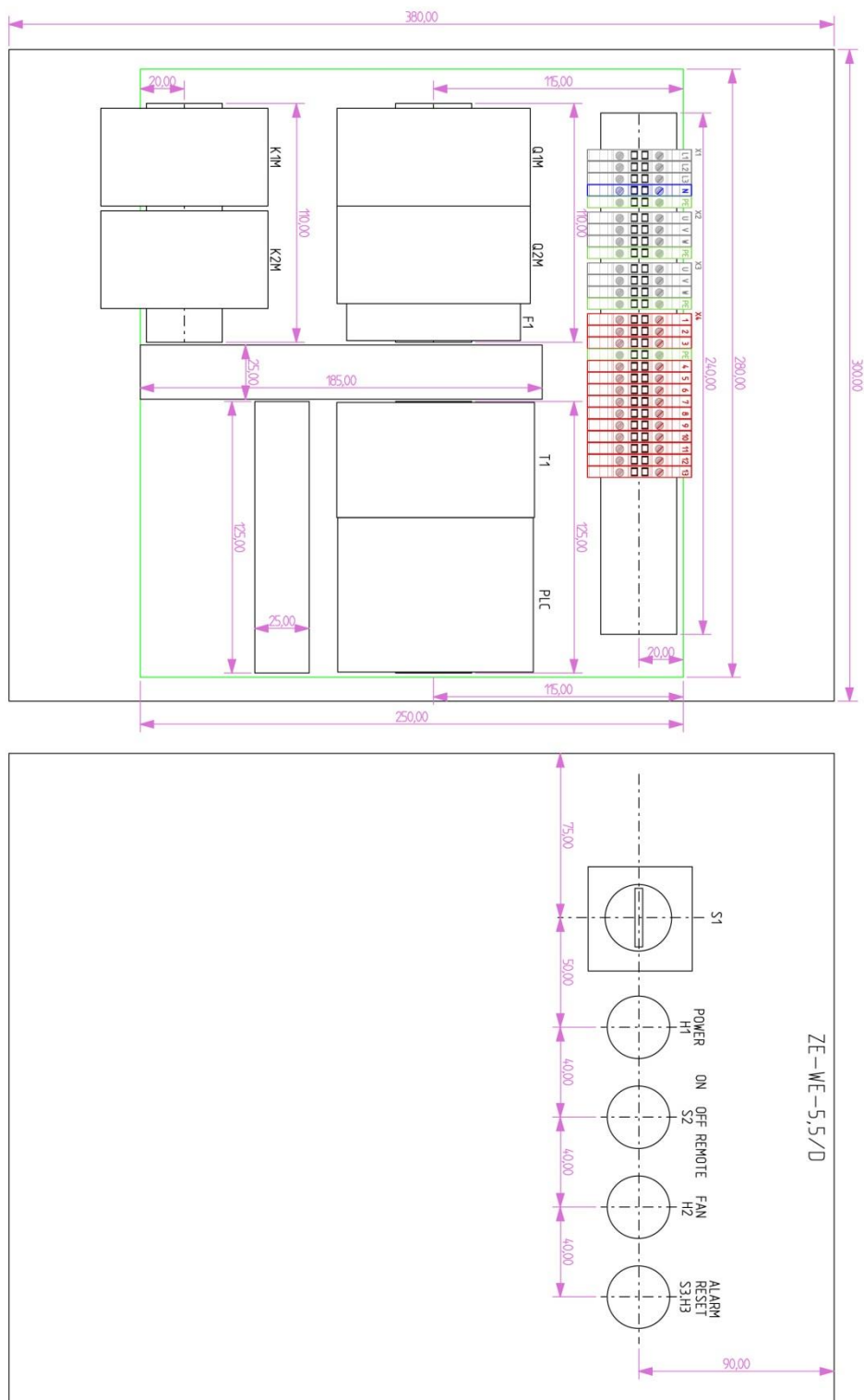
Rys. 8 Zabudowa aparatury
