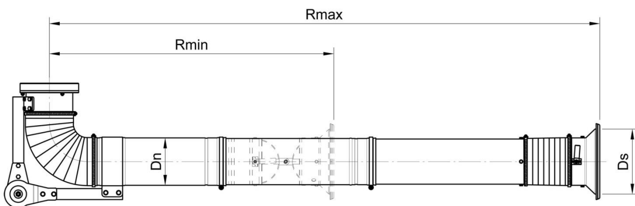
Rys. 1 TELERGO-L-3-2000, rysunek wymiarowy
