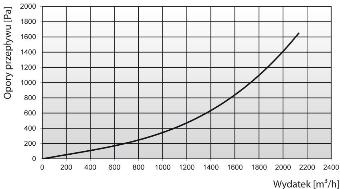
Rys. 3 Charakterystyka przepływowa
