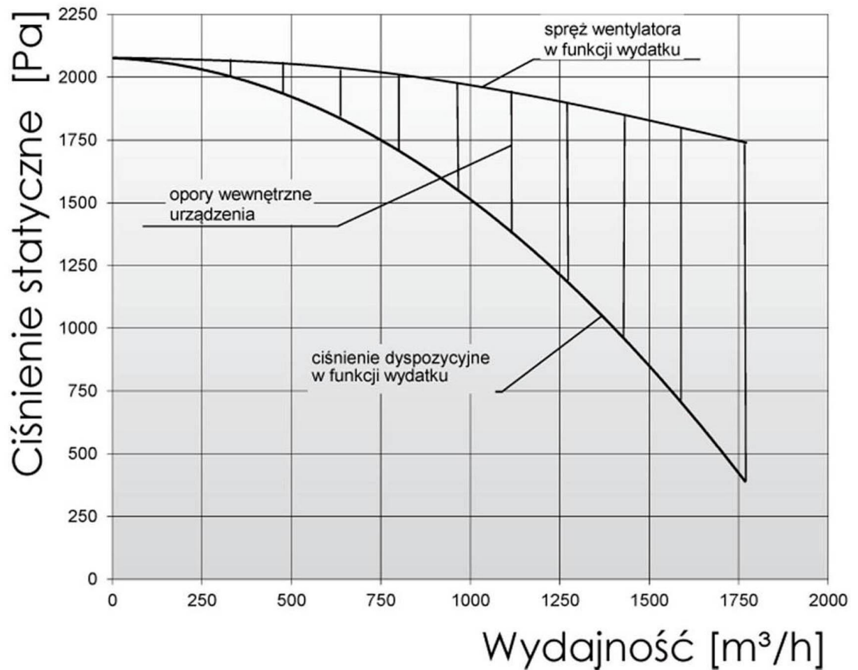
Rys. 1 Charakterystyka przepływowa
