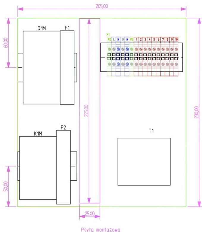
Rys. 4 Zespół elektryczny urządzenia typu MISTOL MIX-2000
