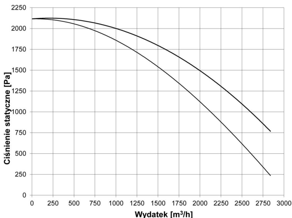
Rys. 1 Charakterystyka przepływowa urządzenia typu MISTOL MIX-2000
