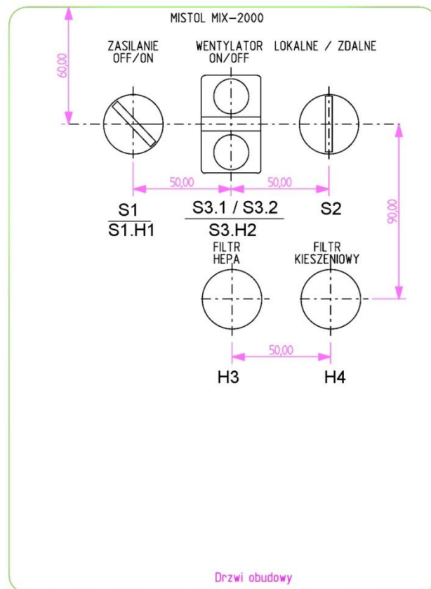
Rys. 4 Zespół elektryczny urządzenia typu MISTOL MIX-2000
