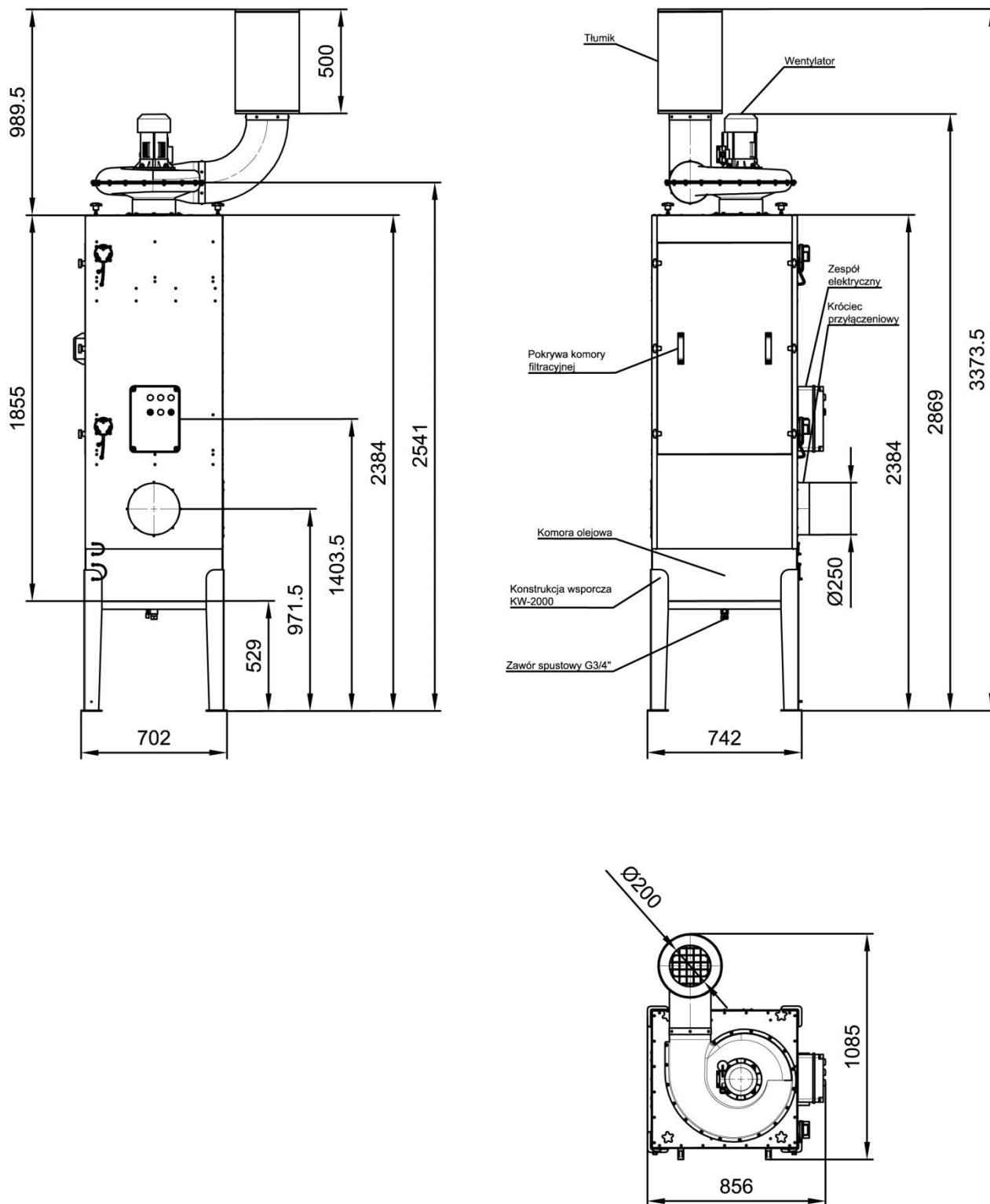
Rys. 2 Budowa i wymiary urządzenia typu MISTOL MIX-2000
