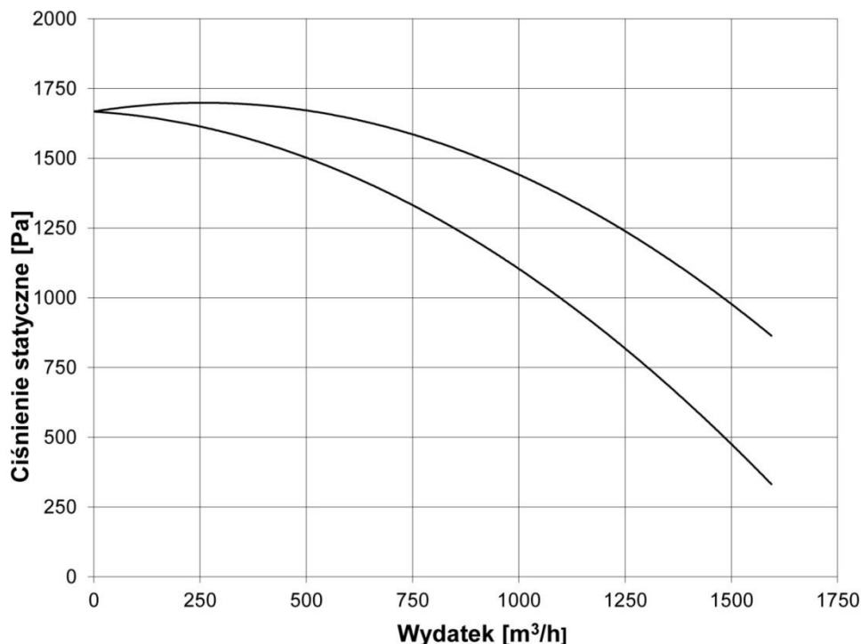
Rys. 1 Charakterystyka przepływowa urządzenia typu MISTOL MIX-1000
