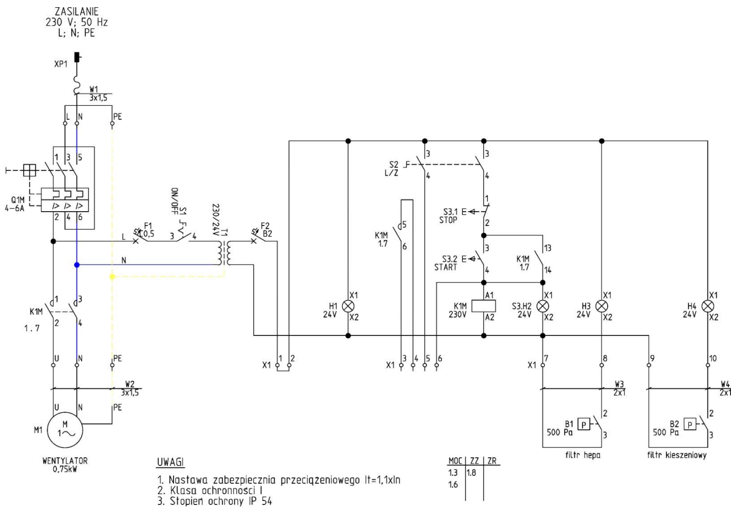
Rys. 3 Schemat elektryczny urządzenia typu MISTOL MIX-1000
