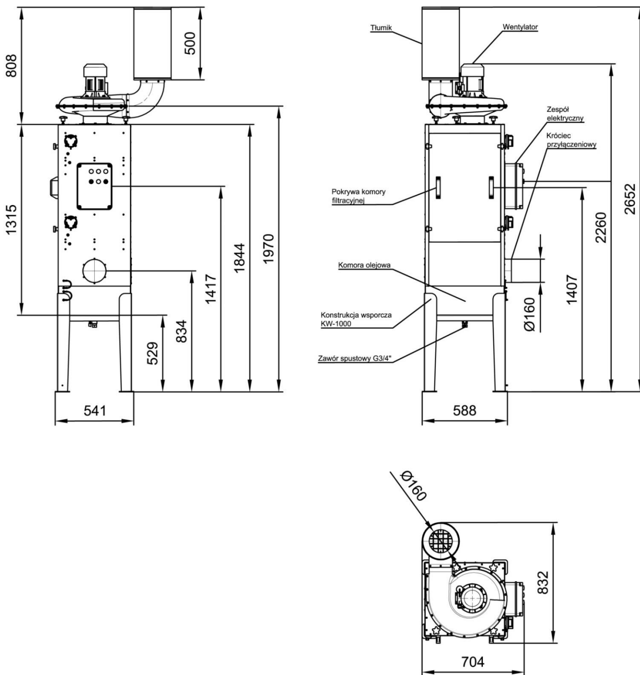
Rys. 2 Budowa i wymiary urządzenia typu MISTOL MIX-1000
