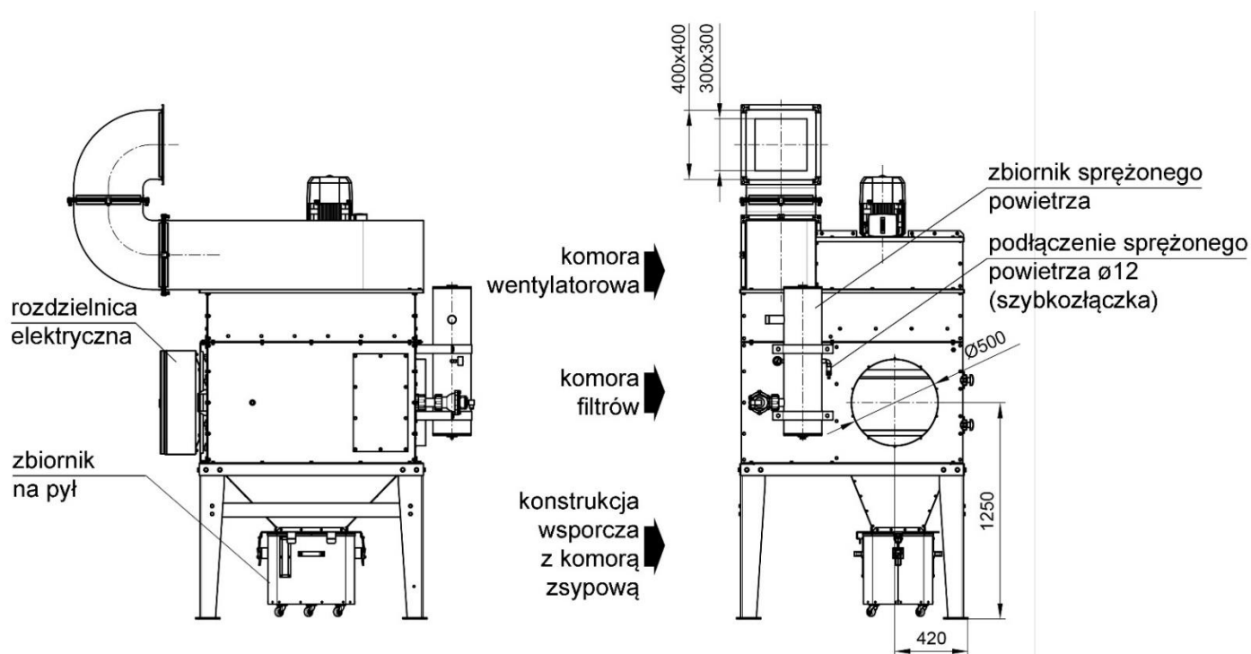
Rys. 3 UFO-A-5000/R RH i LH, budowa i wymiary.
