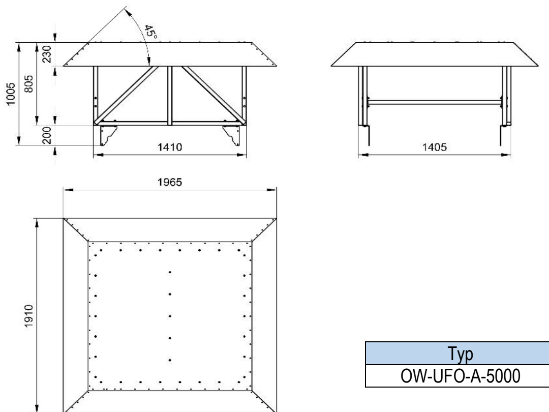
Rys. 1 Element dodatkowy – osłona wentylatora montowana na urządzeniu
