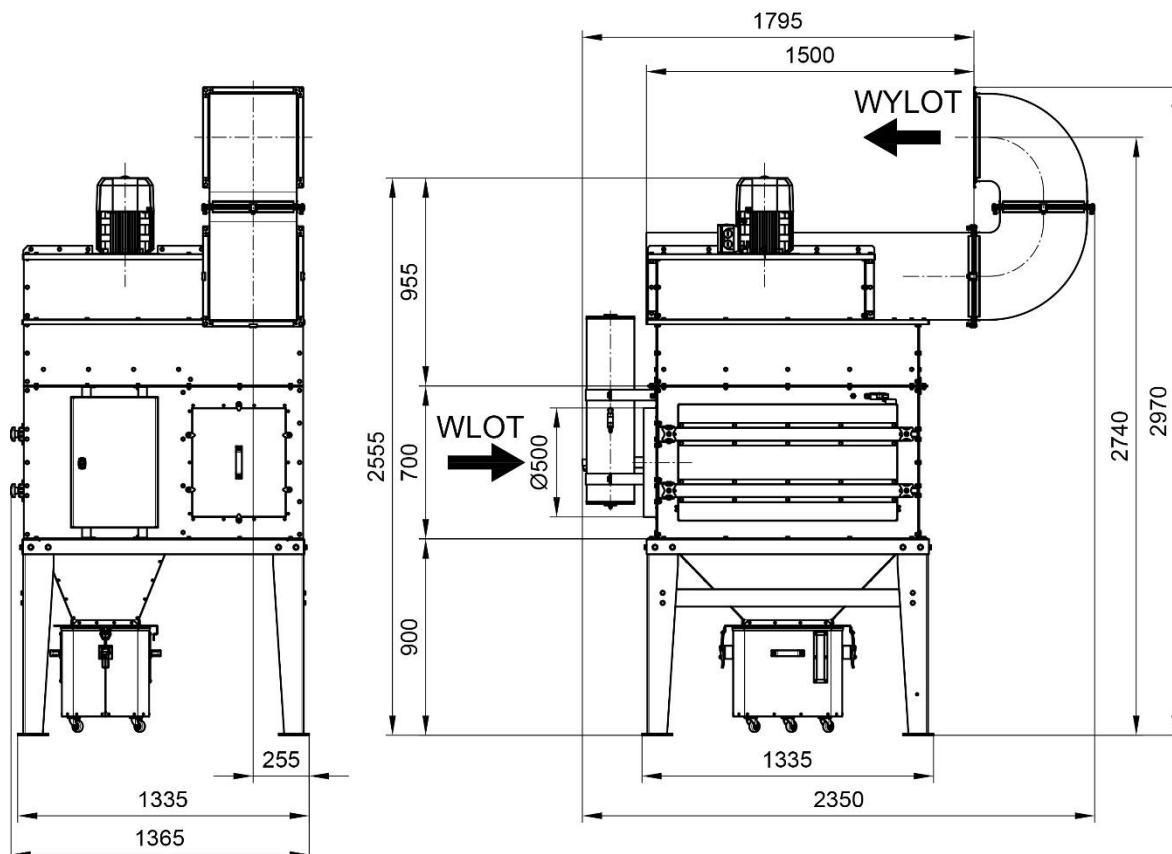
Rys. 2b UFO-A-5000/R LH (z wlotem powietrza z lewej strony) - wymiary
