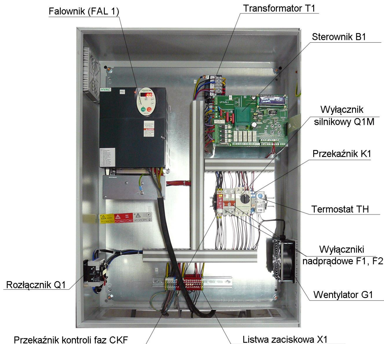
Rys. 7 Rozdzielnica elektryczna ZE-UFO-A – wnętrze
