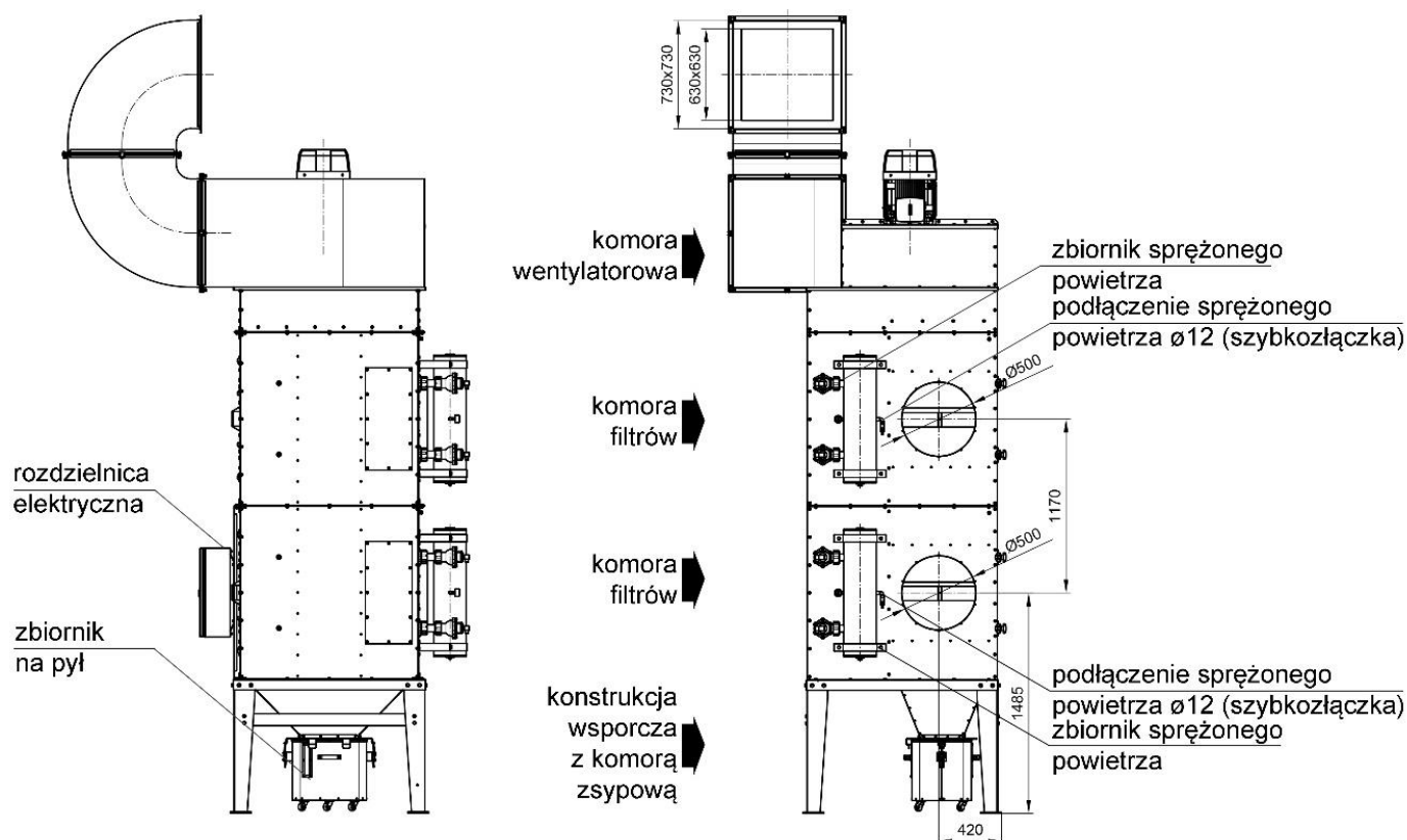
Rys. 3 UFO-A-2000, budowa i wymiary
