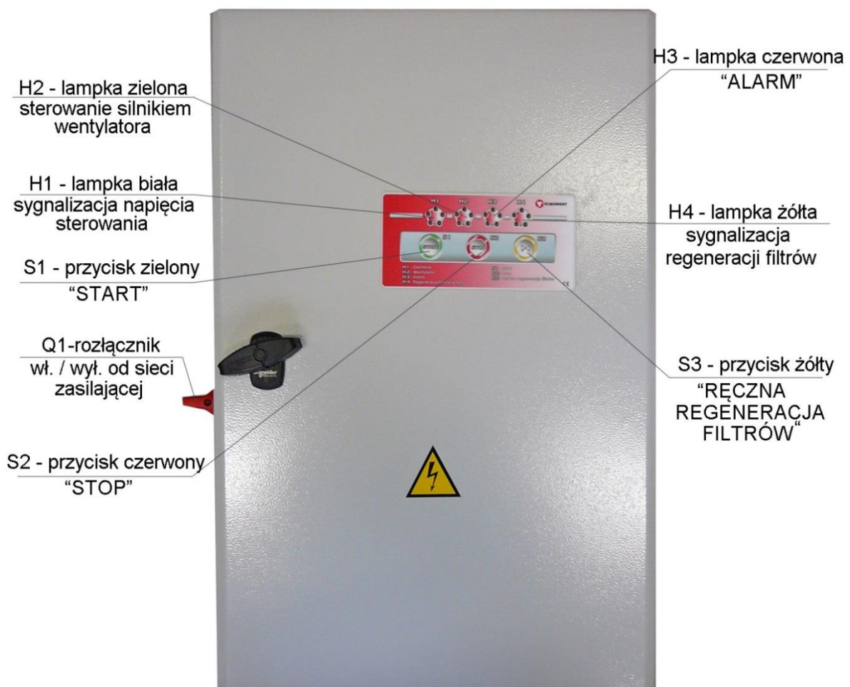
Rys.5 Rozdzielnica elektryczna – elewacja
