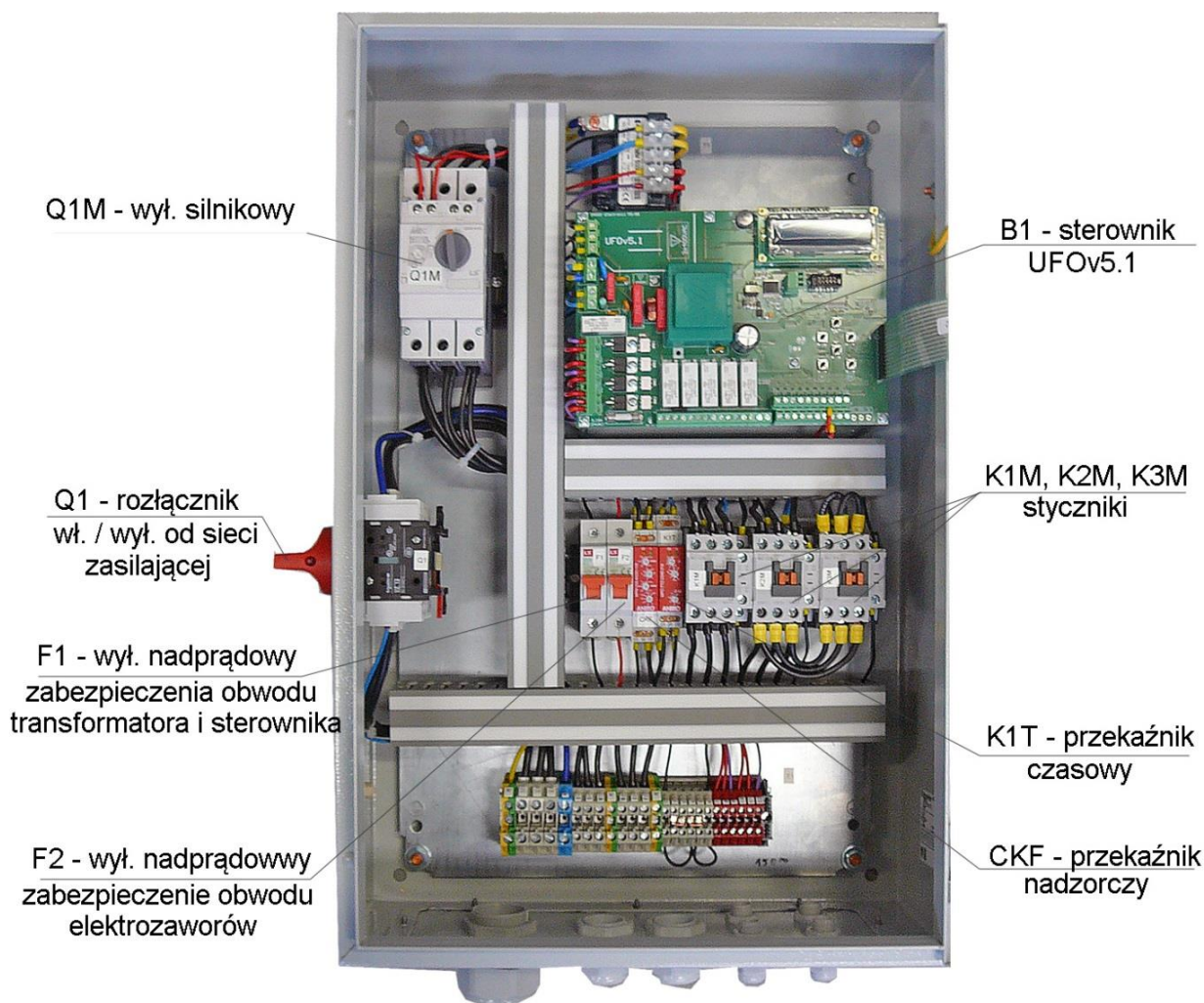
Rys.7 Rozdzielnica elektryczna ZE-UFO-A – wnętrze
