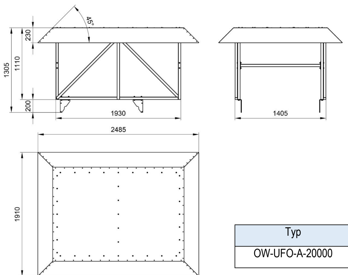
Rys.1 Element dodatkowy – osłona wentylatora montowana na urządzeniu
