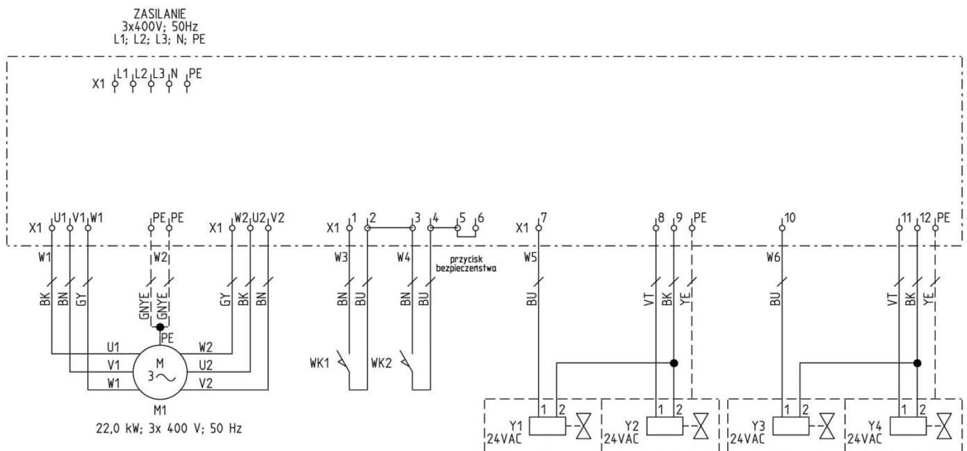
Rys. 4 UFO-A-20000, schemat połączeń elektrycznych
