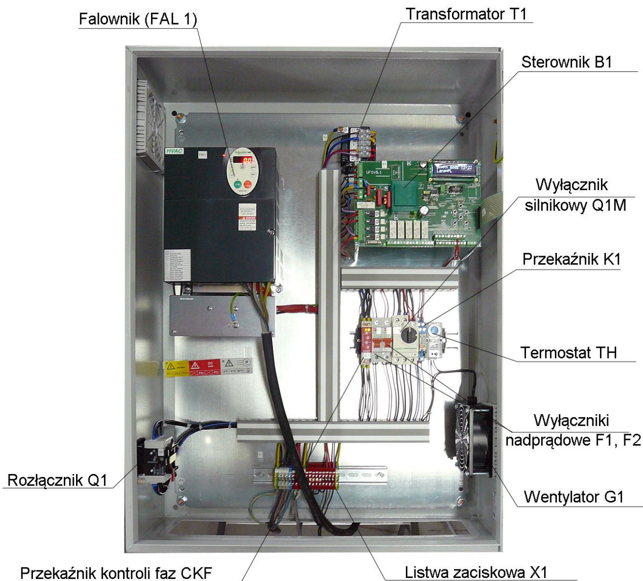
Rys. 7 Rozdzielnica elektryczna ZE-UFO-A-15000/R
