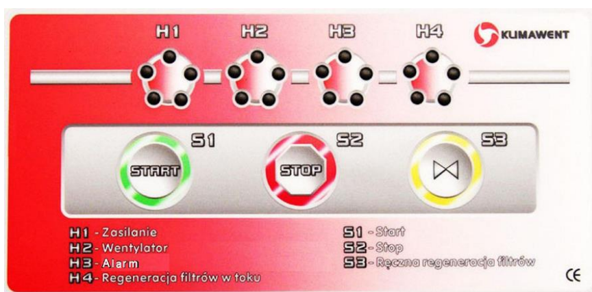
Rys. 6 Panel sterowniczy
