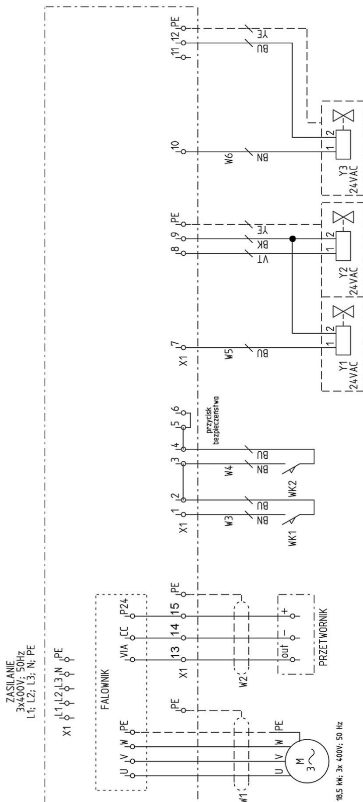
Rys. 4 UFO- A-15000/R, schemat połączeń elektrycznych
