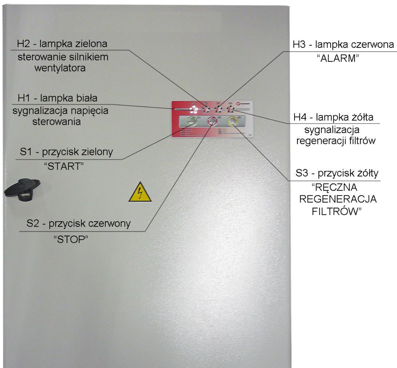
Rys. 5 Rozdzielnica elektryczna – elewacja
