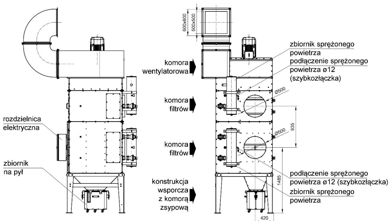
Rys. 3 UFO-A-15000/R, budowa i wymiary
